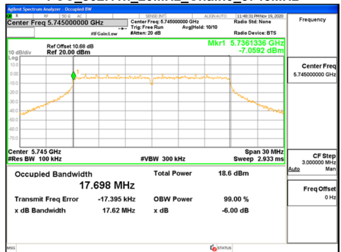
FCC_802.11n_20MHz_Chain0_5745MHz
