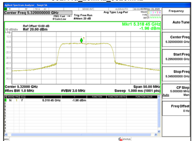
802.11a_20MHz_5320MHz
