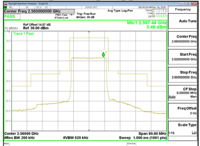
Band7_20MHz\QPSK_RB100_0_CH21350
