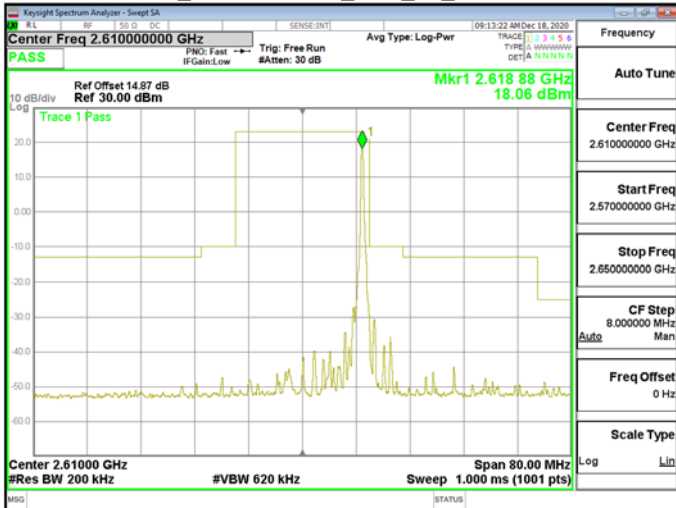
Band38_20MHz\QPSK_RB1_99_CH38150
