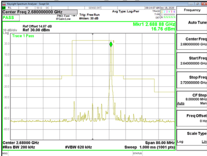
Band41_20MHzQPSK_RB1_99_CH41490
