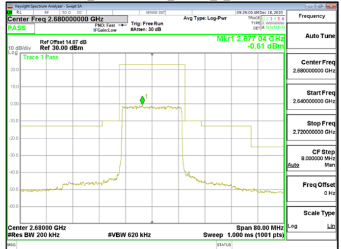
Band41_20MHzQPSK_RB100_0_CH41490
