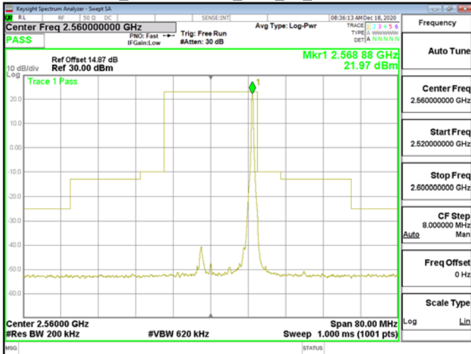
Band7_20MHz\QPSK_RB1_99_CH21350
