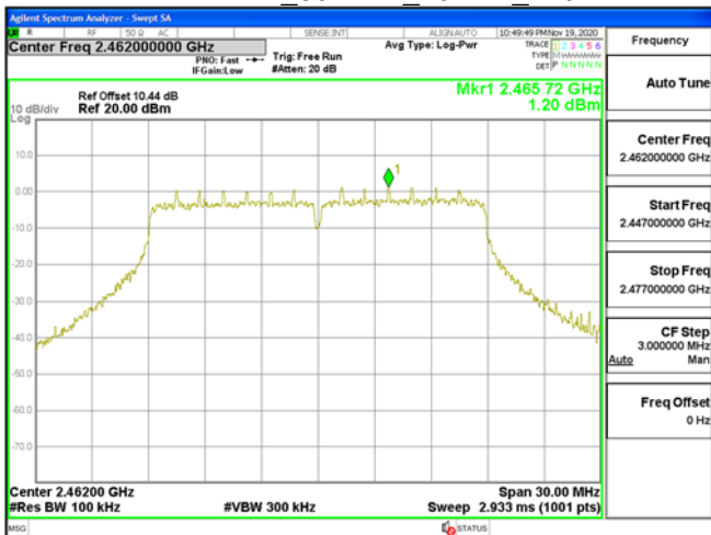
Reference Level 802.11n 20MHz 2462MHz
