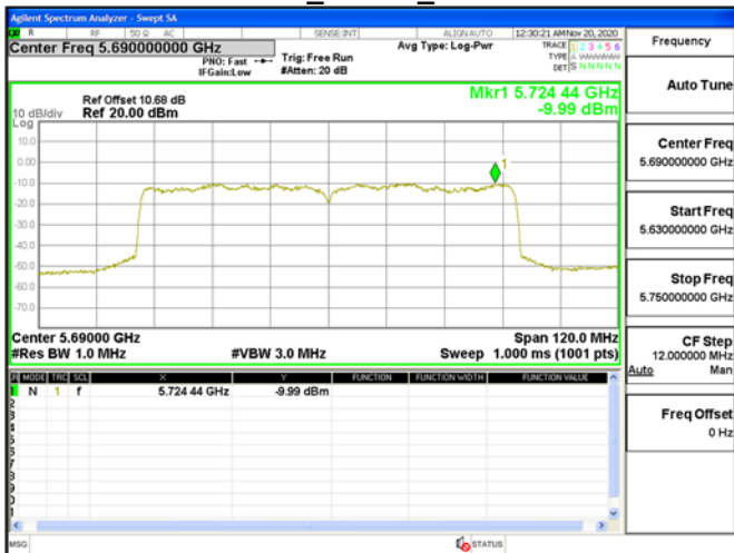
802.11ac_80MHz_5690MHz
