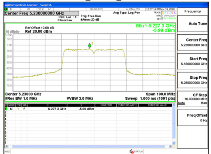
802.11n_40MHz_5230MHz
