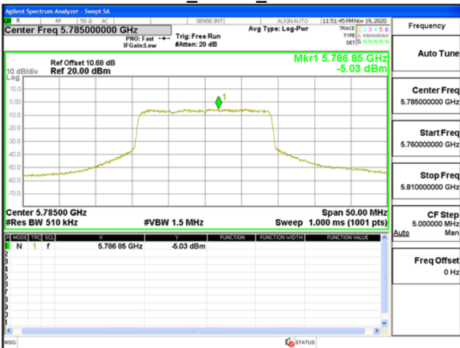
802.11n_20MHz_5785MHz
