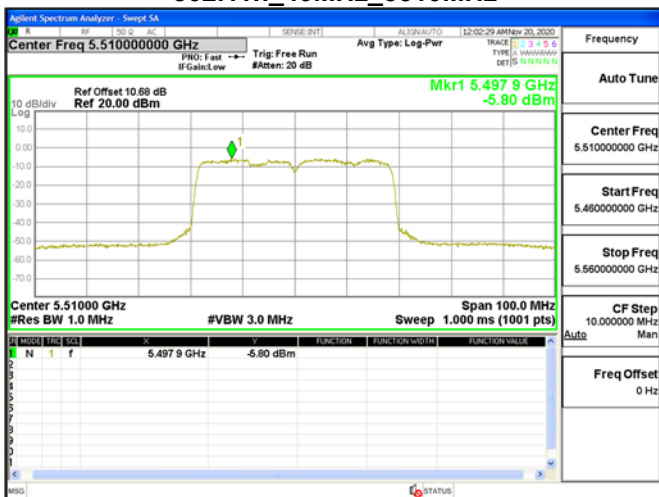
802.11n_40MHz_5510MHz
