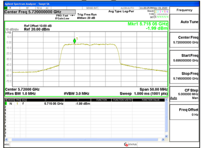
802.11a_20MHz\5720MHz
