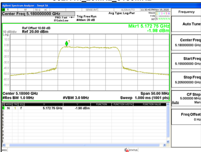
802.11n_20MHz_5180MHz
