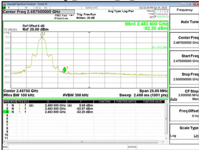
Hopping Band Edge \pi/4 DQPSK_2M_2480MHz
