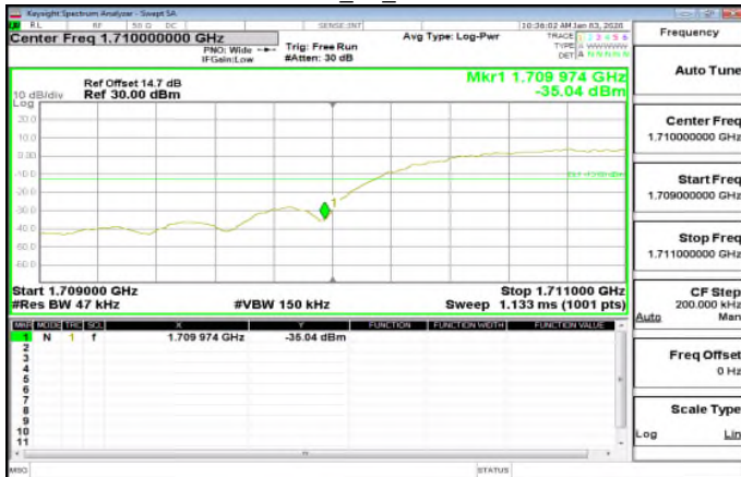
WCDMA\WCDMA_B4_LowCH1312-1712.4
