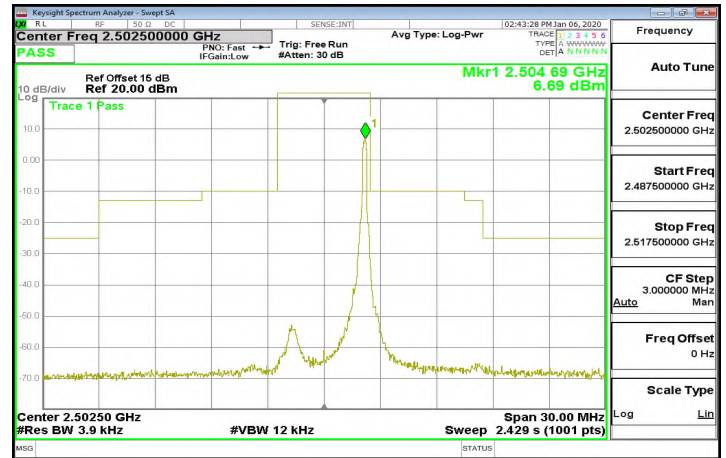
Band7_5MHz_QPSK_1_24_CH21100
