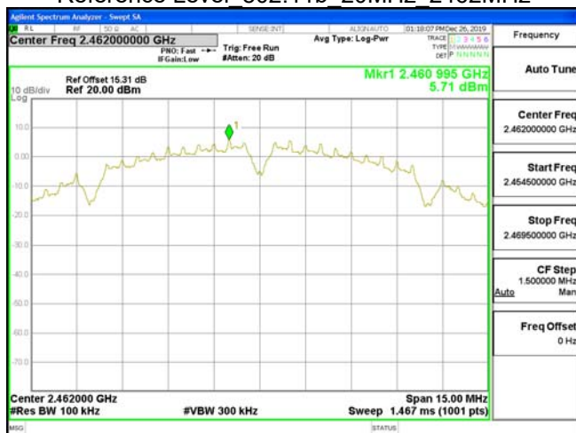
Reference Level 802.11b 20MHz 2462MHz
