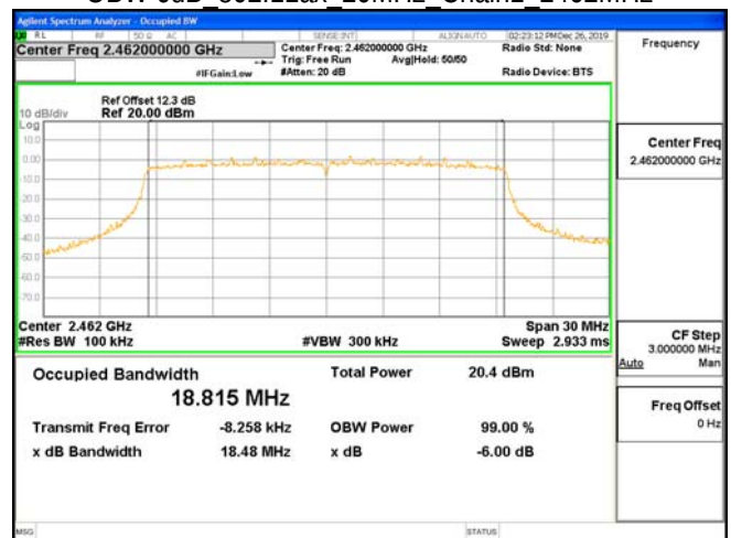
OBW 6dB 802.11ax 20MHz Chain1 2462MHz
