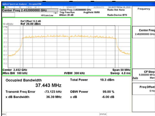
OBW 6dB 802.11ax 40MHz Chain0 2452MHz
