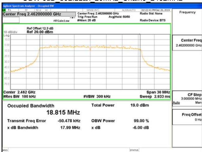
OBW 6dB 802.11ax 20MHz Chain0 2462MHz
