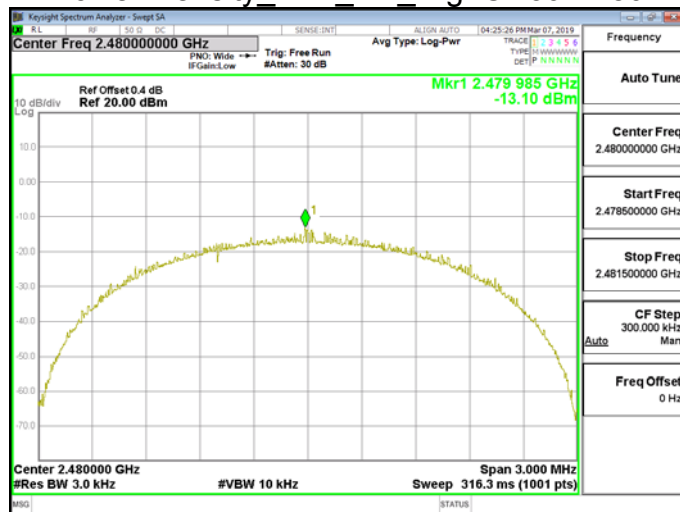
Power Density BLE 2M HighCH39-2480
