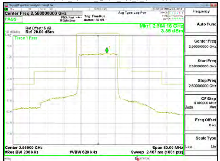
Band7_20MHz_QPSK_100_0_CH21350
