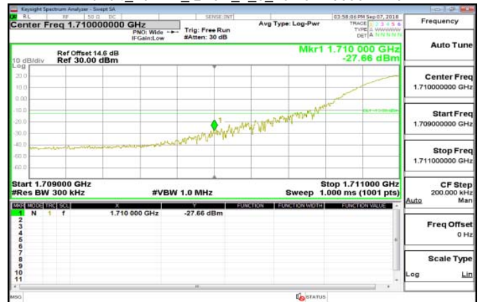
Band4_20MHz_QPSK_1_0_LowCH20050-1720
