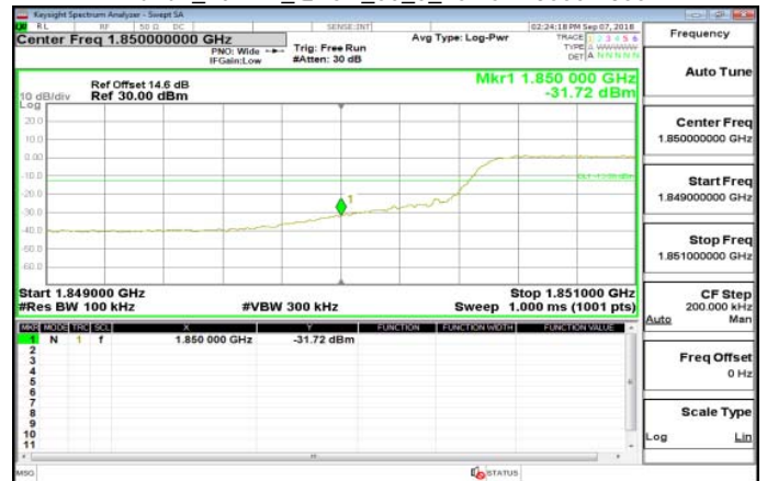
Band2_10MHz_QPSK_50_0_LowCH18650-1855
