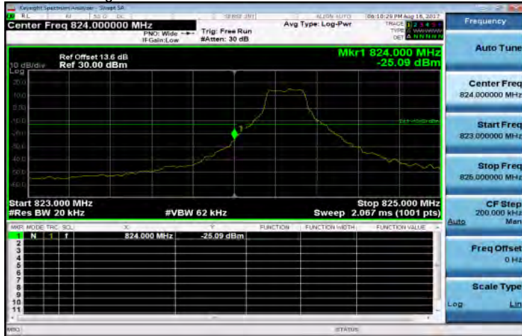
Band Edge_Band5 1.4MHz_QPSK 1 0_LowCH20407-824.7
