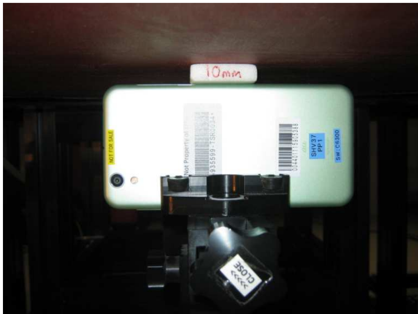
SAR - Right Edge (Body)
