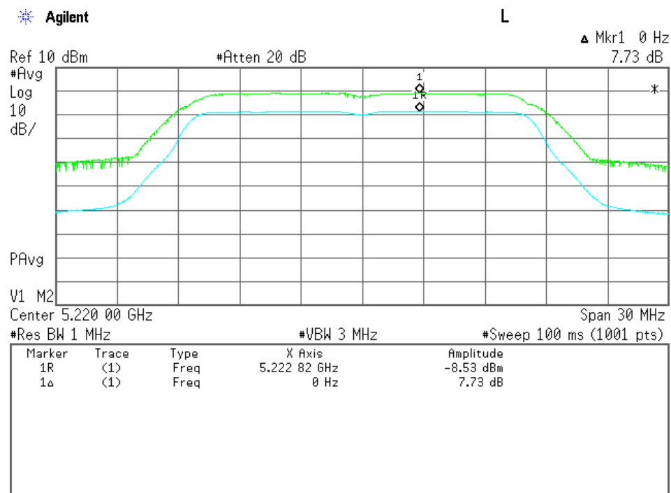
802.11a 44ch (5220 MHz)
