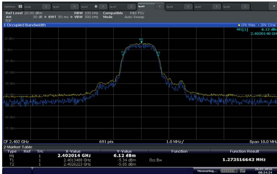
\pi/4 -DQPSK Low Channel
