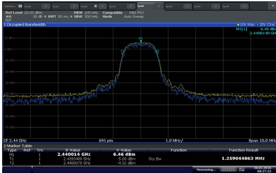
\pi/4 -DQPSK Mid Channel
