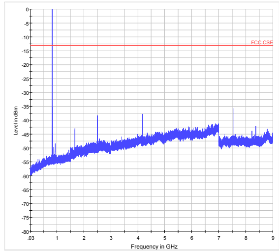
GSM 850 CH-Middle 30MHz~9GHz
