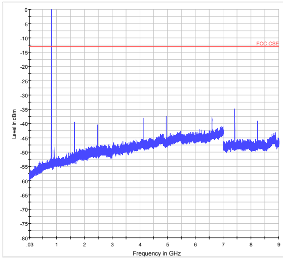
GSM 850 CH-High 30MHz~9GHz
