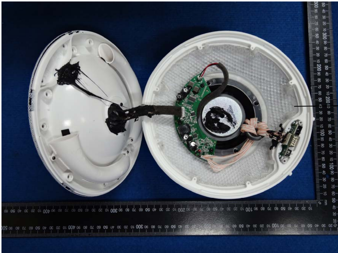
Subwoofer unit
