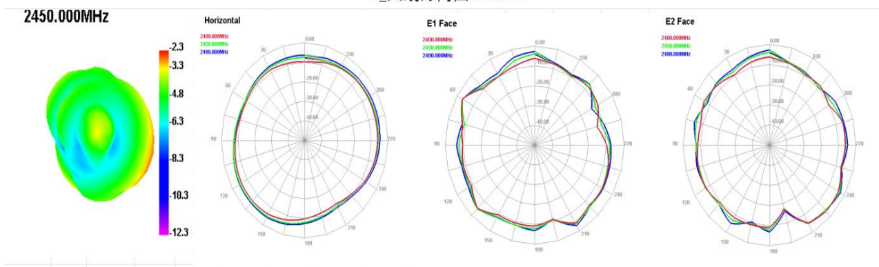
R_天线方向图 2D/3D
