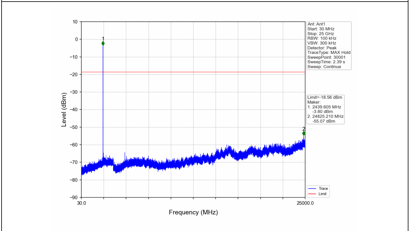
2M_MCH_2440MHz_DataRate=_Ant1_NTNV
