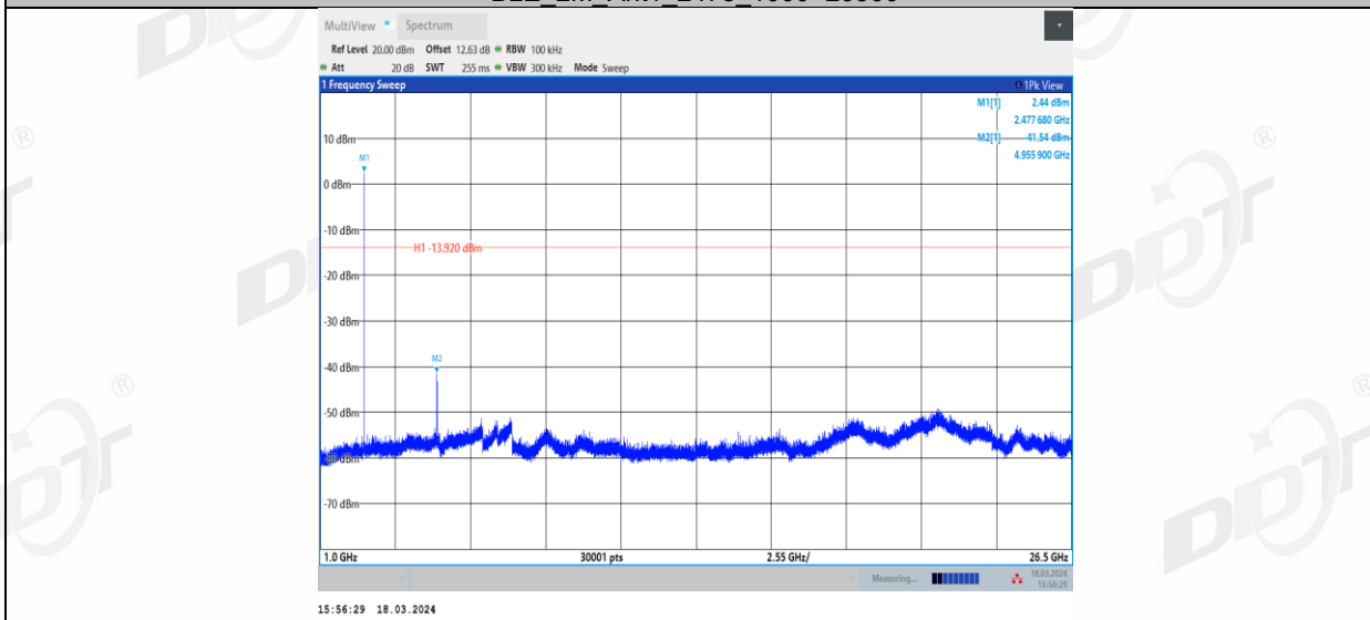
BLE_2M_Ant1_2478_1000~26500
