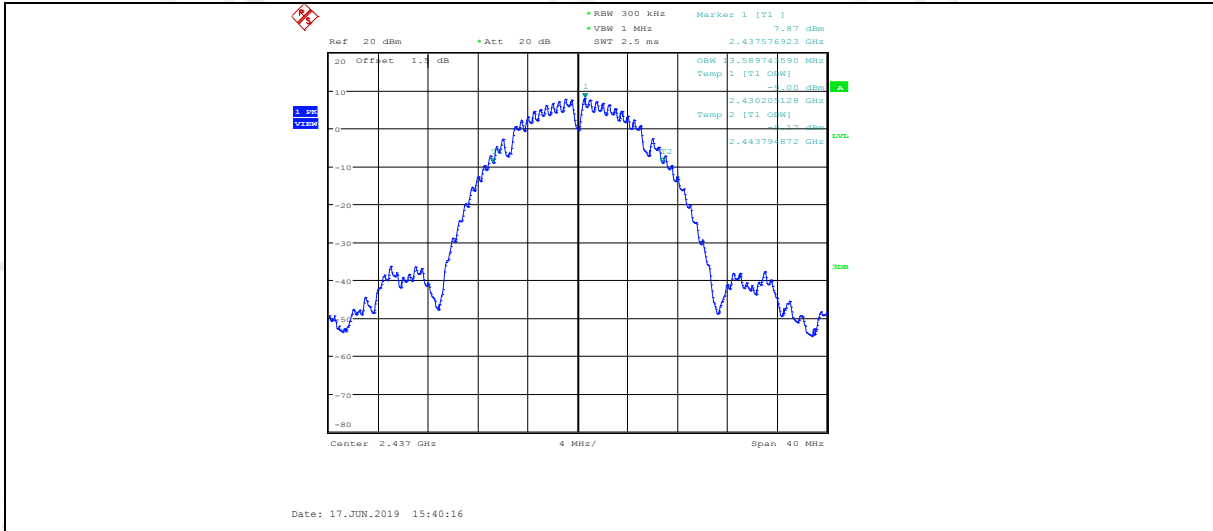
11B_ANT2_2437_99% Bandwidth
