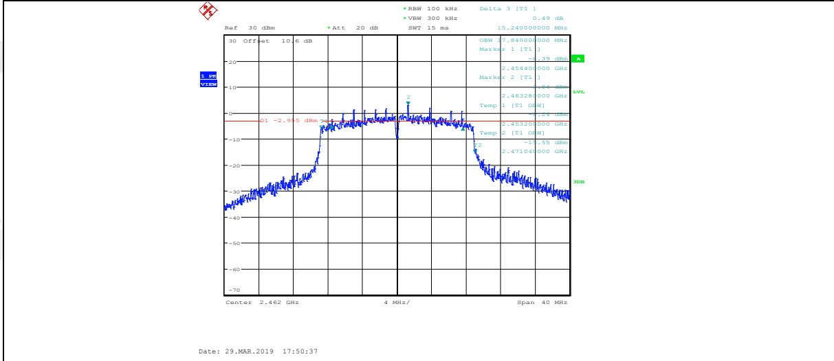
11N20SISO_ANT2_2462_6dB Bandwidth
