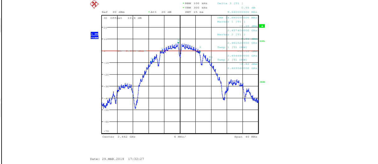
11B_ANT2_2462_6dB Bandwidth
