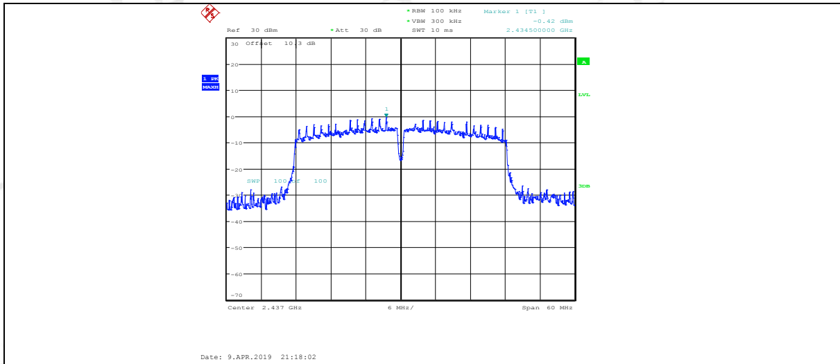
11N40SISO_ANT2_2437_30~1000
