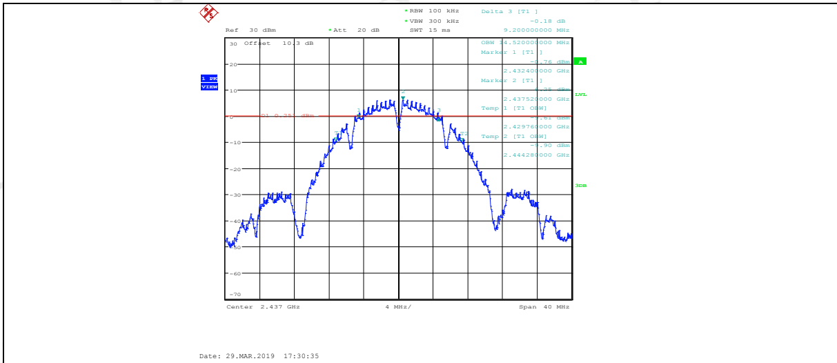
11B_ANT2_2437_6dB Bandwidth
