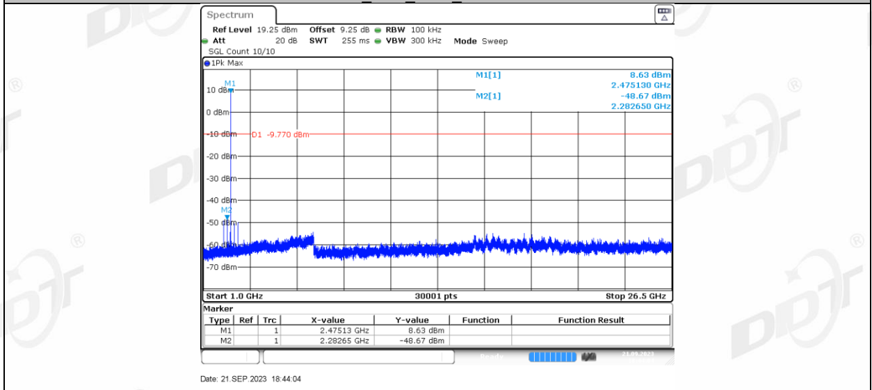
3DH5 Ant1 2475 1000~26500
