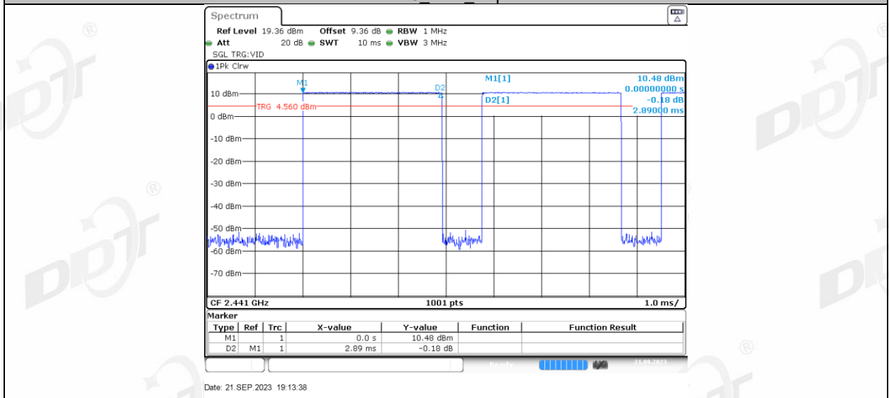
DH5_Ant1_Hop
