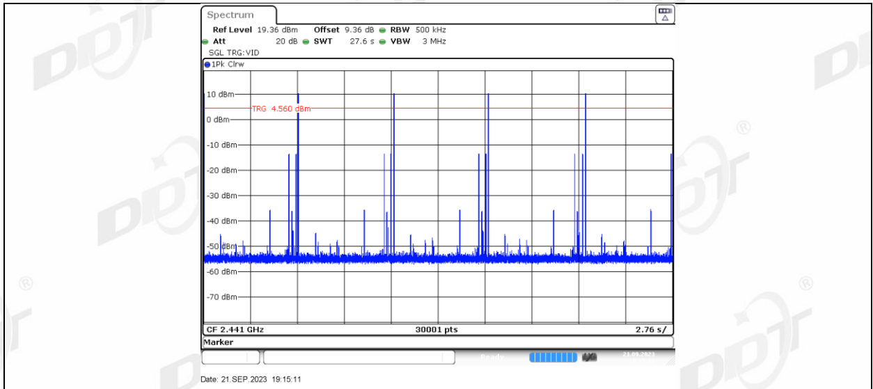
DH5_Ant1_Hop
