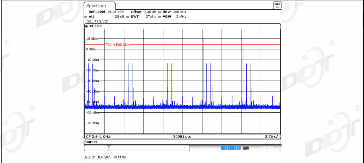
2DH1_Ant1_Hop
