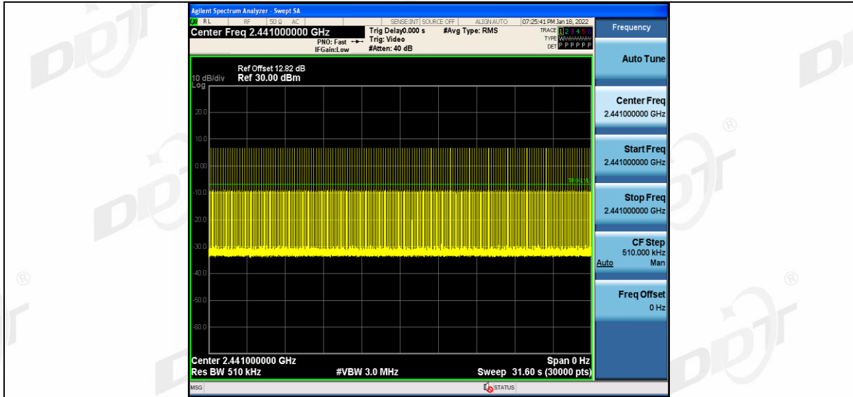
2DH5_Ant1_Hop
