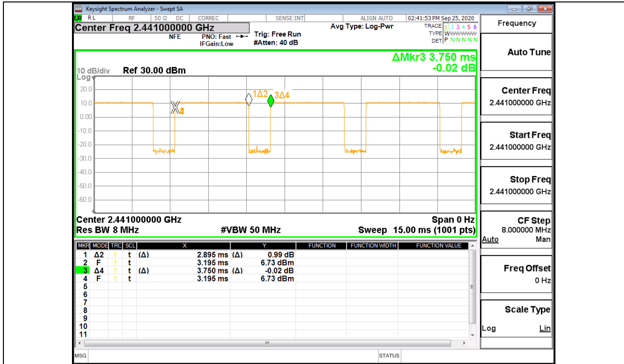
DH5_Ant1_2441
