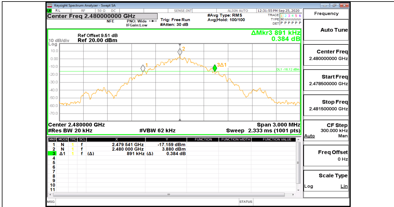
DH5_Ant1_2480
