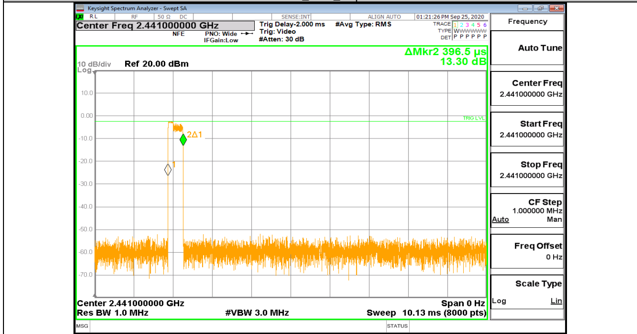
3DH1_Ant1_Hop
