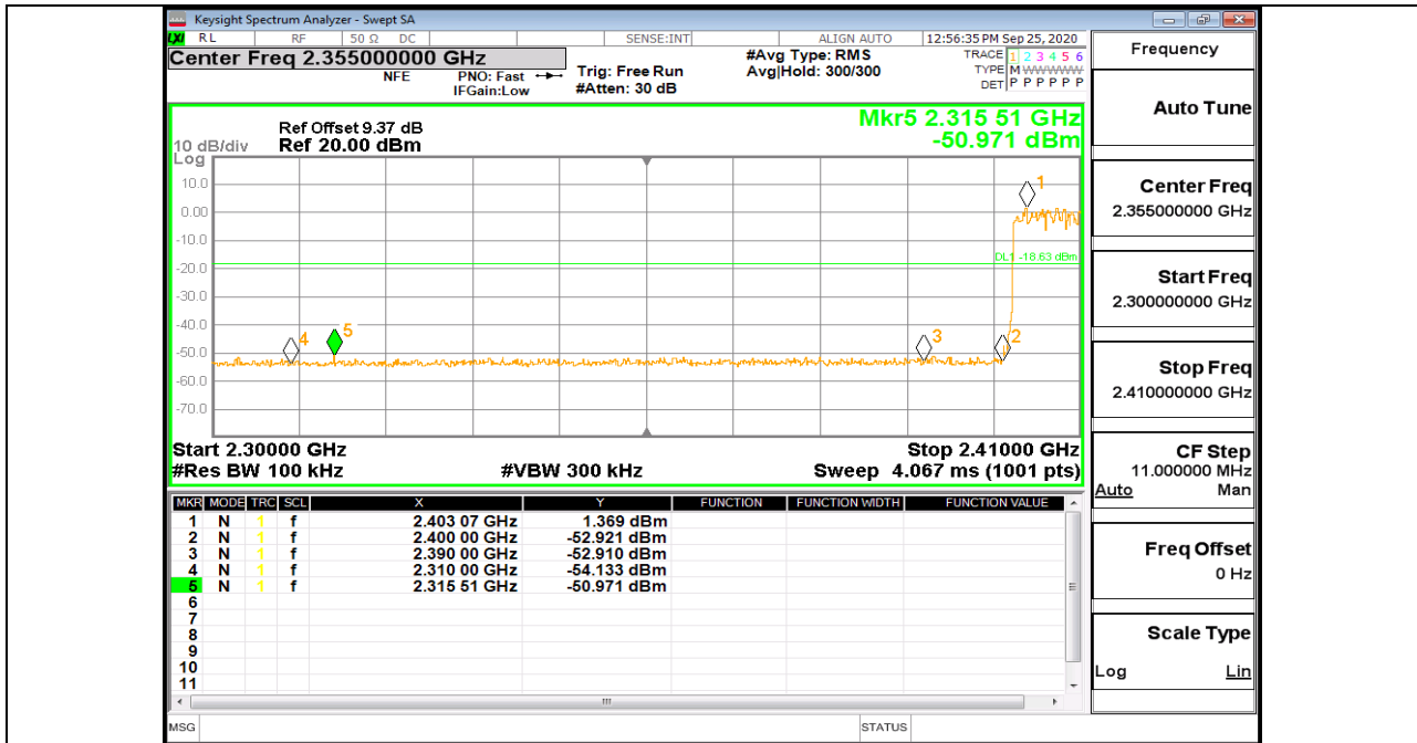
3DH5_Ant1_Low_Hop_2402
