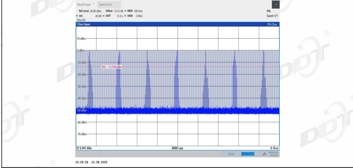
3DH3 Ant1 Hop
