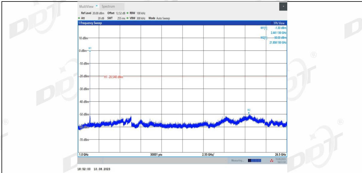
DH5 Ant1 2480 0~Reference
