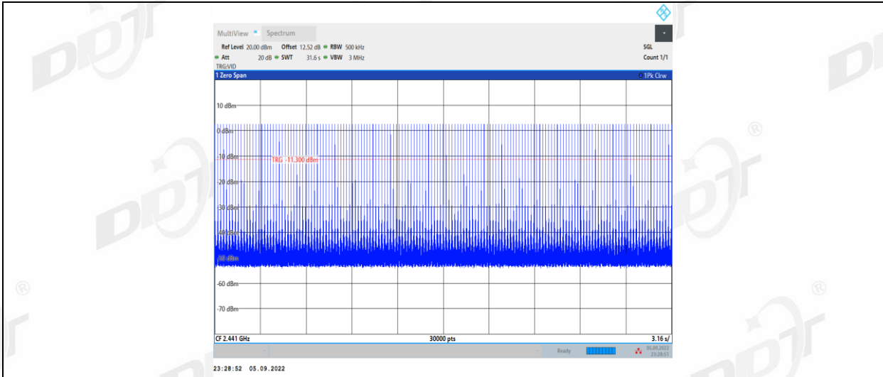
DH5_Ant1_Hop
