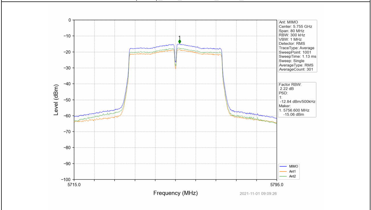
802.11n(HT40)_LCH_5755MHz_MIMO_NTNV
