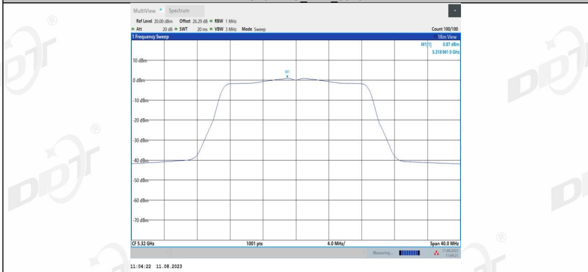
11AC20MIMO_Ant2_5320
