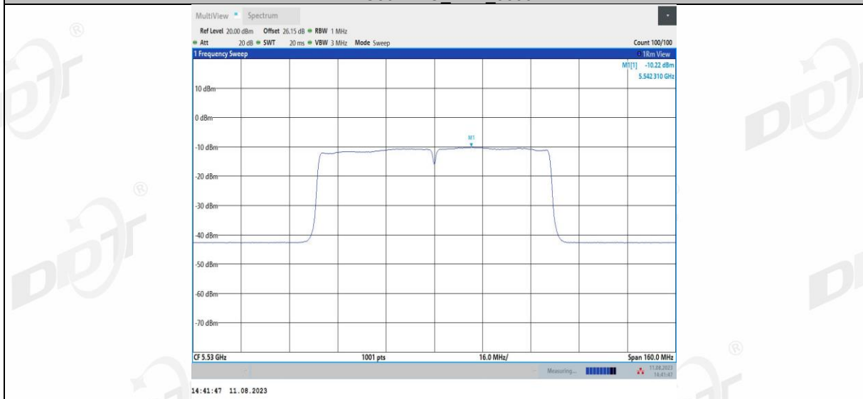
11AC80MIMO_Ant2_5530
