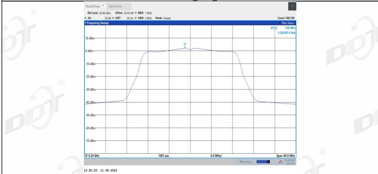
11AC20MIMO_Ant2_5240
