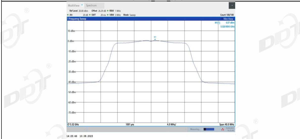
11N20MIMO_Ant2_5320
