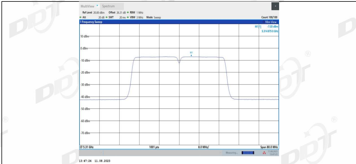
11AC40MIMO_Ant2_5310
