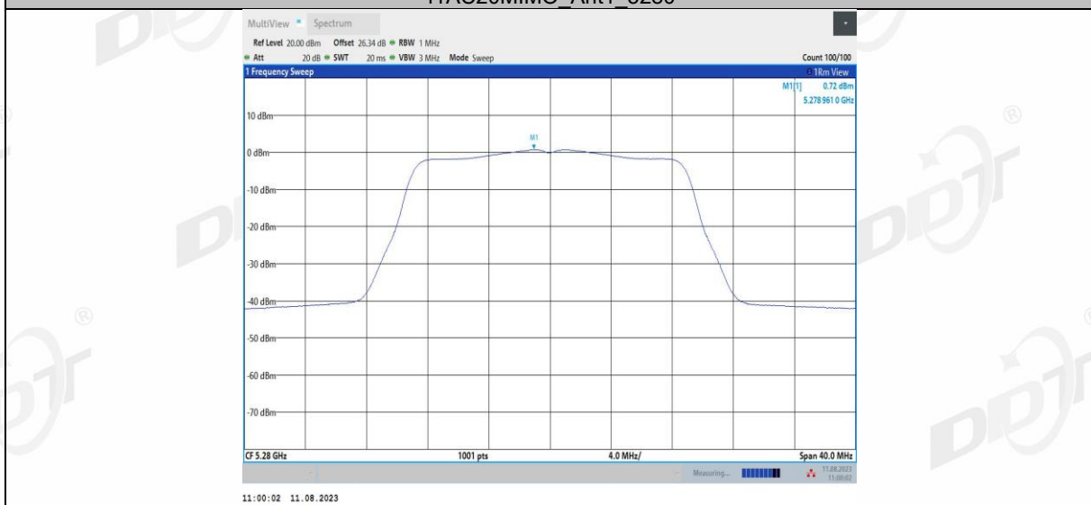
11AC20MIMO_Ant2_5280
