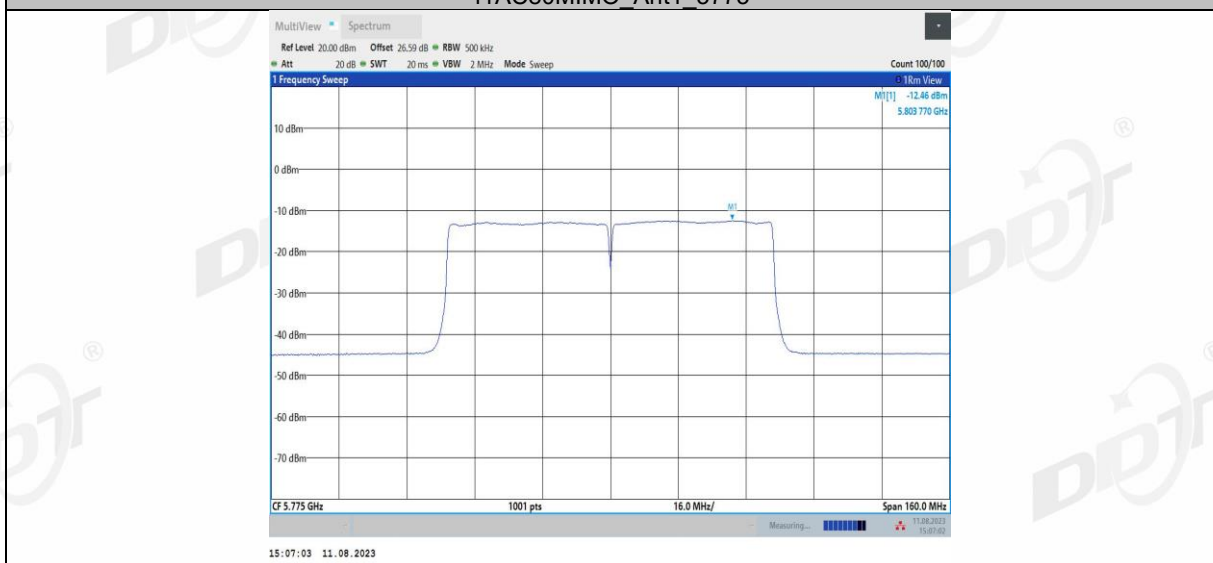
11AC80MIMO_Ant2_5775
