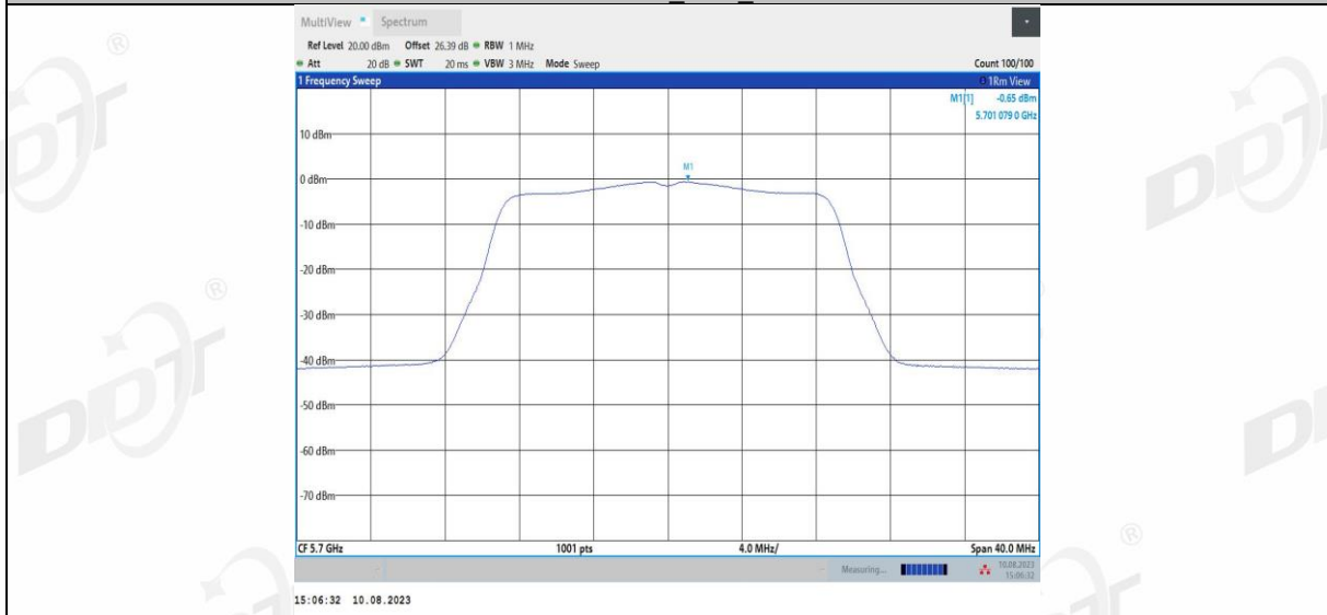
11N20MIMO_Ant2_5700
