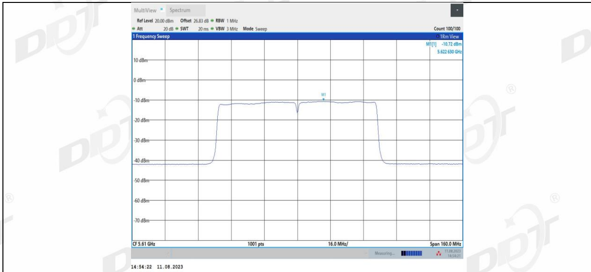
11AC80MIMO_Ant2_5610
