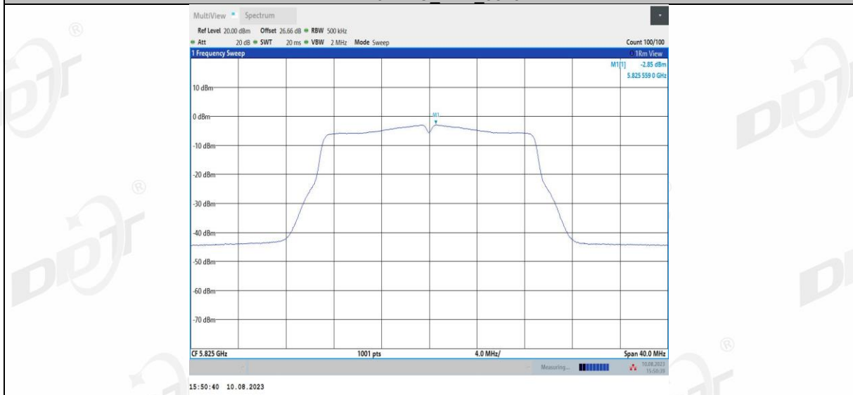
11N20MIMO_Ant2_5825
