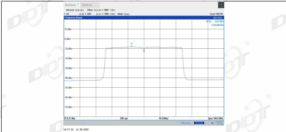
11AC80MIMO_Ant2_5210
