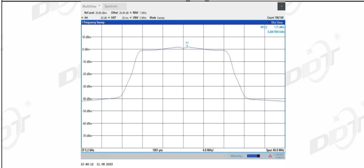
11AC20MIMO_Ant2_5200
