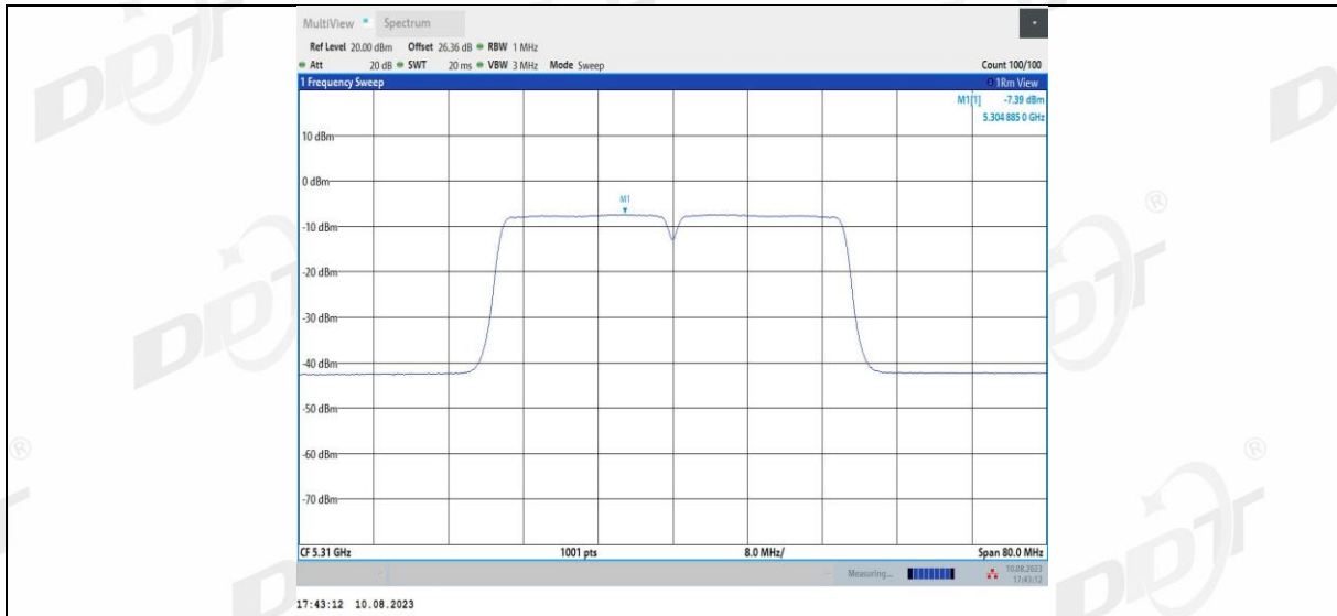
11N40MIMO_Ant2_5310
