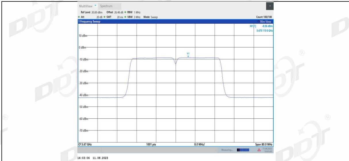
11AC40MIMO_Ant2_5670
