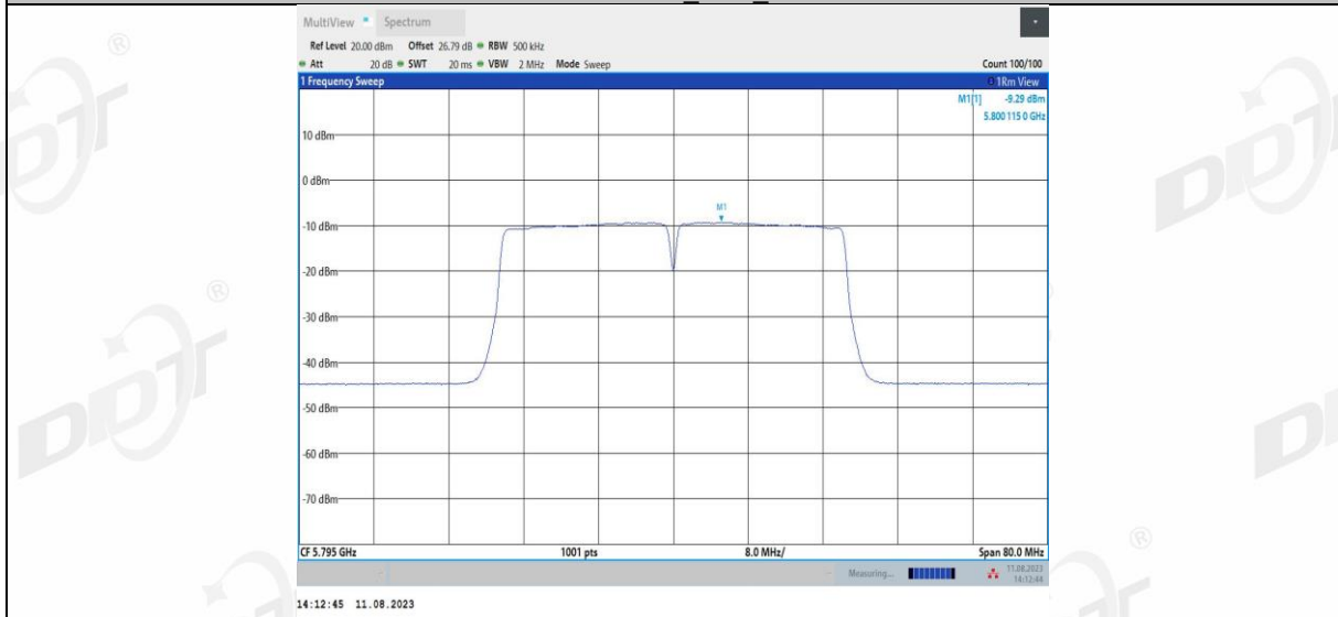
11AC40MIMO_Ant2_5795
