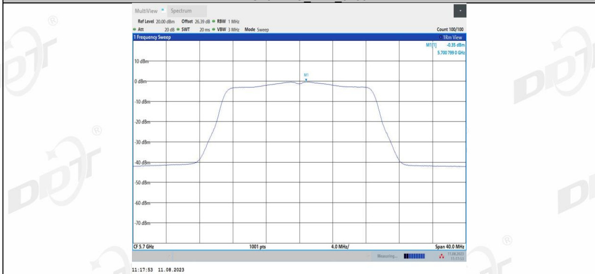
11AC20MIMO_Ant2_5700
