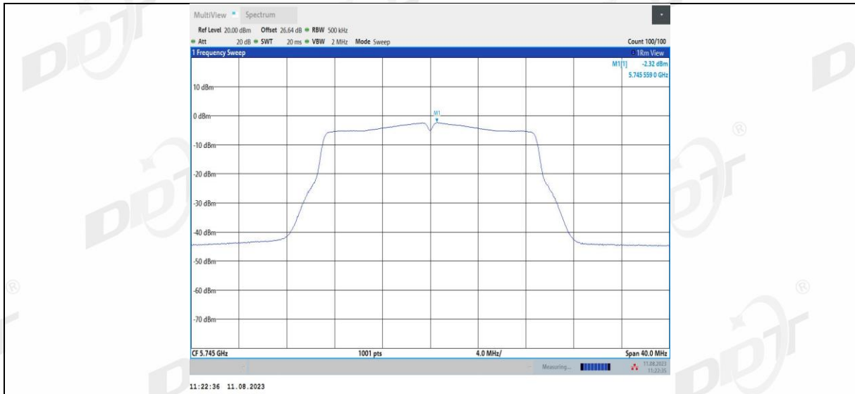
11AC20MIMO_Ant2_5745
