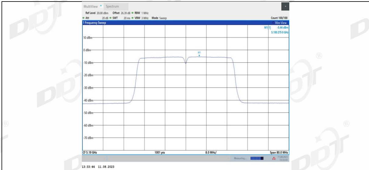
11AC40MIMO_Ant2_5190
