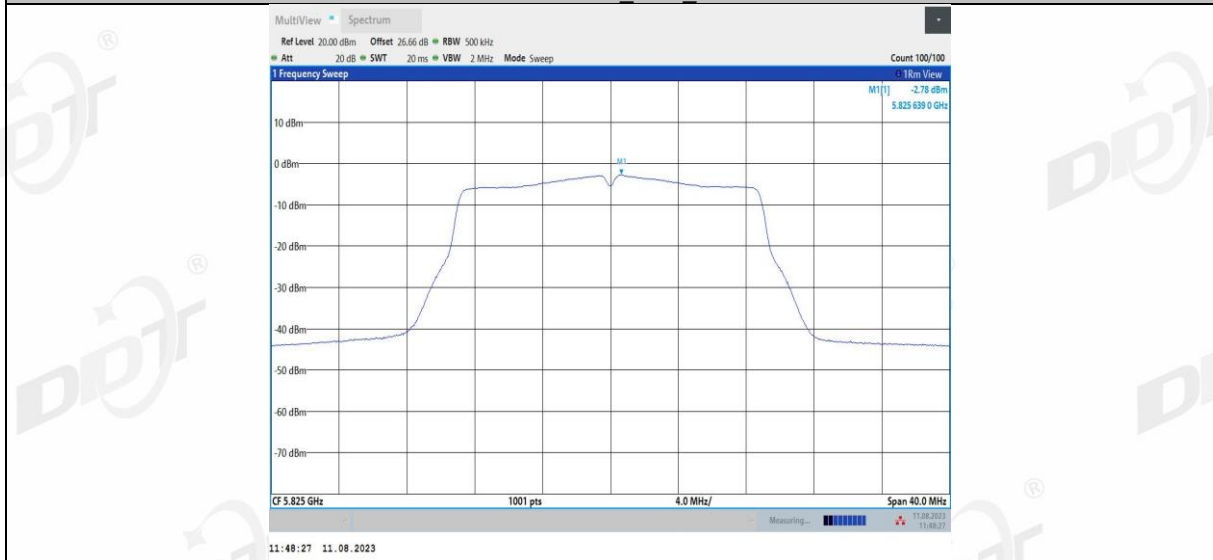
11AC20MIMO_Ant2_5825
