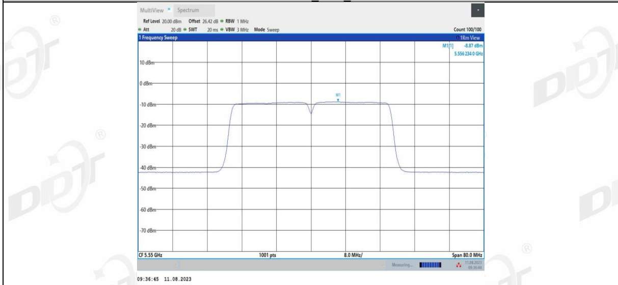
11N40MIMO_Ant2_5550
