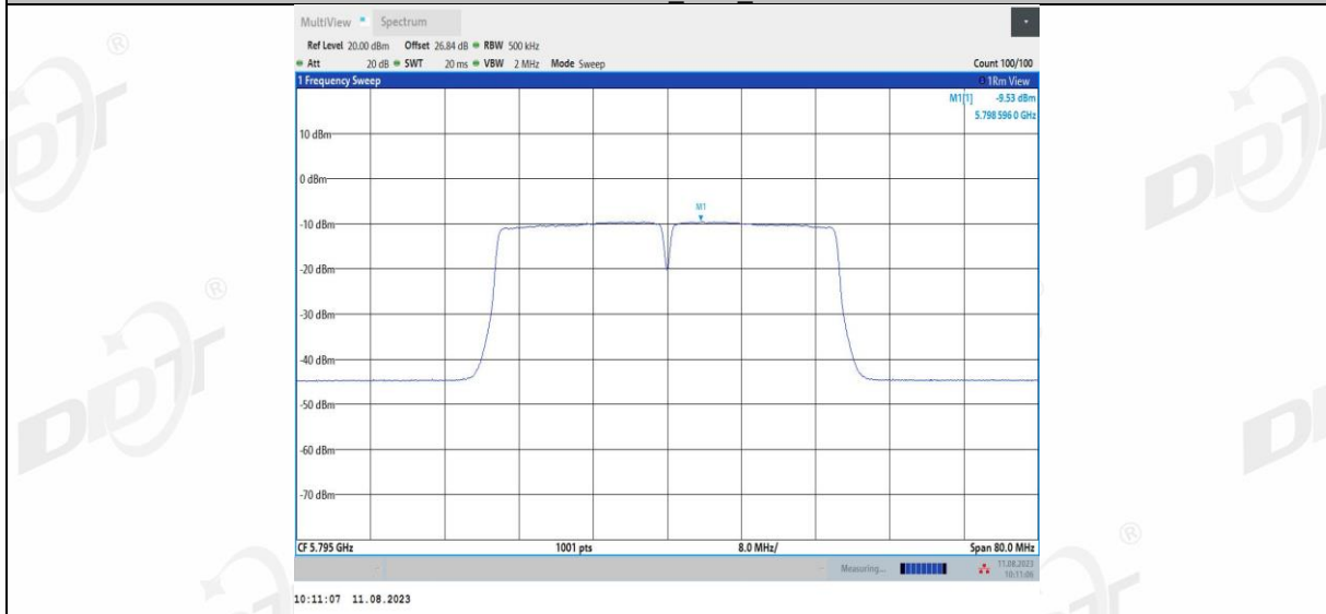
11N40MIMO_Ant2_5795
