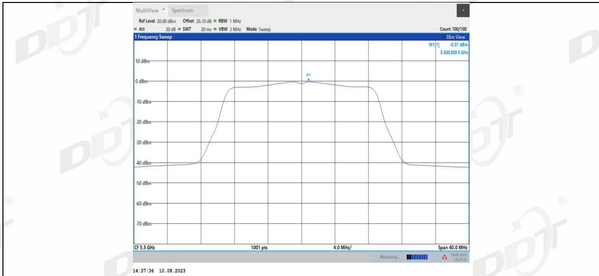
11N20MIMO_Ant2_5500
