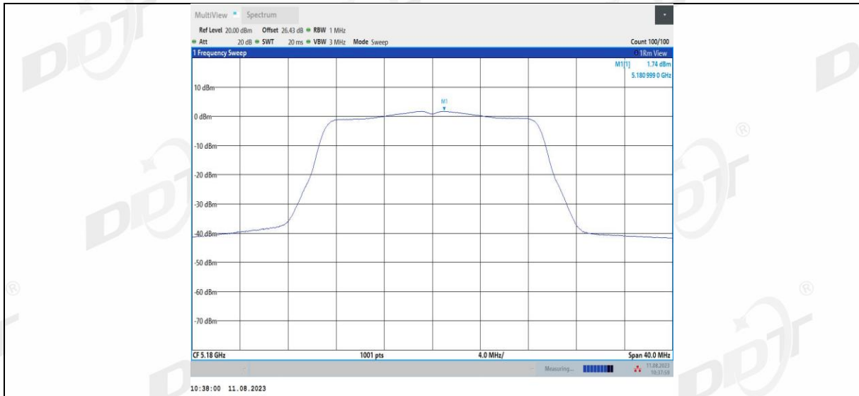
11AC20MIMO_Ant2_5180
