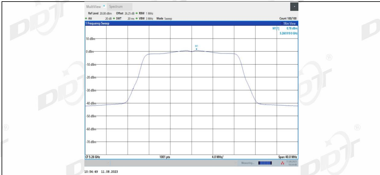
11AC20MIMO_Ant2_5260
