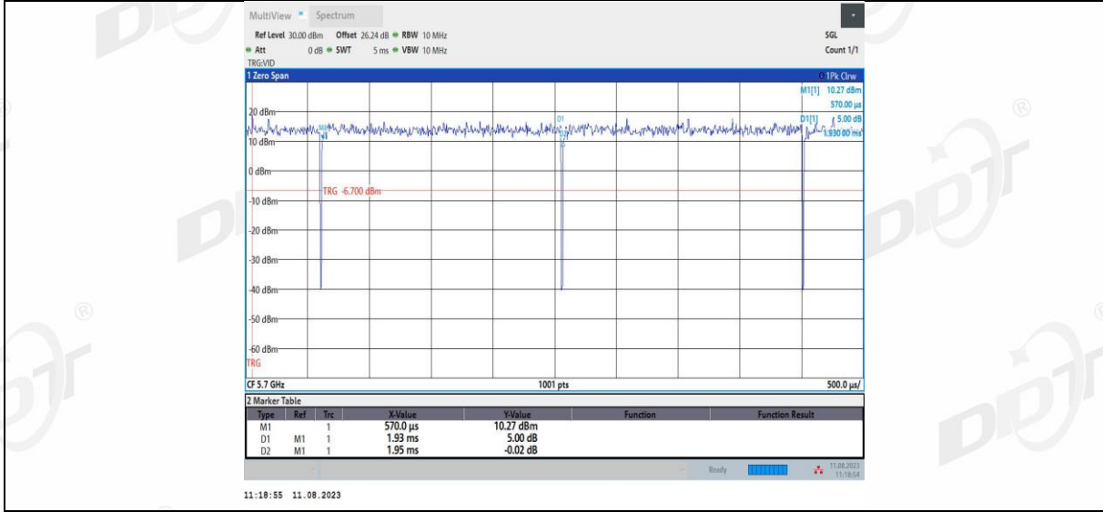
11AC20MIMO_Ant1_5745
