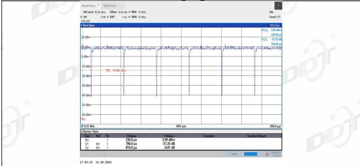
11N40MIMO_Ant2_5510
