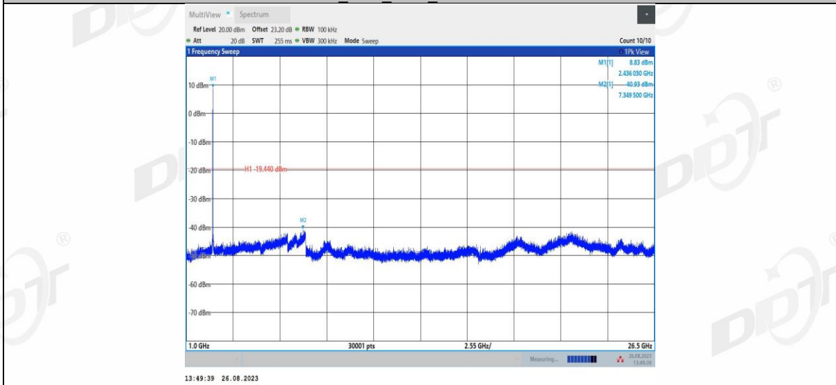
11B_Ant1_2462_0~Reference
