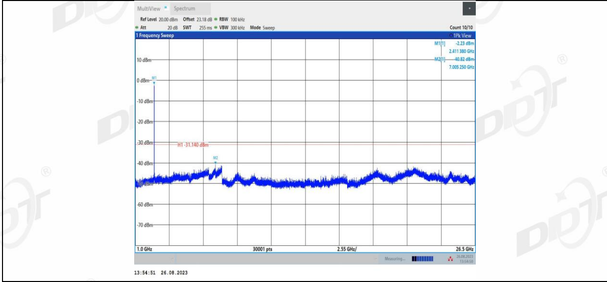
11N20MIMO_Ant1_2437_0~Reference
