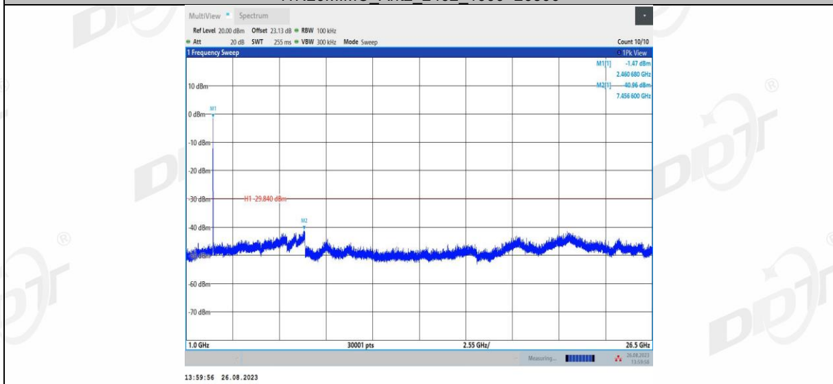
11N20MIMO_Ant2_2462_1000~26500
