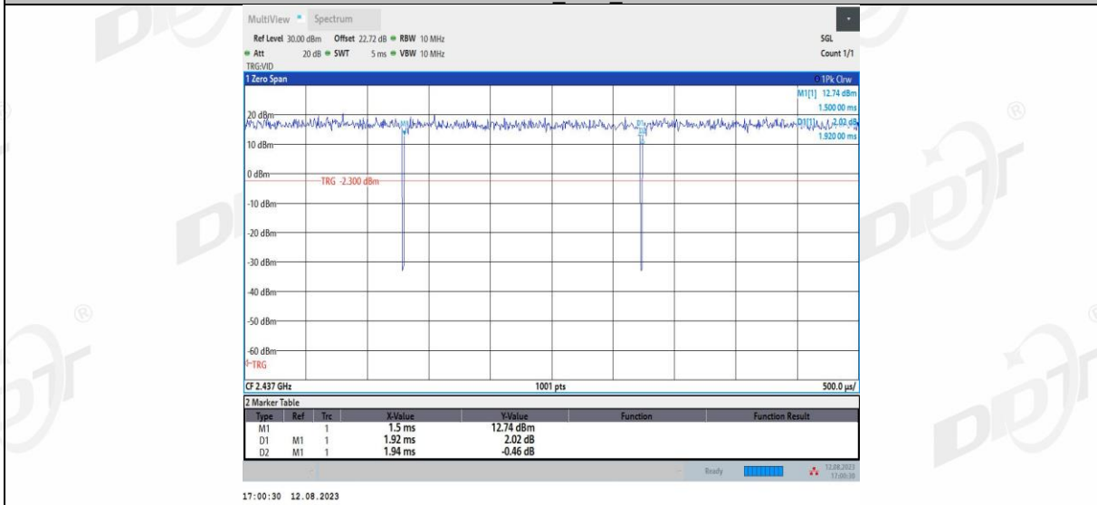
11N20MIMO_Ant2_2437
