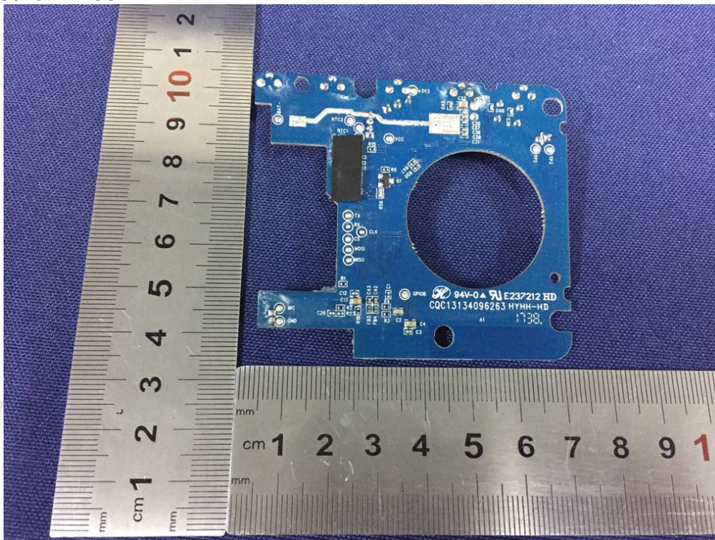
Mainboard: HT862E
