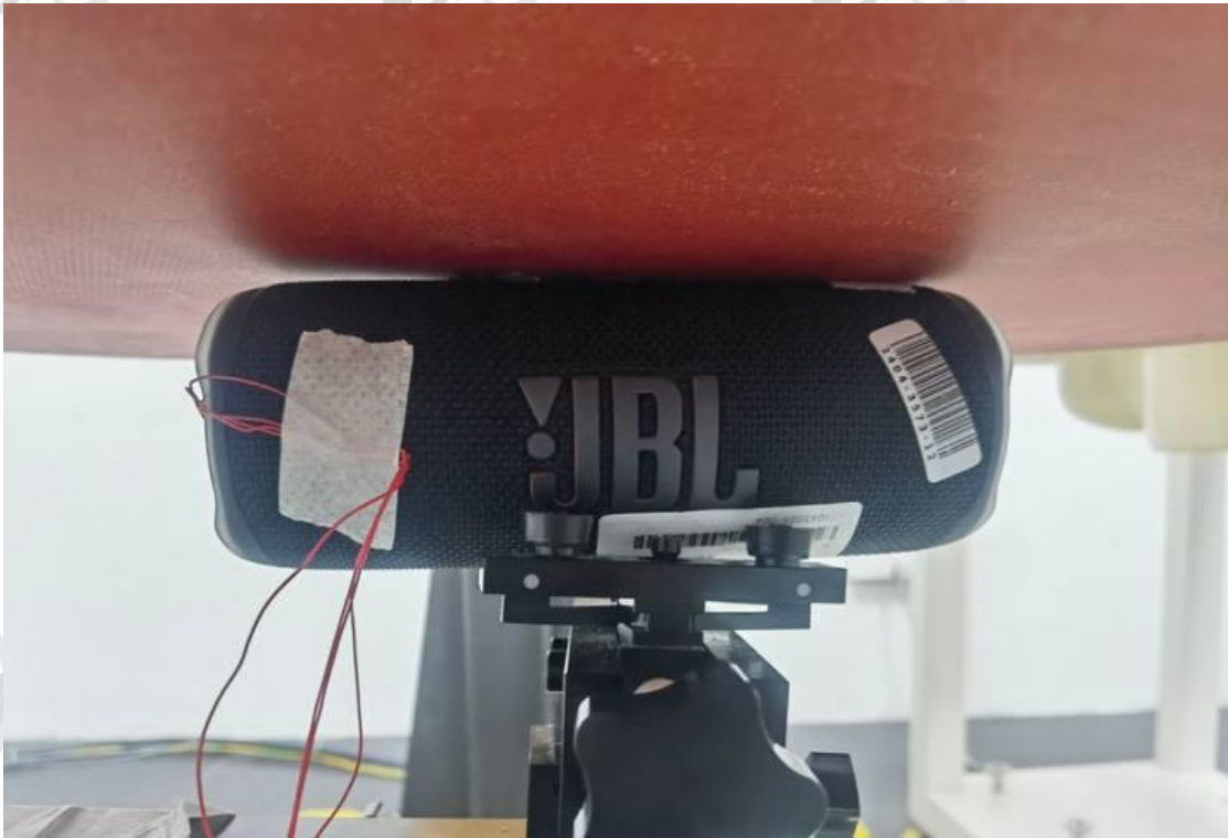
Top Side-0mm
