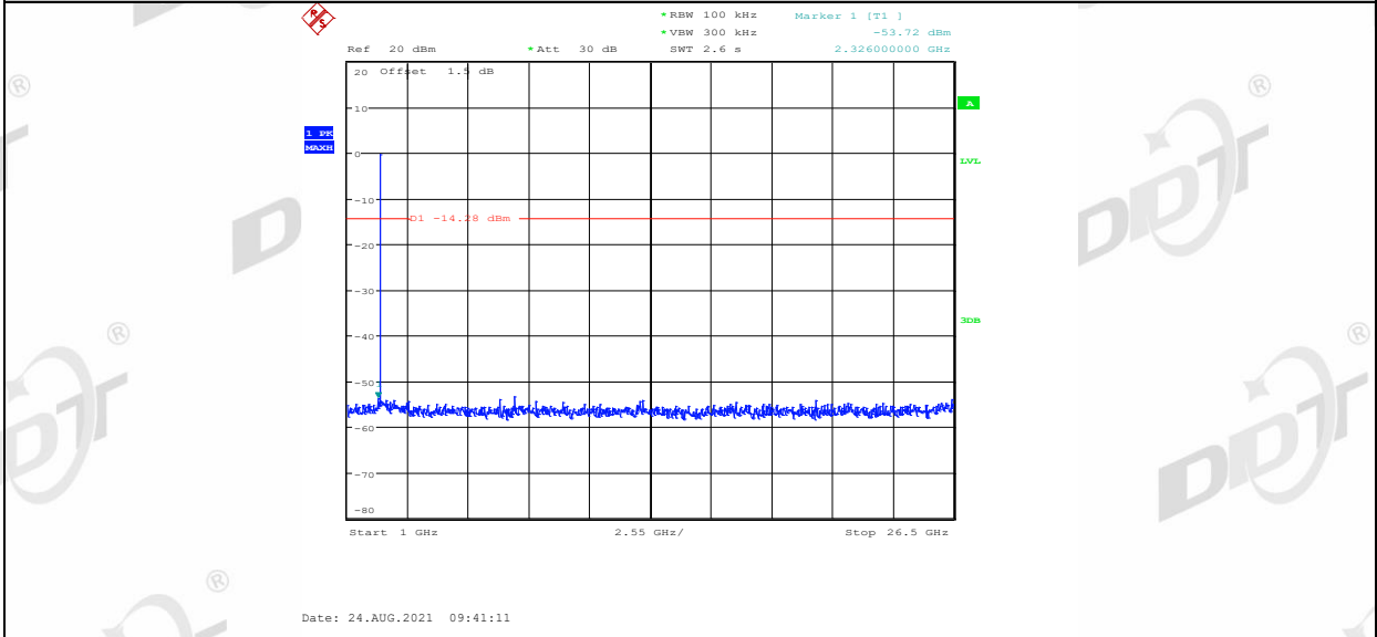
3DH5_ANT1_2480_Ref
