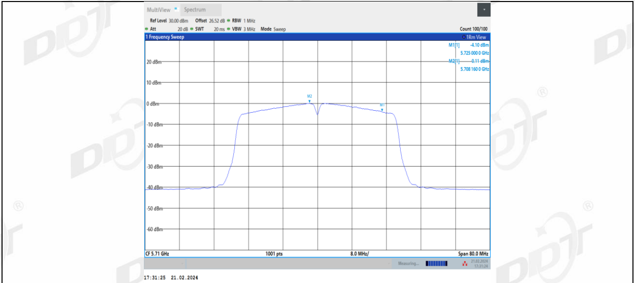
11AC40MIMO_Ant2_5710_UNII-2C
