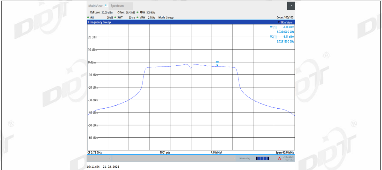
11N20MIMO_Ant2_5720_UNII-3
