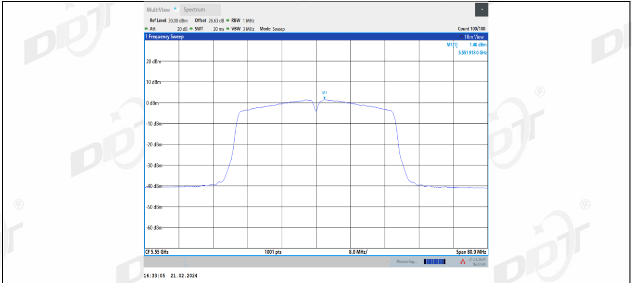
11N40MIMO_Ant2_5550
