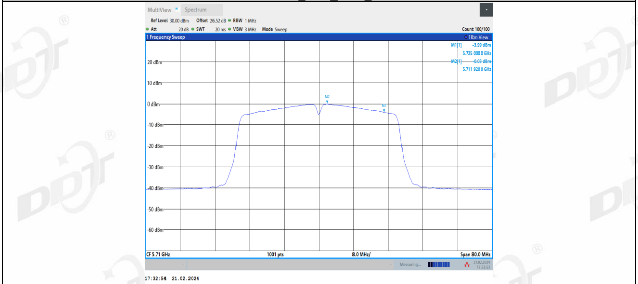
11AC40MIMO_Ant1_5710_UNII-3
