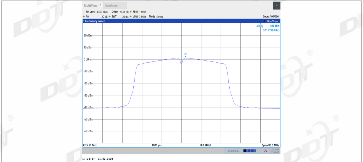
11AC40MIMO_Ant2_5510
