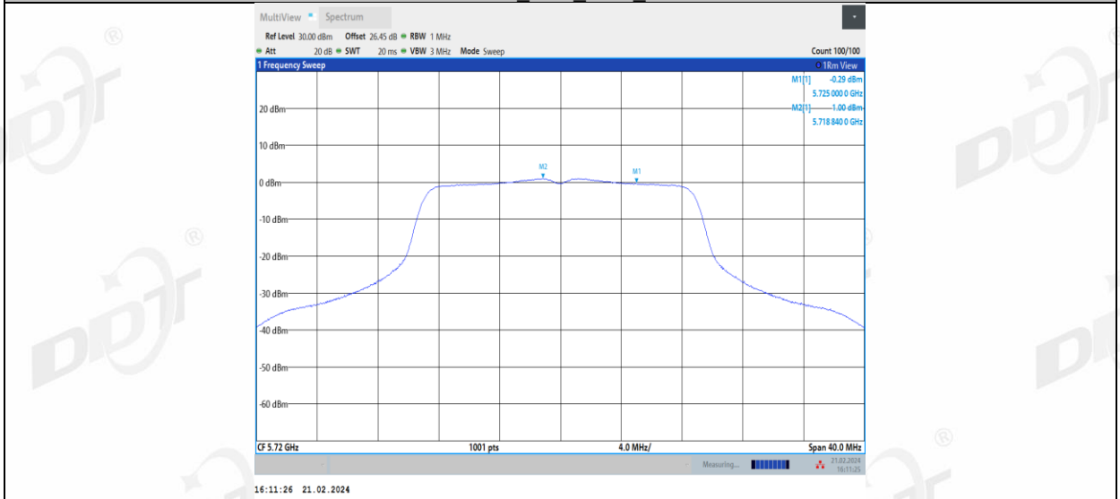
11N20MIMO_Ant2_5720_UNII-2C
