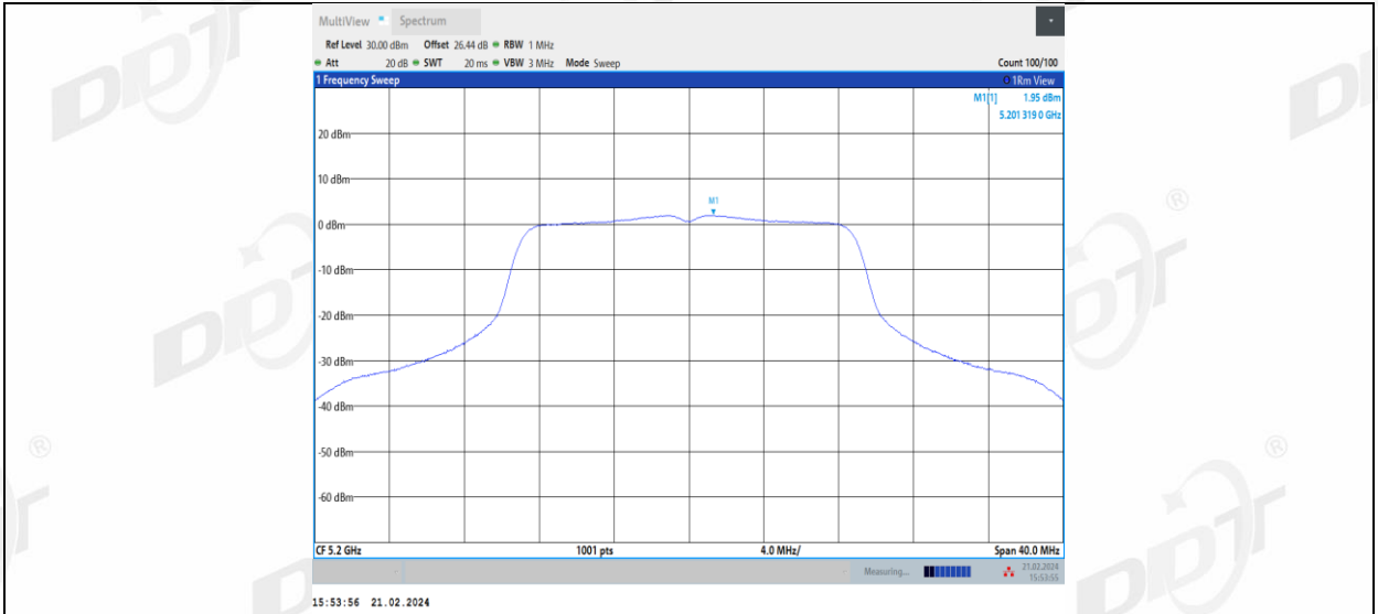
11N20MIMO_Ant2_5200
