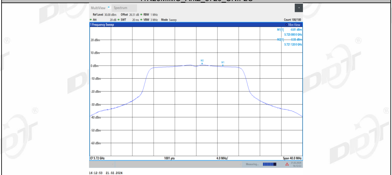
11N20MIMO_Ant1_5720_UNII-3
