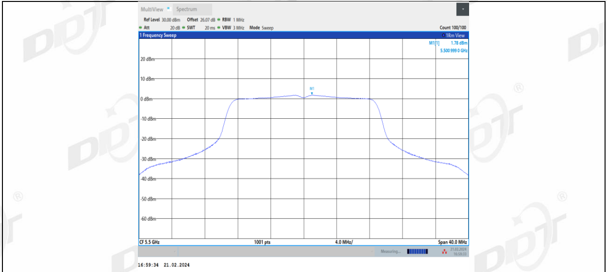
11AC20MIMO_Ant2_5500
