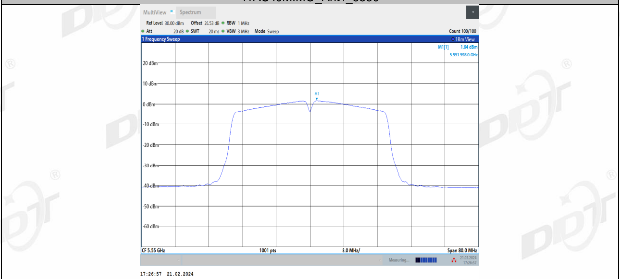
11AC40MIMO_Ant2_5550
