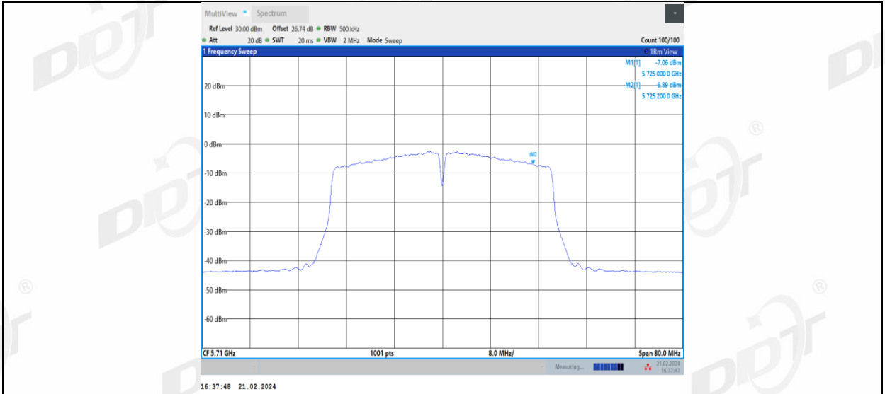
11N40MIMO_Ant2_5710_UNII-3
