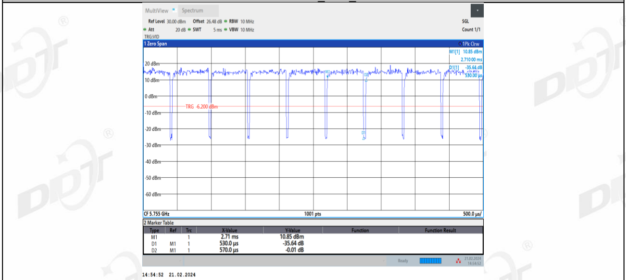
11AX40MIMO_Ant2_5755
