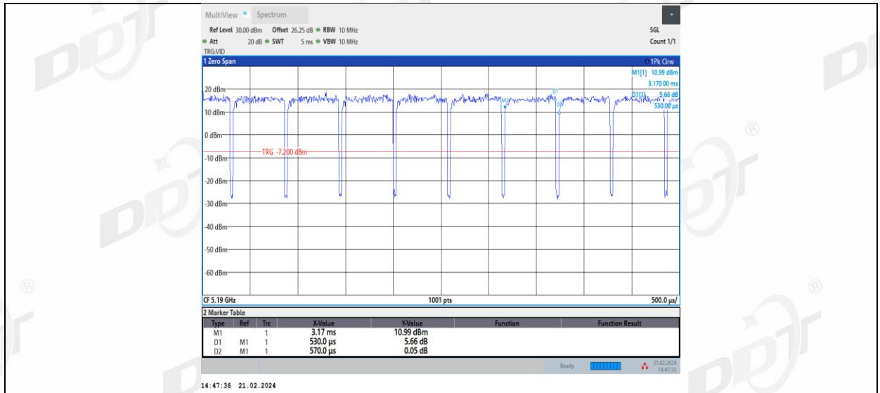
11AX40MIMO_Ant2_5190
