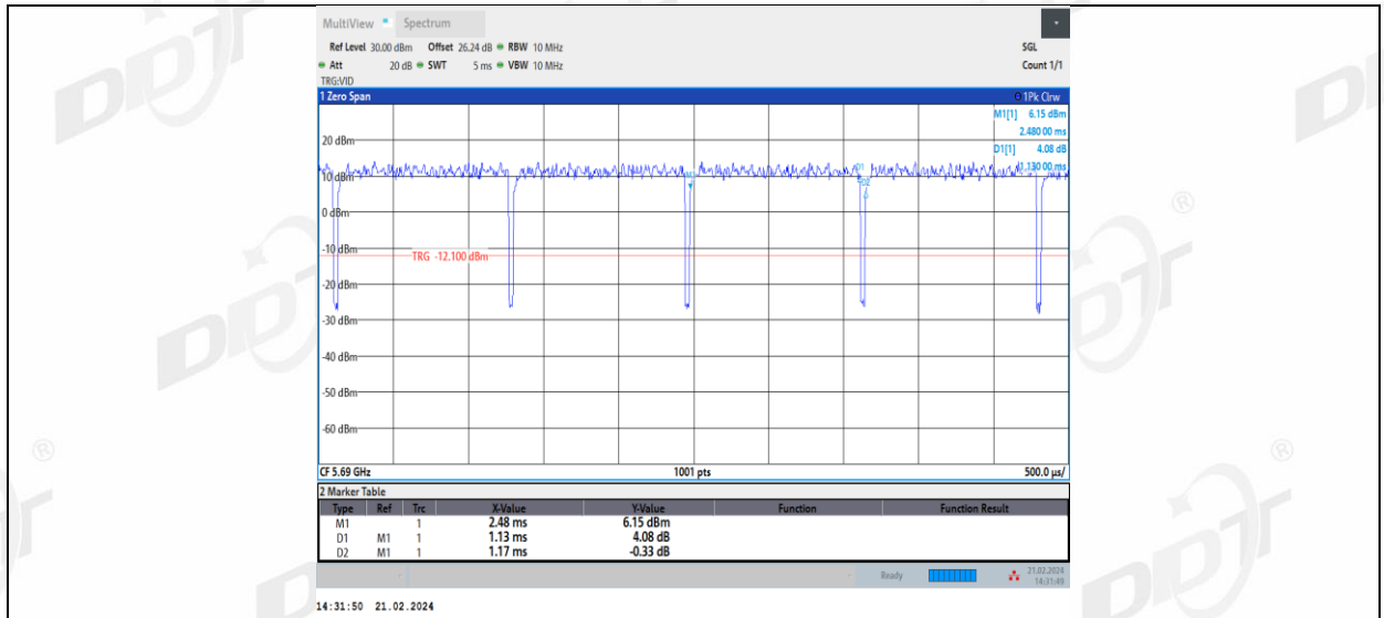
11AC80MIMO_Ant2_5690
