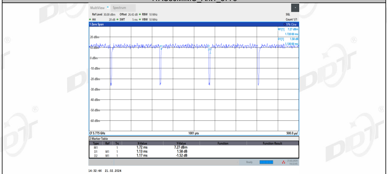
11AC80MIMO_Ant2_5775
