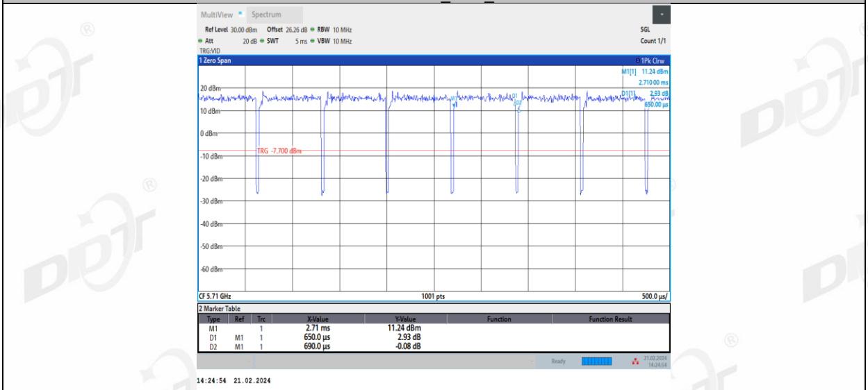
11AC40MIMO_Ant2_5710
