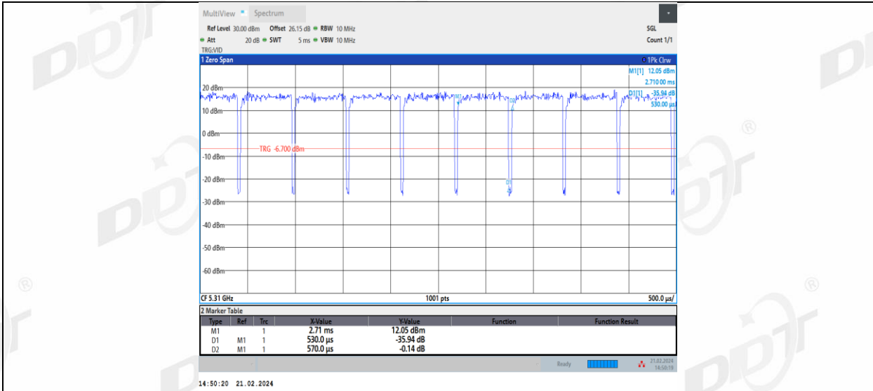
11AX40MIMO_Ant2_5310
