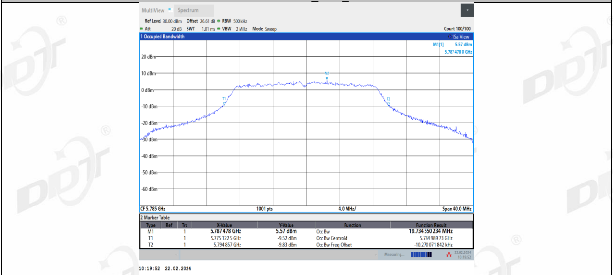
11AC20MIMO_Ant2_5785
