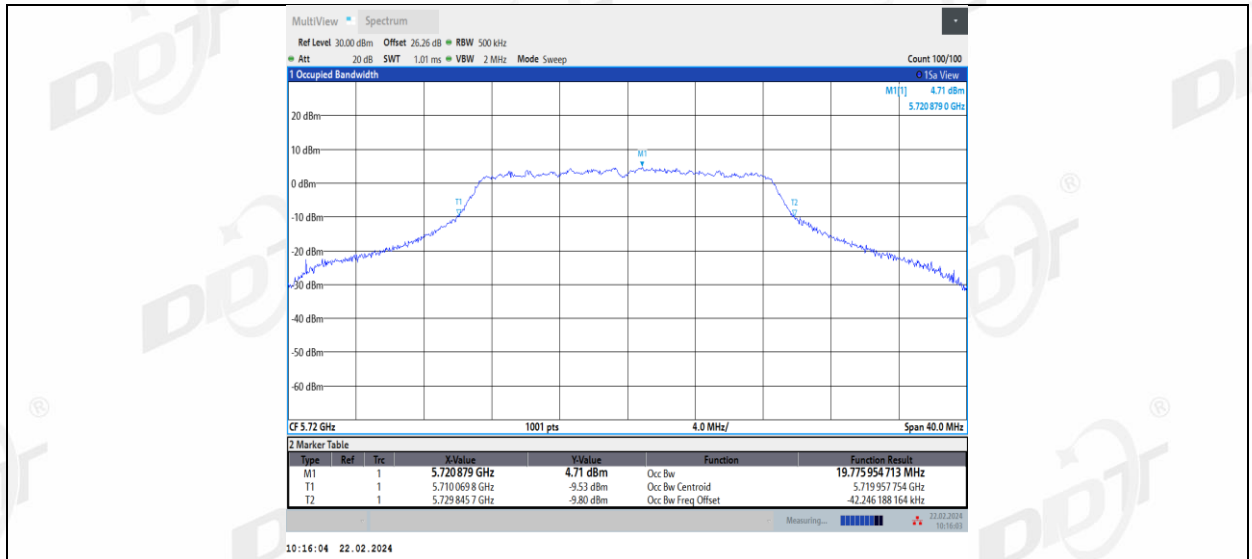
11AC20MIMO_Ant2_5720
