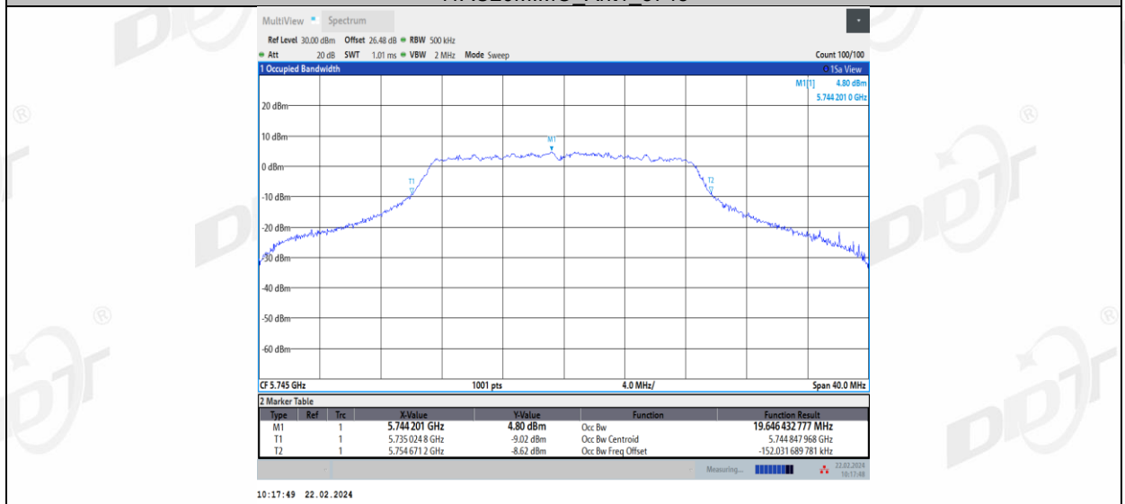
11AC20MIMO_Ant2_5745
