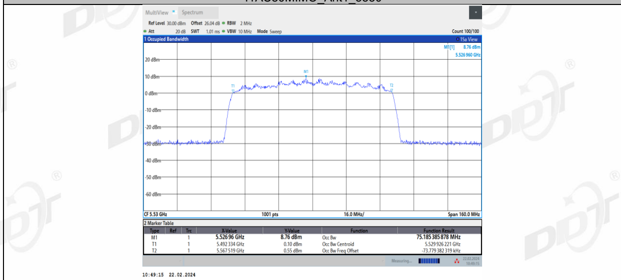
11AC80MIMO_Ant2_5530
