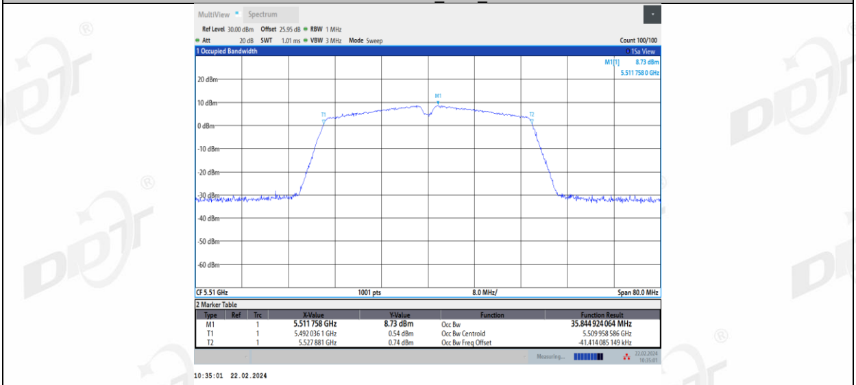
11AC40MIMO_Ant2_5510
