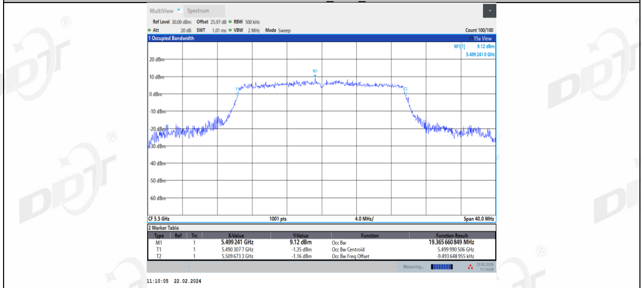
11AX20MIMO_Ant2_5500
