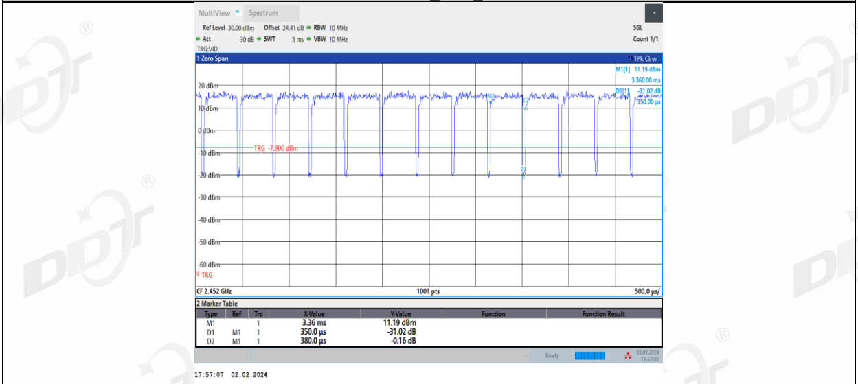
11N40MIMO_Ant2_2452
