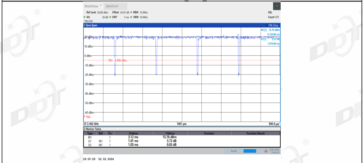
11AX20MIMO_Ant2_2462
