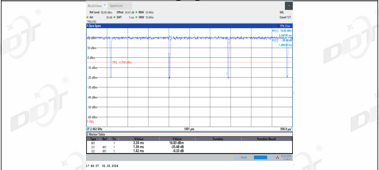
11G_Ant2_2462
