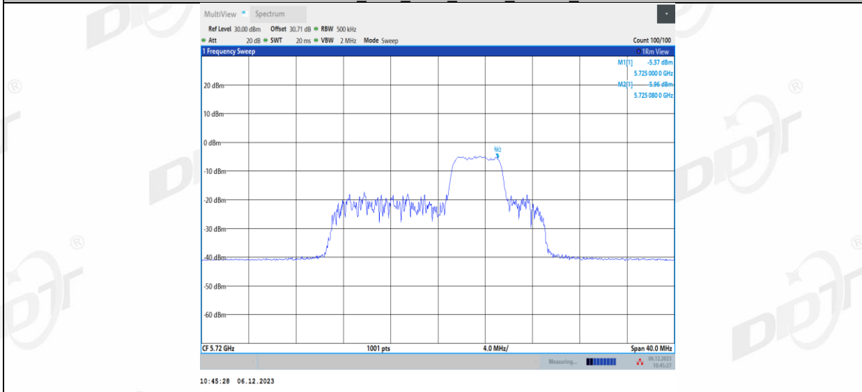
11AX20MIMO_Ant2_5720_UNII-3_52Tone_RU40
