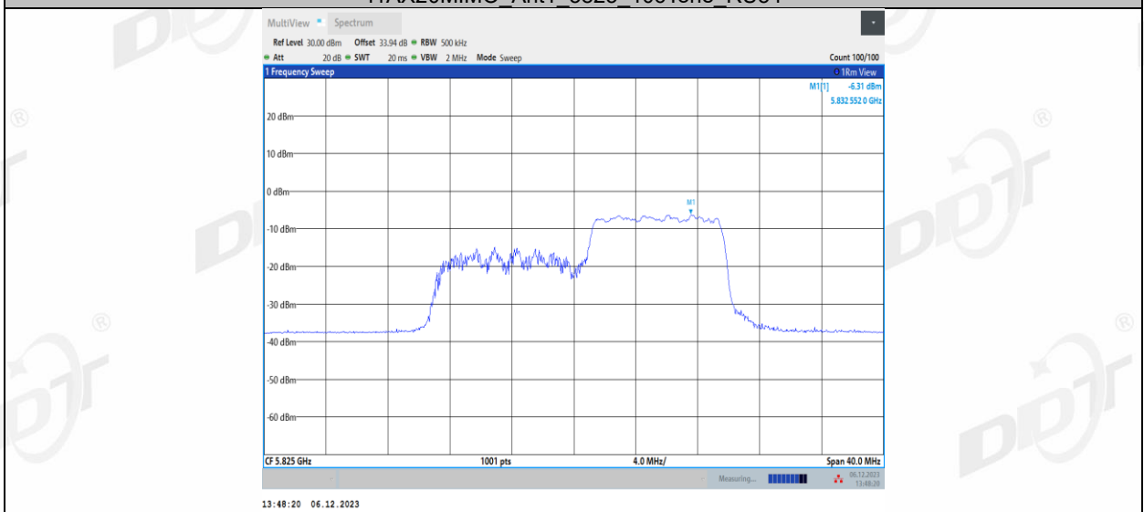
11AX20MIMO_Ant2_5825_26Tone_RU0
