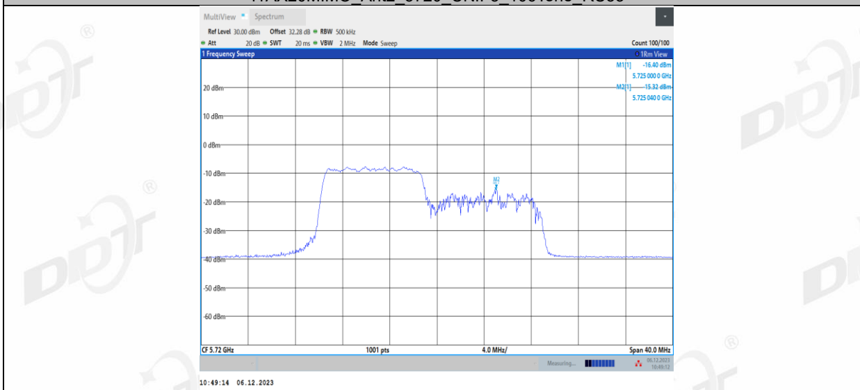
11AX20MIMO_Ant2_5720_UNII-3_106Tone_RU54
