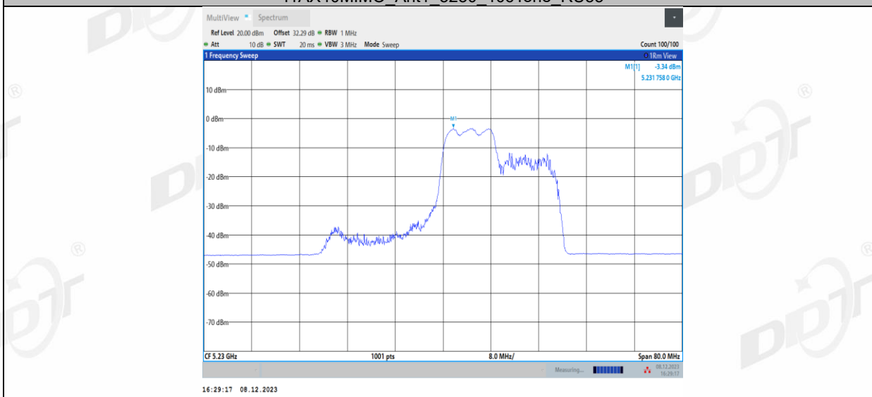
11AX40MIMO_Ant1_5230_106Tone_RU56
