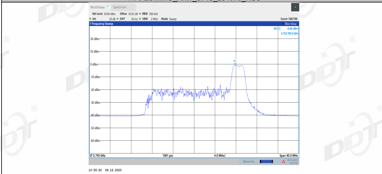
11AX20MIMO_Ant1_5745_52Tone_RU37
