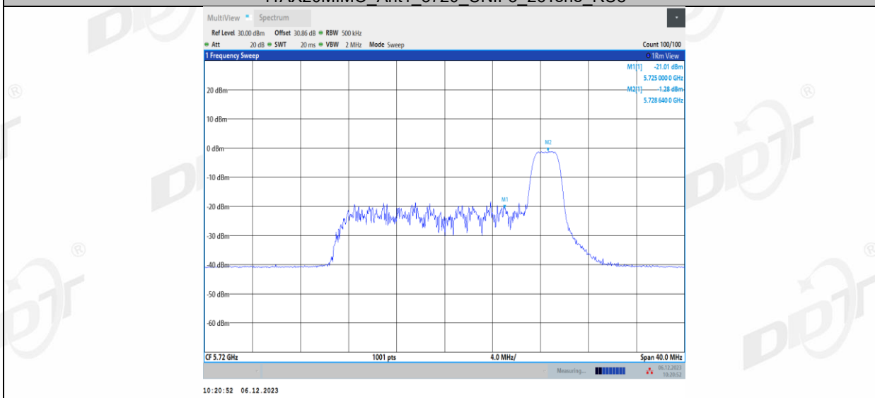
11AX20MIMO_Ant1_5720_UNII-3_52Tone_RU37
