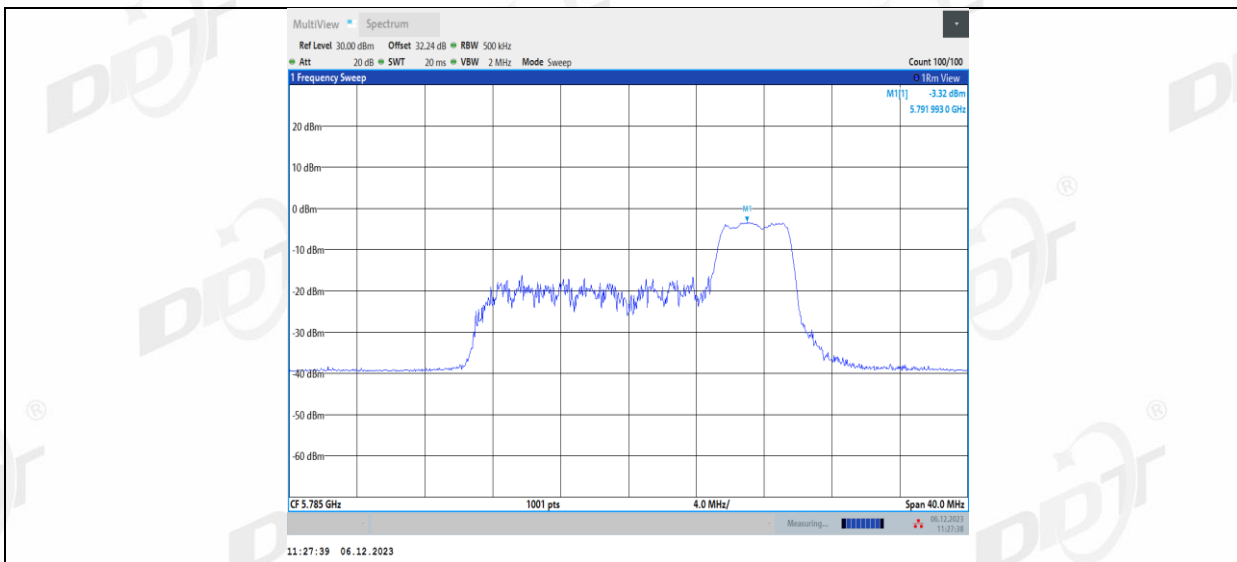
11AX20MIMO_Ant1_5785_106Tone_RU53
