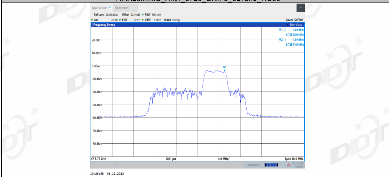
11AX20MIMO_Ant1_5720_UNII-3_52Tone_RU40
