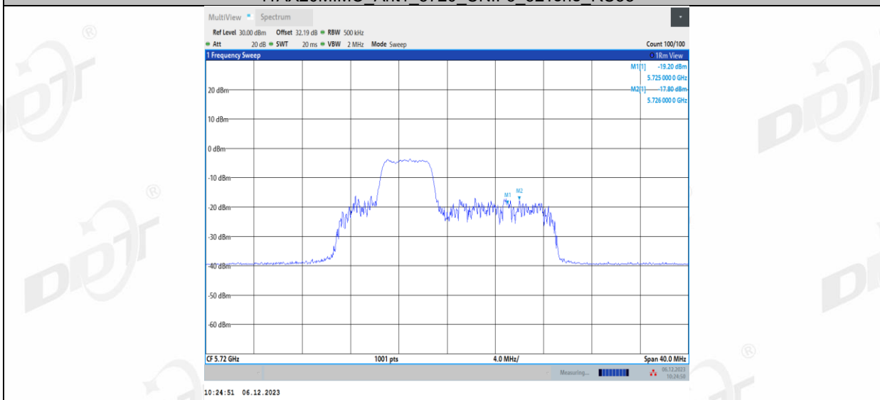
11AX20MIMO_Ant1_5720_UNII-3_52Tone_RU39
