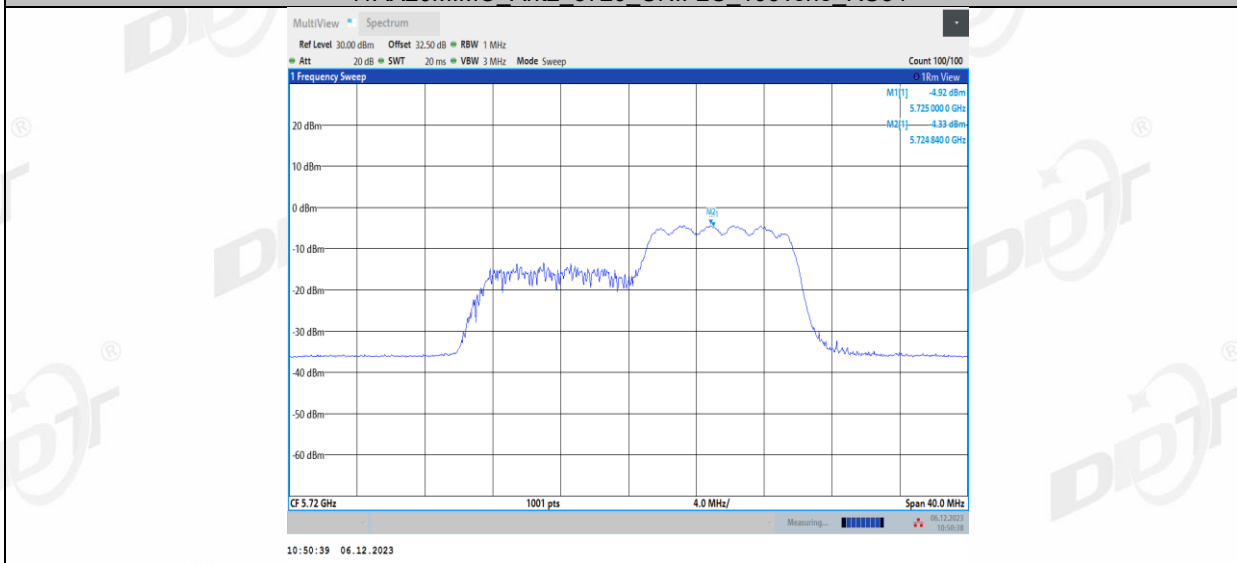
11AX20MIMO_Ant1_5720_UNII-3_26Tone_RU0
