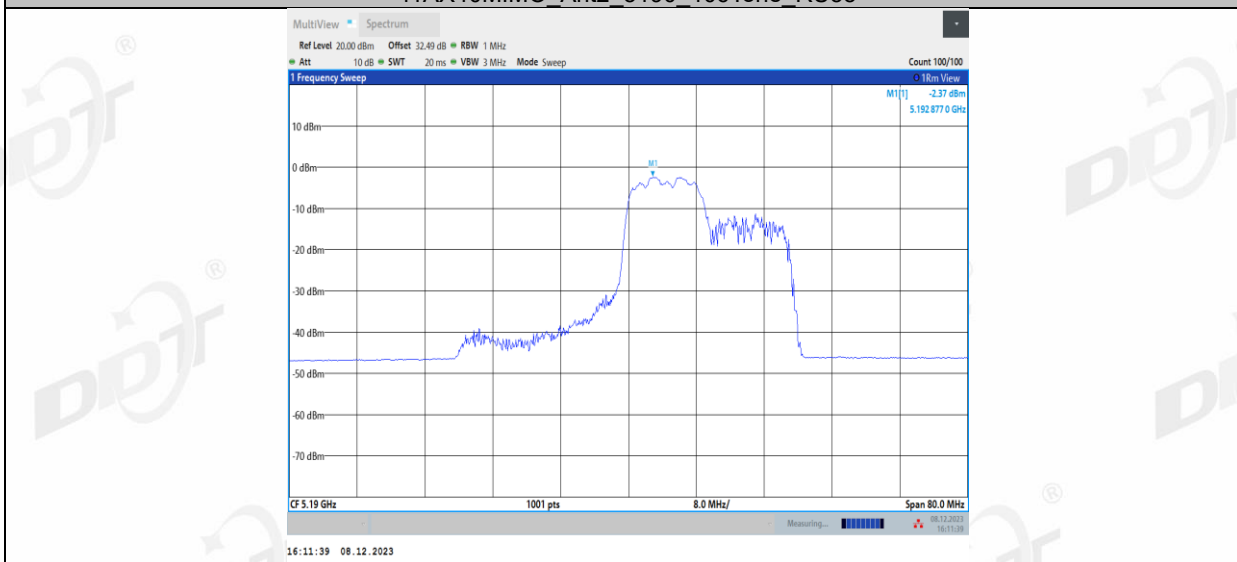
11AX40MIMO_Ant2_5190_106Tone_RU56
