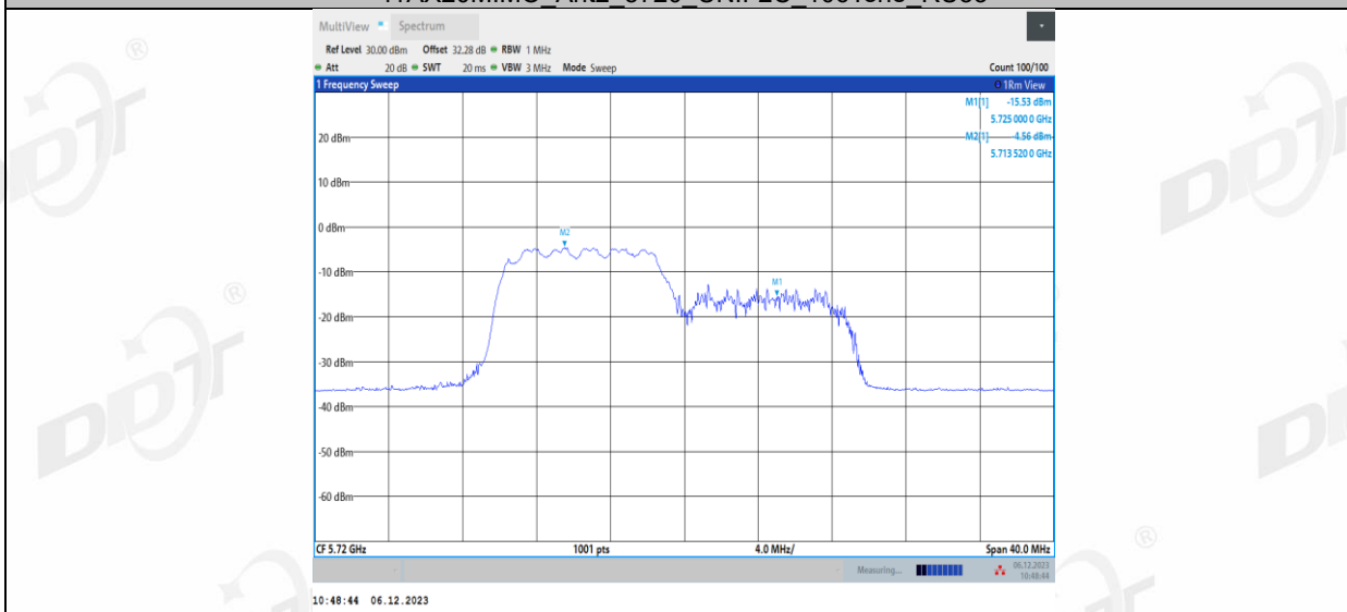
11AX20MIMO_Ant2_5720_UNII-2C_106Tone_RU54
