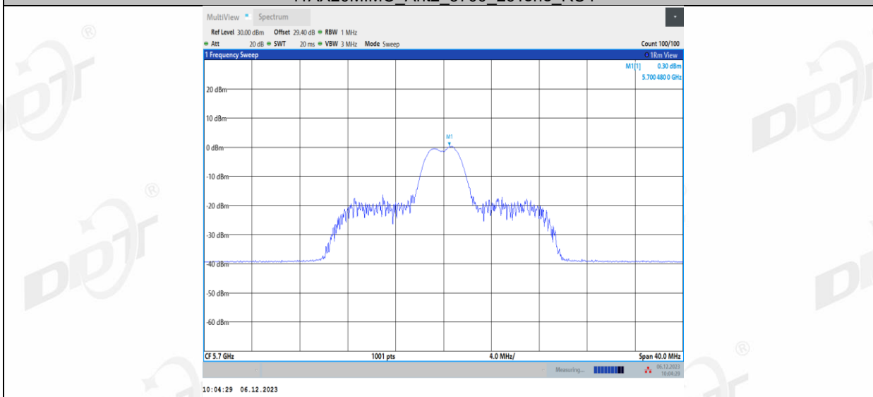
11AX20MIMO_Ant2_5700_26Tone_RU5
