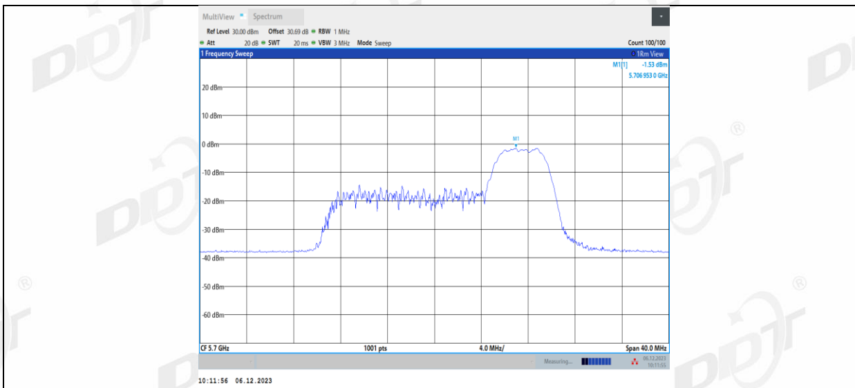
11AX20MIMO_Ant2_5700_106Tone_RU53
