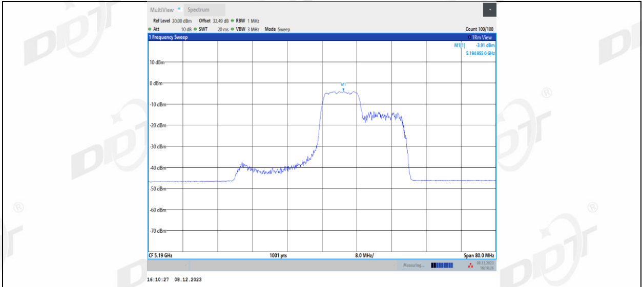
11AX40MIMO_Ant1_5190_106Tone_RU56
