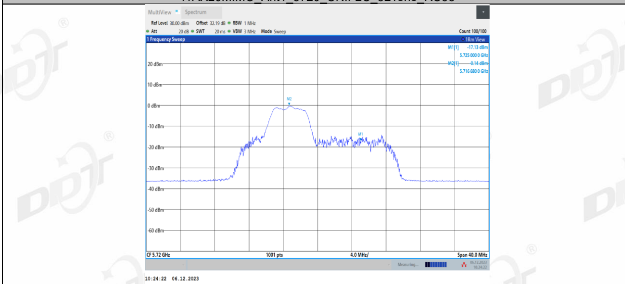
11AX20MIMO_Ant1_5720_UNII-2C_52Tone_RU39
