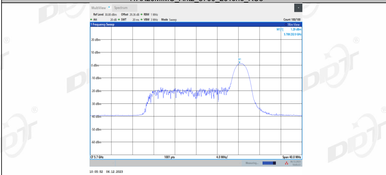
11AX20MIMO_Ant2_5700_52Tone_RU37
