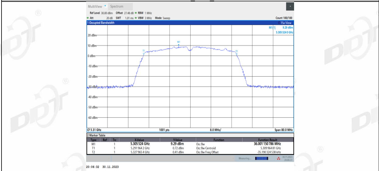
11N40MIMO_Ant2_5310
