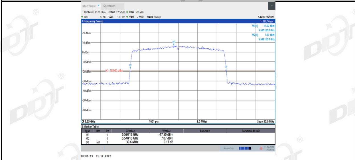
11AX40MIMO_Ant2_5550
