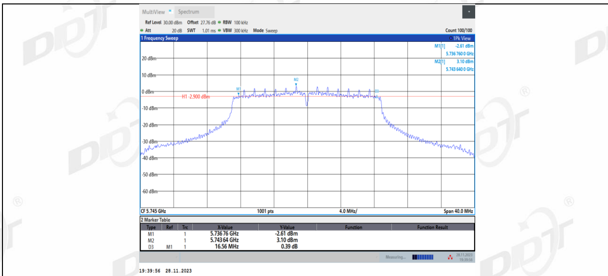
11N20MIMO_Ant2_5745
