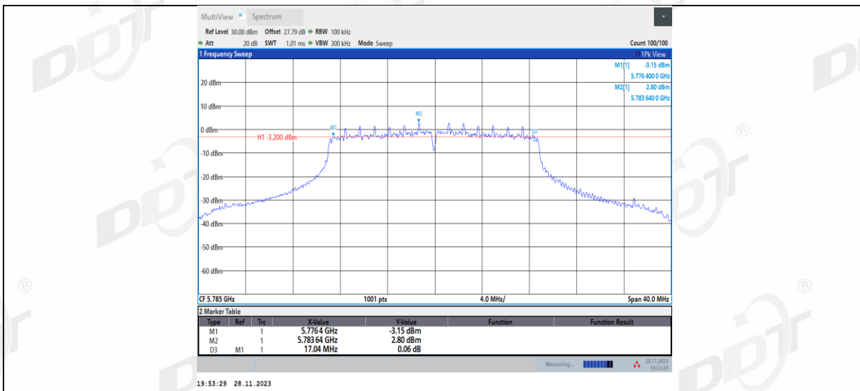
11AC20MIMO_Ant2_5785
