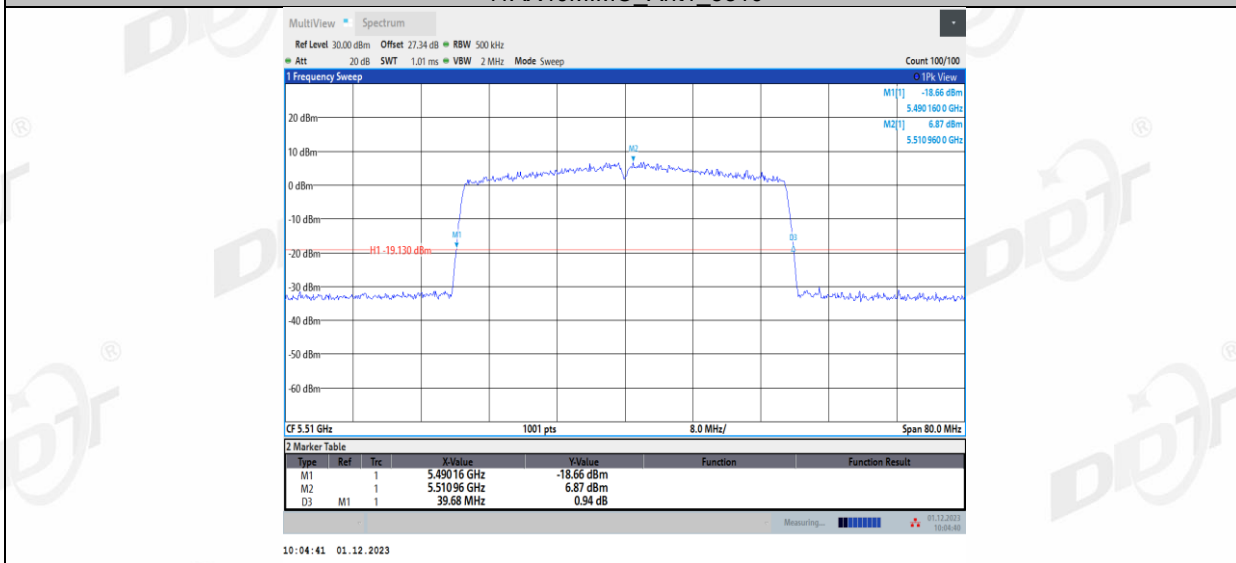
11AX40MIMO_Ant2_5510
