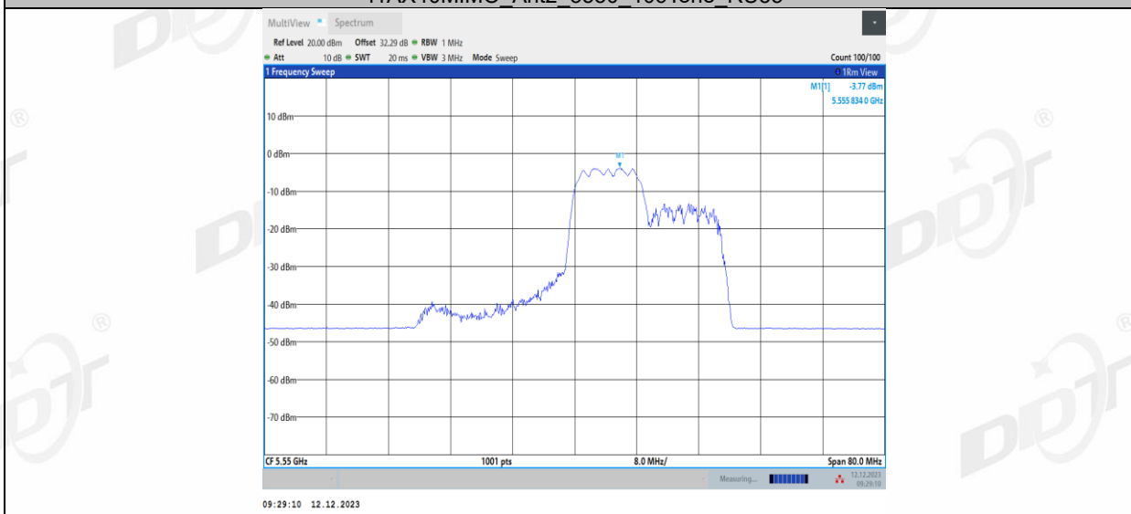
11AX40MIMO_Ant2_5550_106Tone_RU56
