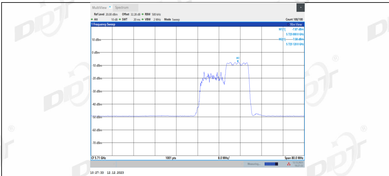
11AX40MIMO_Ant2_5710_UNII-3_242Tone_RU61
