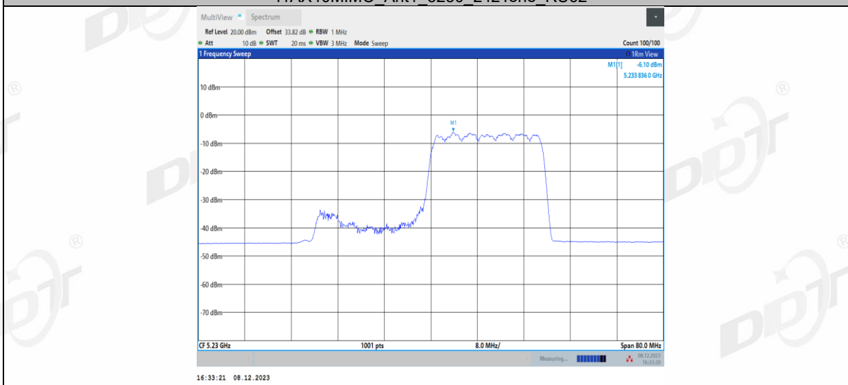
11AX40MIMO_Ant2_5230_106Tone_RU55
