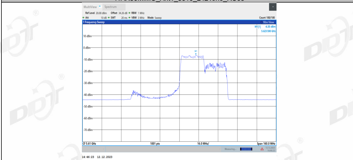
11AX80MIMO_Ant1_5610_242Tone_RU64
