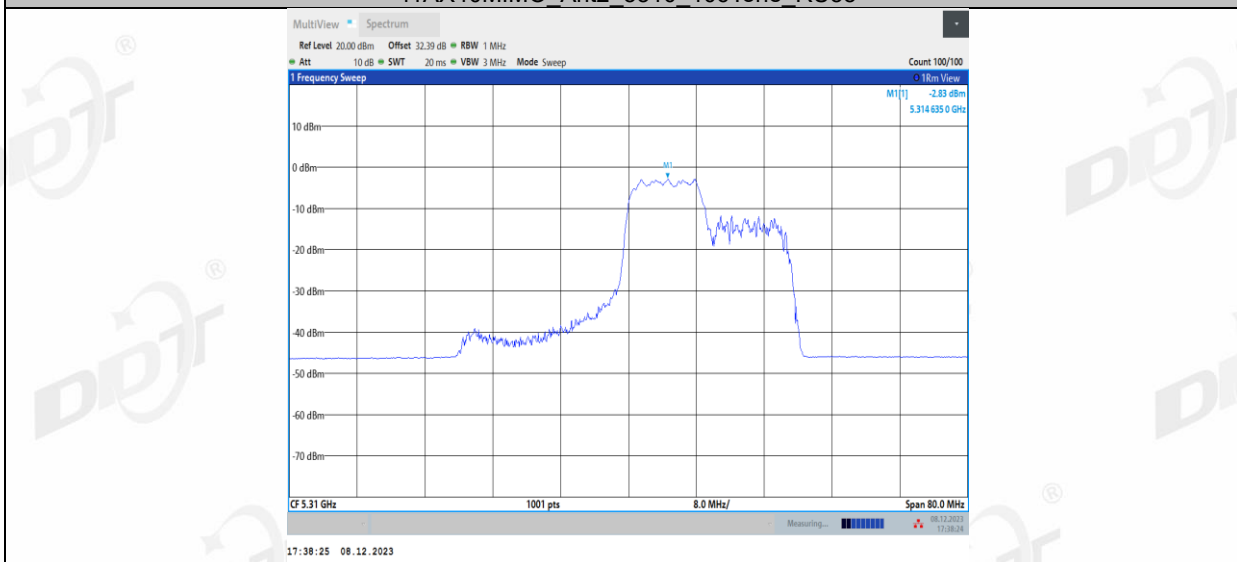
11AX40MIMO_Ant2_5310_106Tone_RU56
