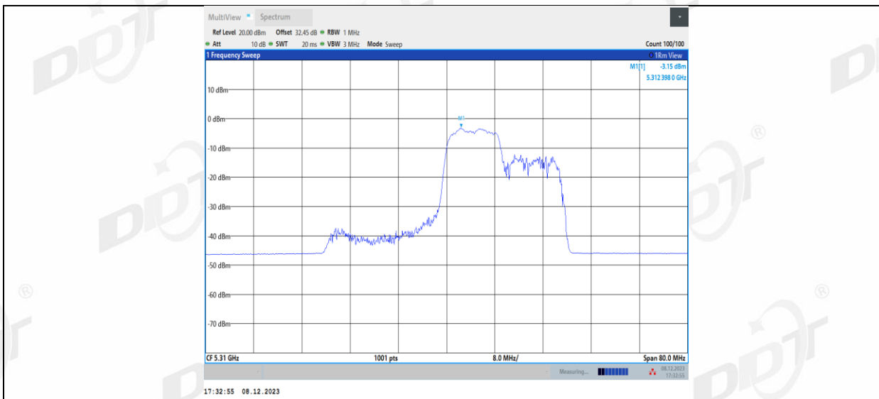
11AX40MIMO_Ant1_5310_106Tone_RU56
