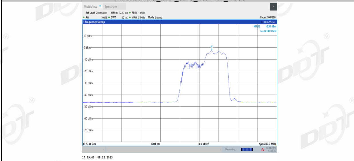
11AX40MIMO_Ant2_5310_242Tone_RU61
