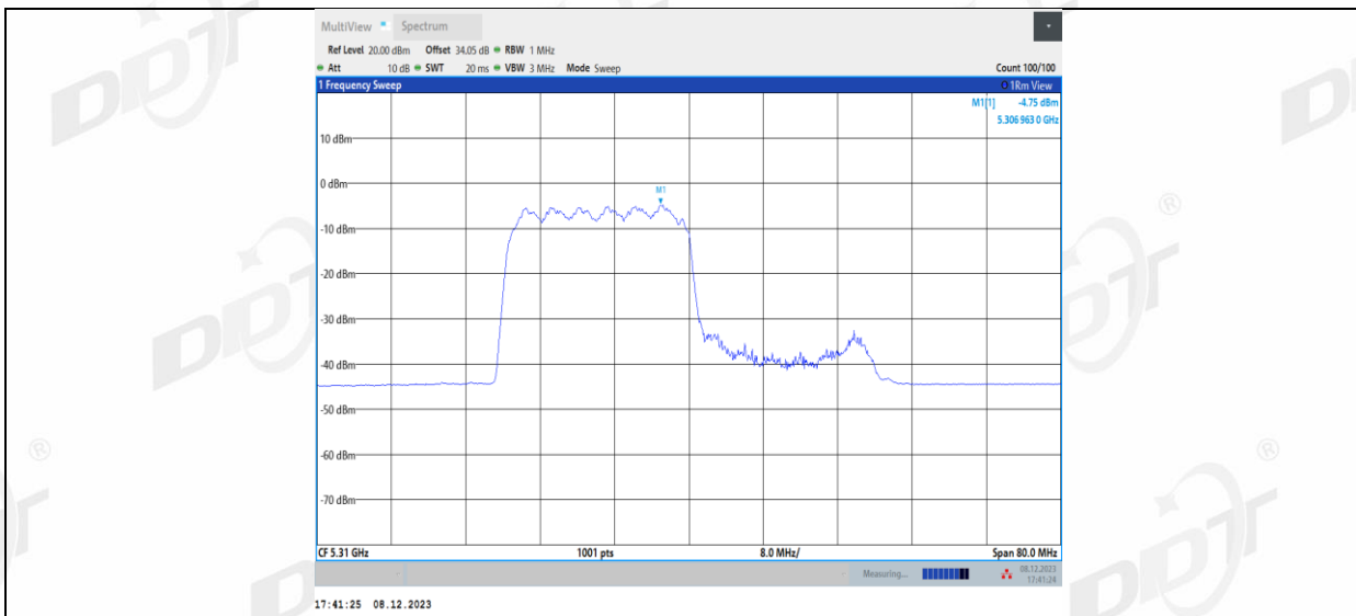
11AX40MIMO_Ant2_5310_242Tone_RU62
