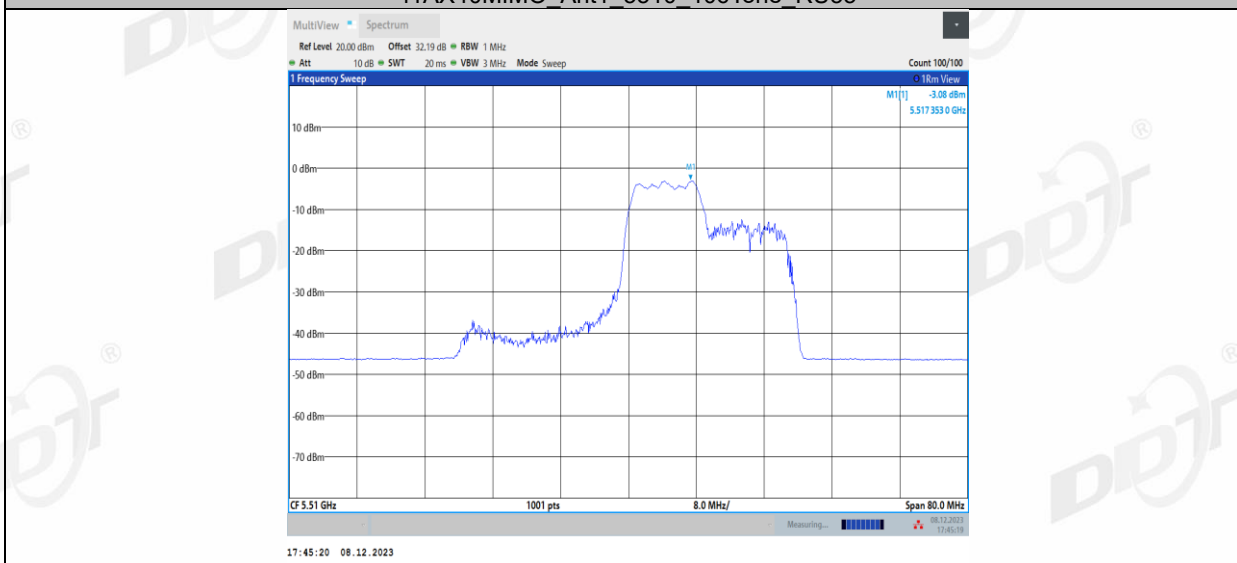
11AX40MIMO_Ant1_5510_106Tone_RU56
