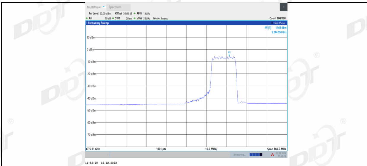
11AX80MIMO_Ant2_5210_484Tone_RU65
