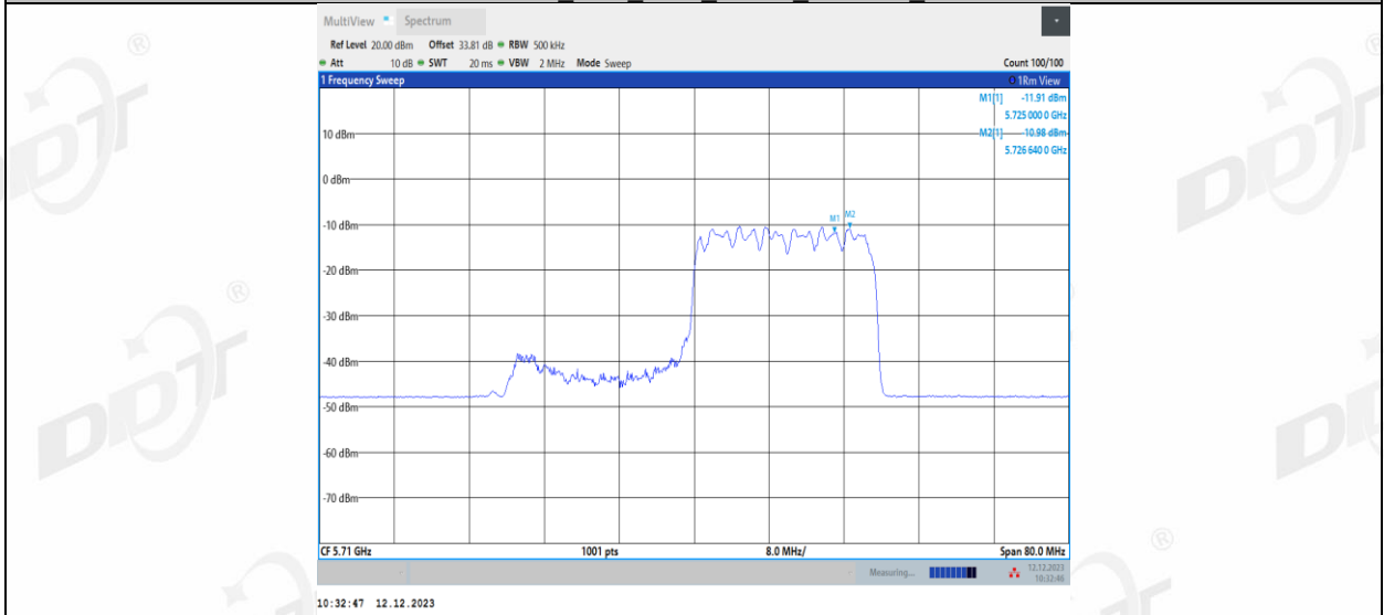
11AX40MIMO_Ant2_5710_UNII-3_106Tone_RU55
