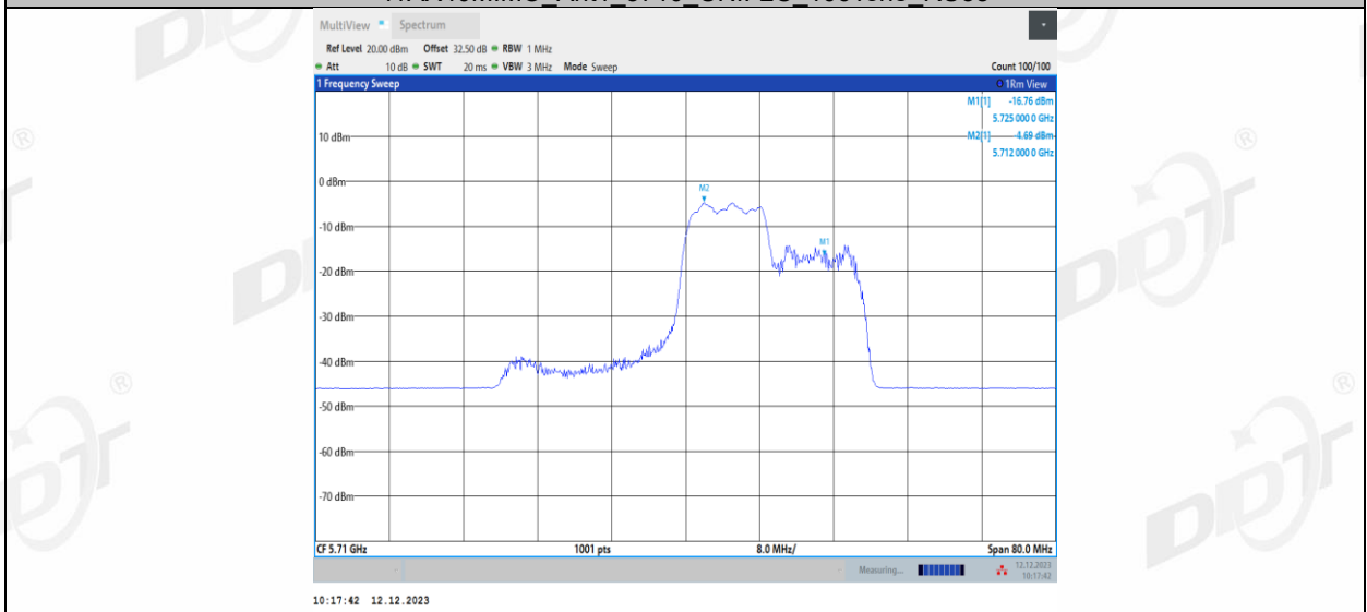
11AX40MIMO_Ant1_5710_UNII-2C_106Tone_RU56
