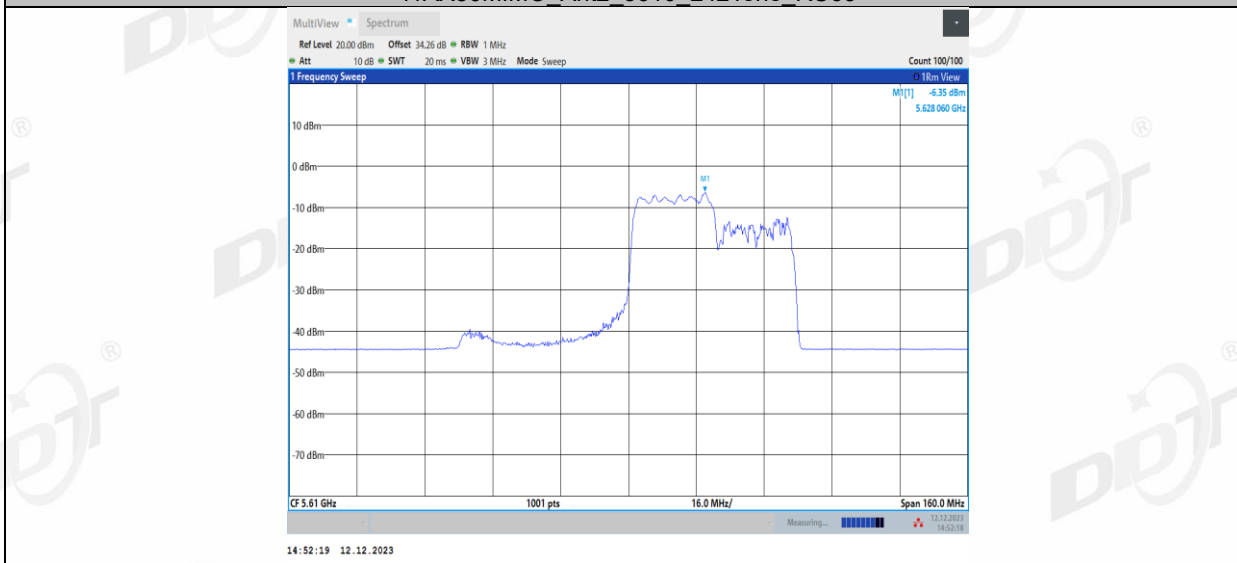
11AX80MIMO_Ant2_5610_242Tone_RU64
