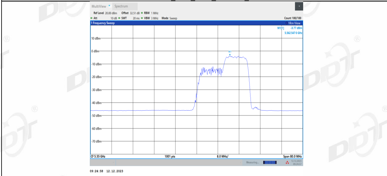
11AX40MIMO_Ant1_5550_242Tone_RU61
