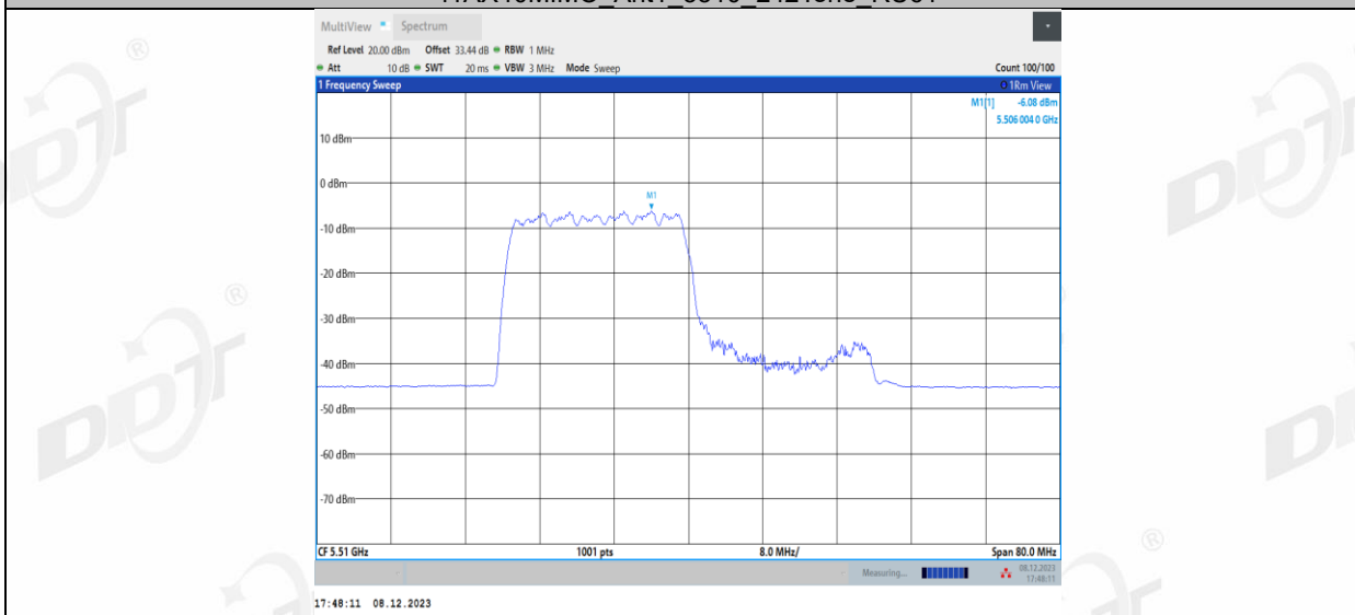
11AX40MIMO_Ant1_5510_242Tone_RU62
