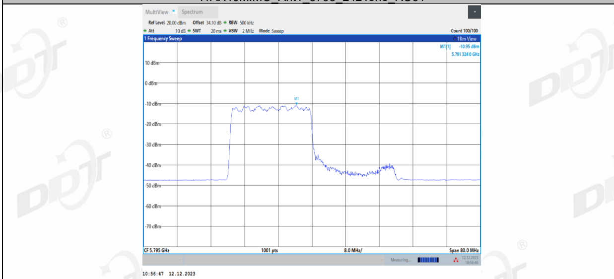
11AX40MIMO_Ant1_5795_242Tone_RU62
