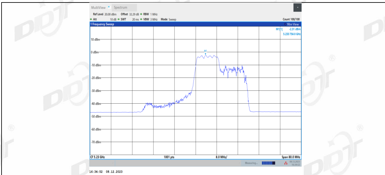
11AX40MIMO_Ant2_5230_106Tone_RU56
