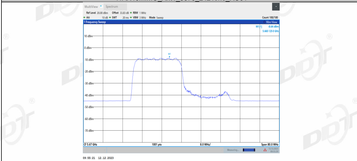
11AX40MIMO_Ant1_5670_242Tone_RU62
