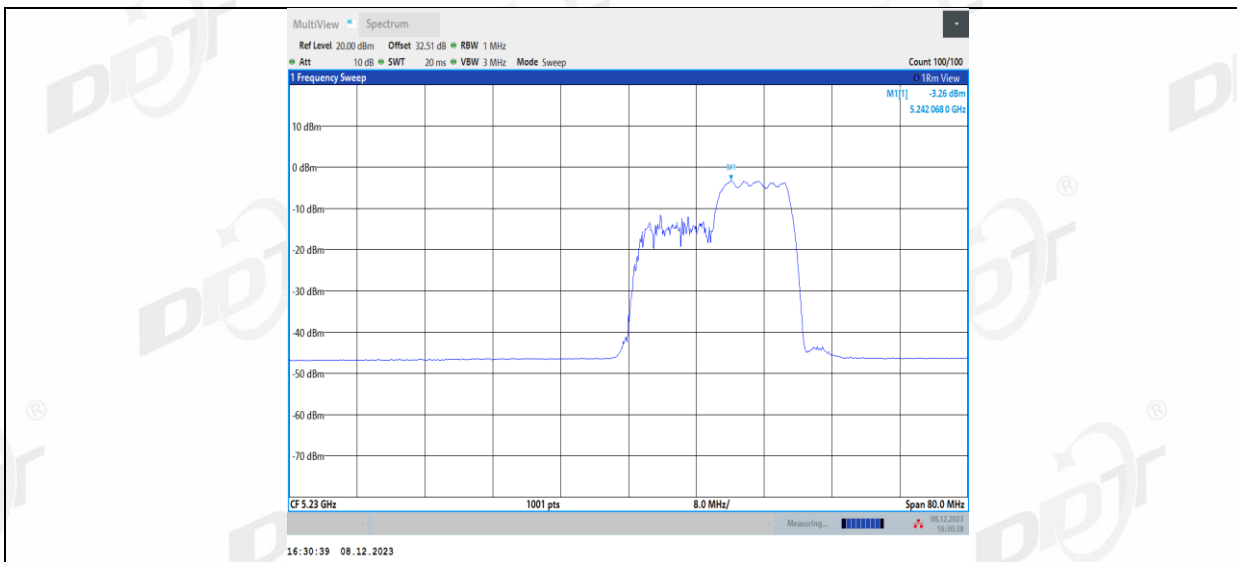
11AX40MIMO_Ant1_5230_242Tone_RU61
