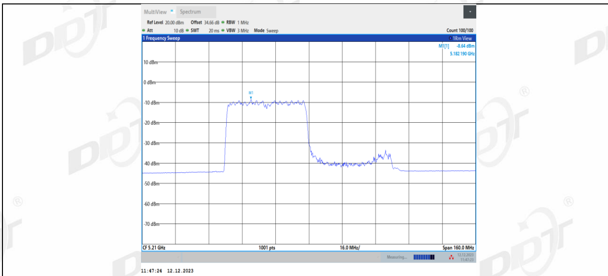
11AX80MIMO_Ant1_5210_484Tone_RU66
