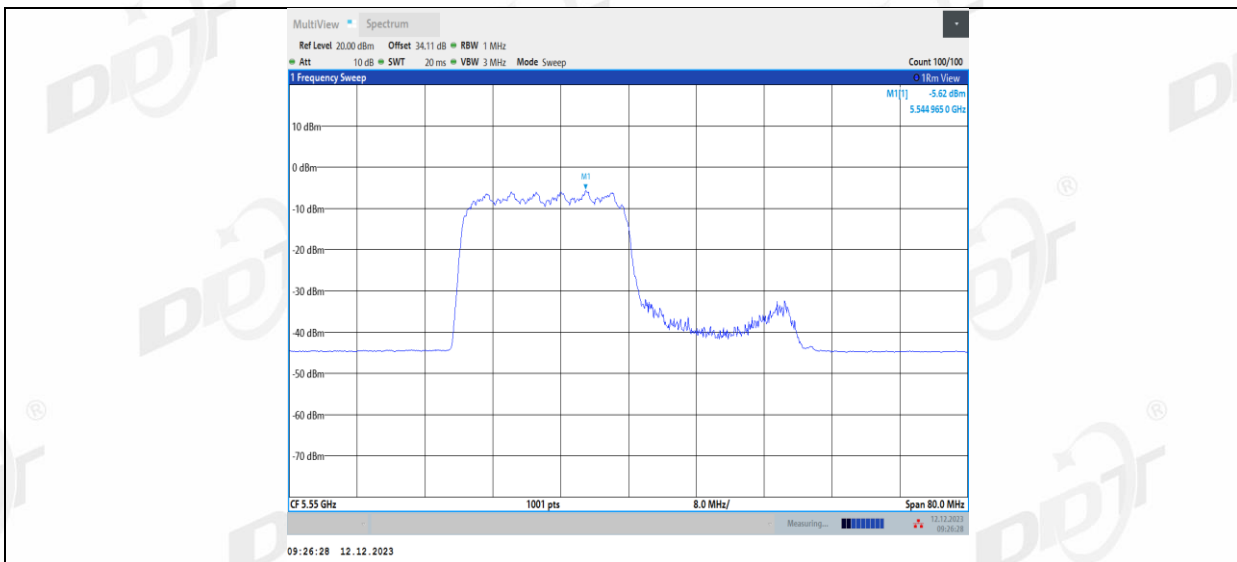
11AX40MIMO_Ant1_5550_242Tone_RU62
