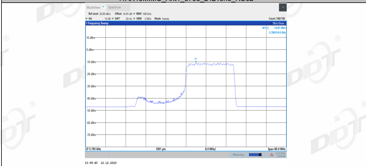
11AX40MIMO_Ant2_5795_106Tone_RU55
