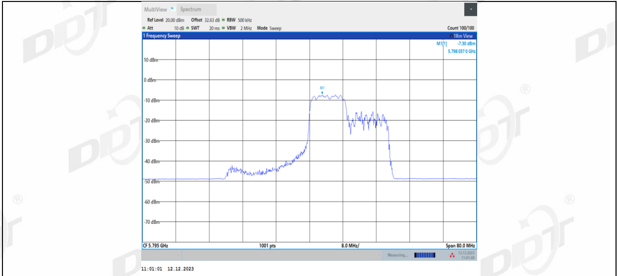
11AX40MIMO_Ant2_5795_106Tone_RU56
