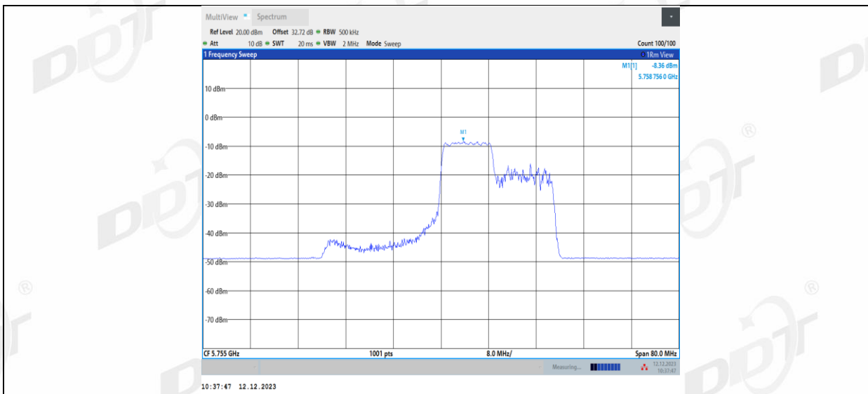
11AX40MIMO_Ant1_5755_106Tone_RU56
