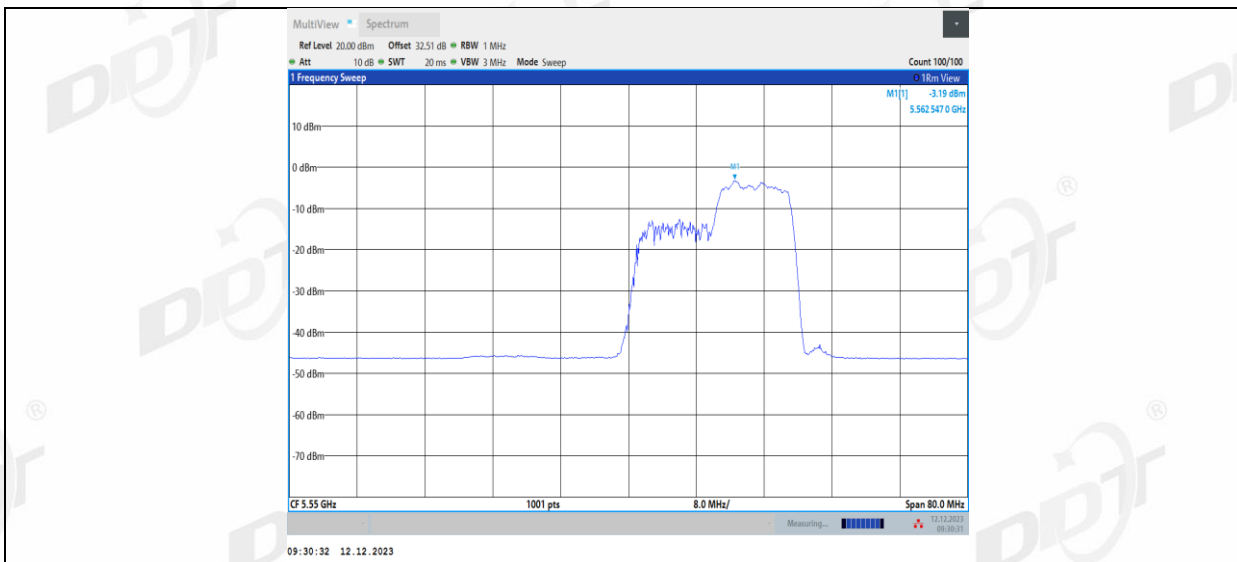
11AX40MIMO_Ant2_5550_242Tone_RU61
