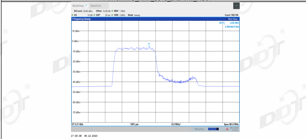
11AX40MIMO_Ant1_5310_242Tone_RU62
