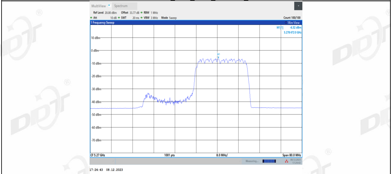
11AX40MIMO_Ant2_5270_106Tone_RU55
