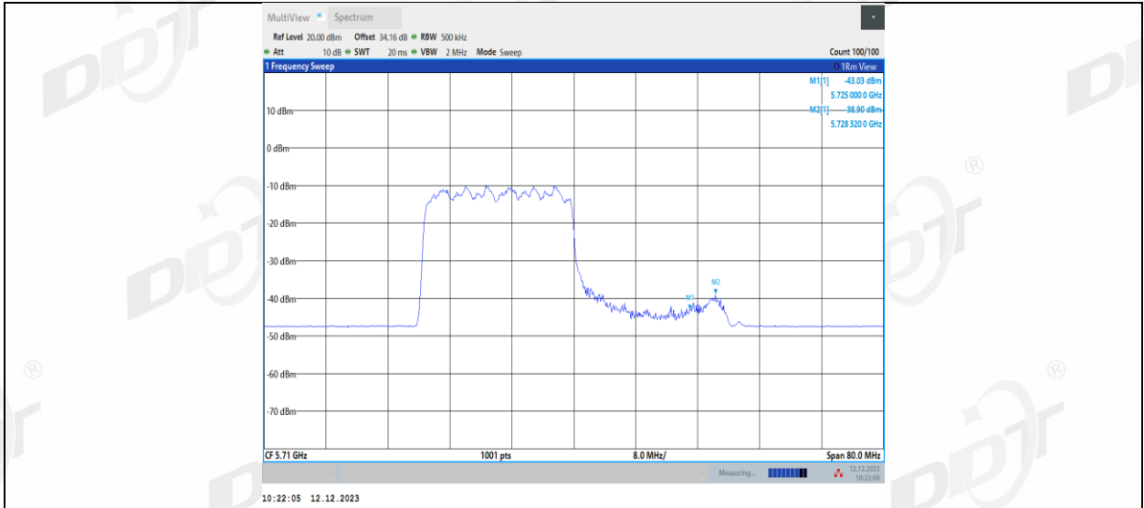
11AX40MIMO_Ant1_5710_UNII-3_242Tone_RU62
