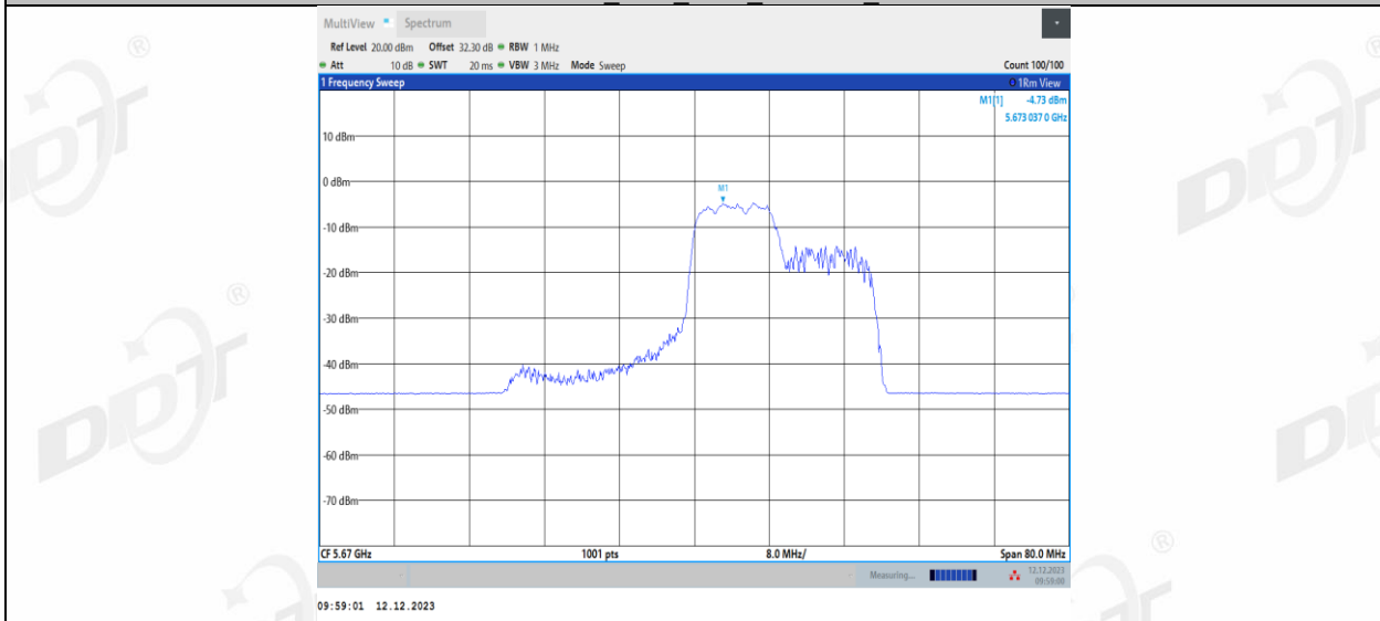
11AX40MIMO_Ant2_5670_106Tone_RU56
