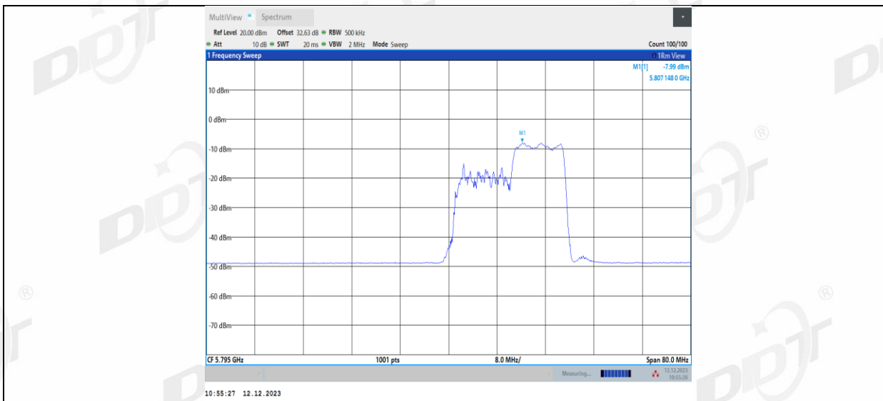
11AX40MIMO_Ant1_5795_242Tone_RU61
