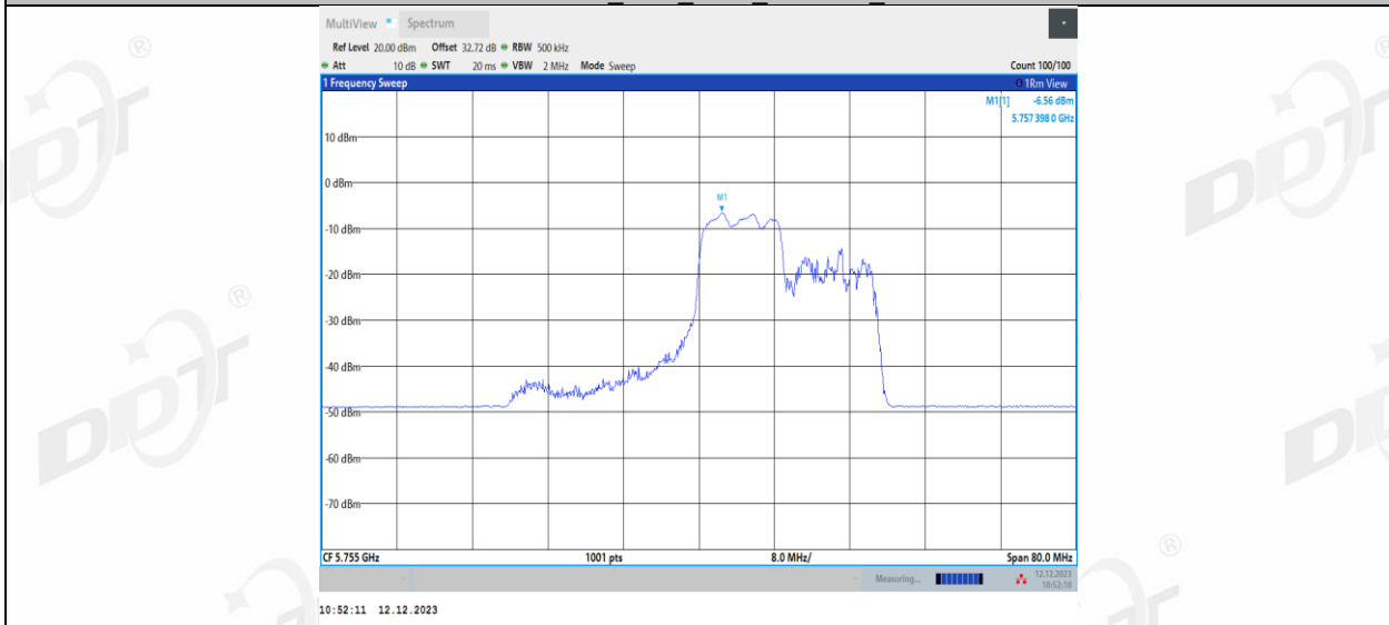
11AX40MIMO_Ant2_5755_106Tone_RU56
