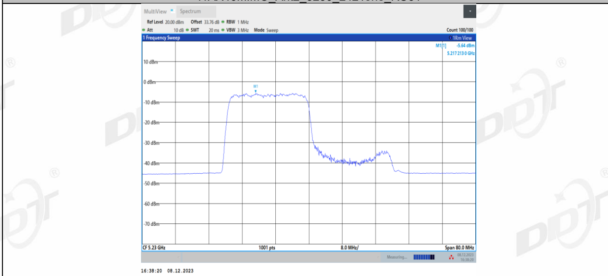
11AX40MIMO_Ant2_5230_242Tone_RU62
