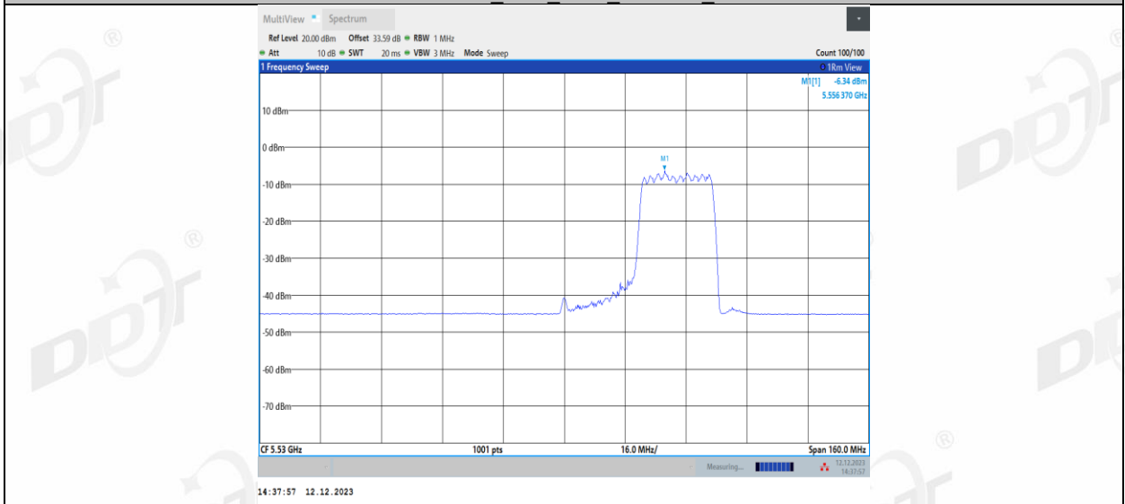
11AX80MIMO_Ant2_5530_484Tone_RU65
