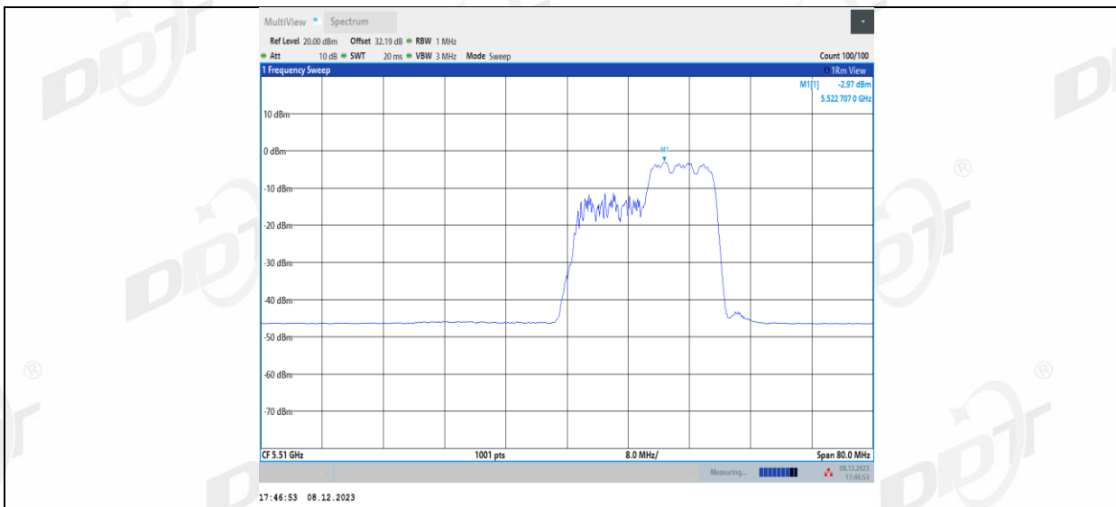
11AX40MIMO_Ant1_5510_242Tone_RU61
