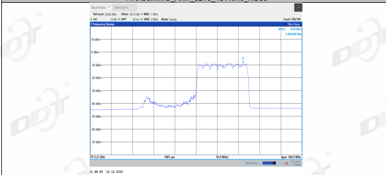
11AX80MIMO_Ant2_5210_242Tone_RU63
