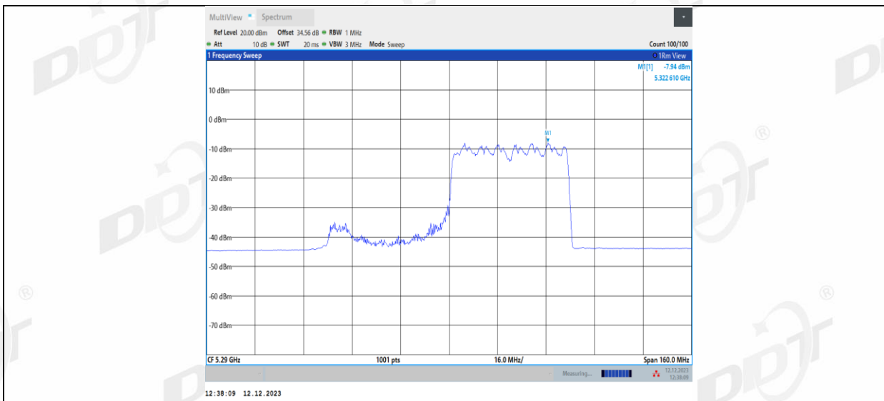
11AX80MIMO_Ant2_5290_242Tone_RU63
