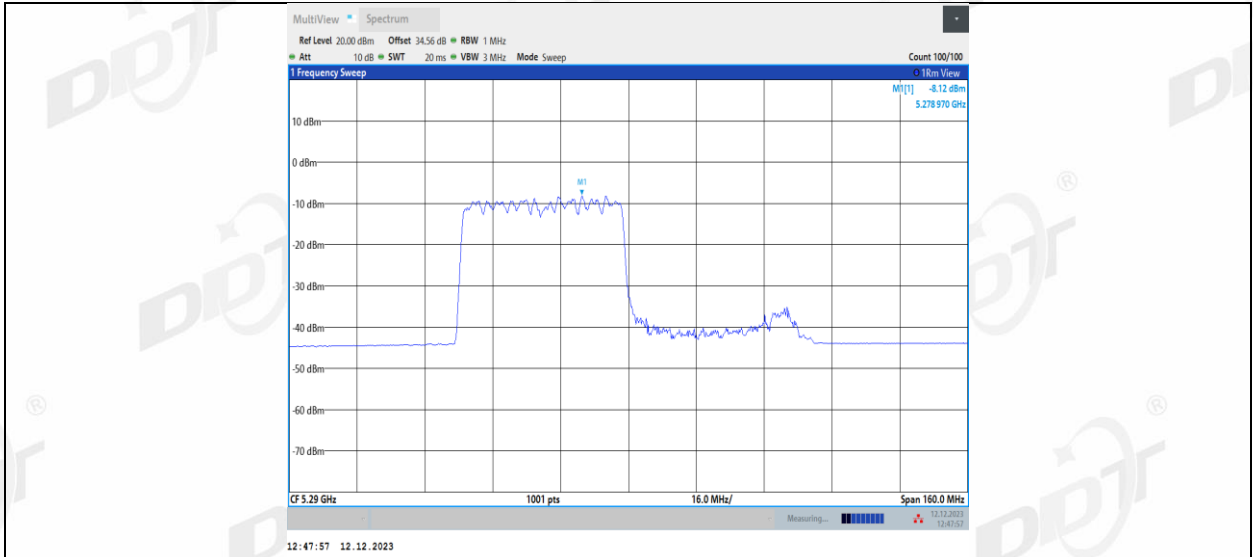
11AX80MIMO_Ant2_5290_484Tone_RU66
