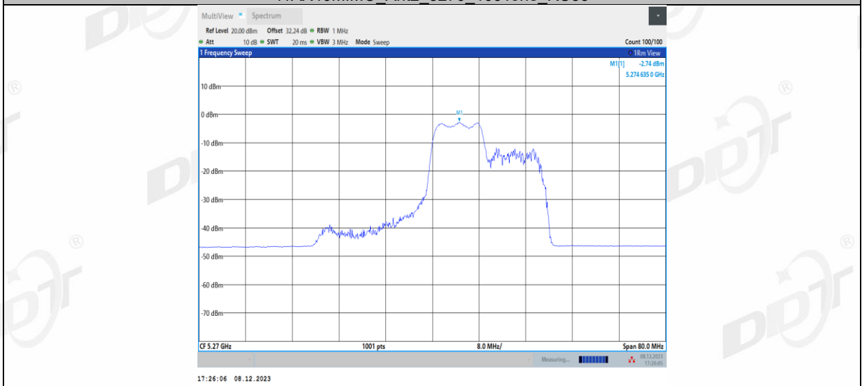
11AX40MIMO_Ant2_5270_106Tone_RU56
