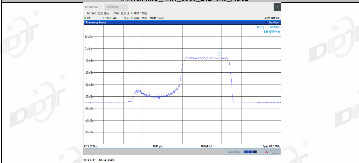
11AX40MIMO_Ant2_5550_106Tone_RU55
