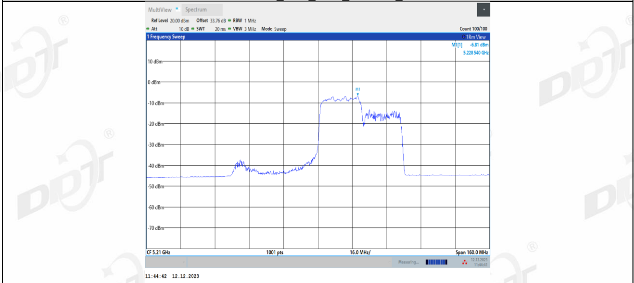
11AX80MIMO_Ant1_5210_242Tone_RU64
