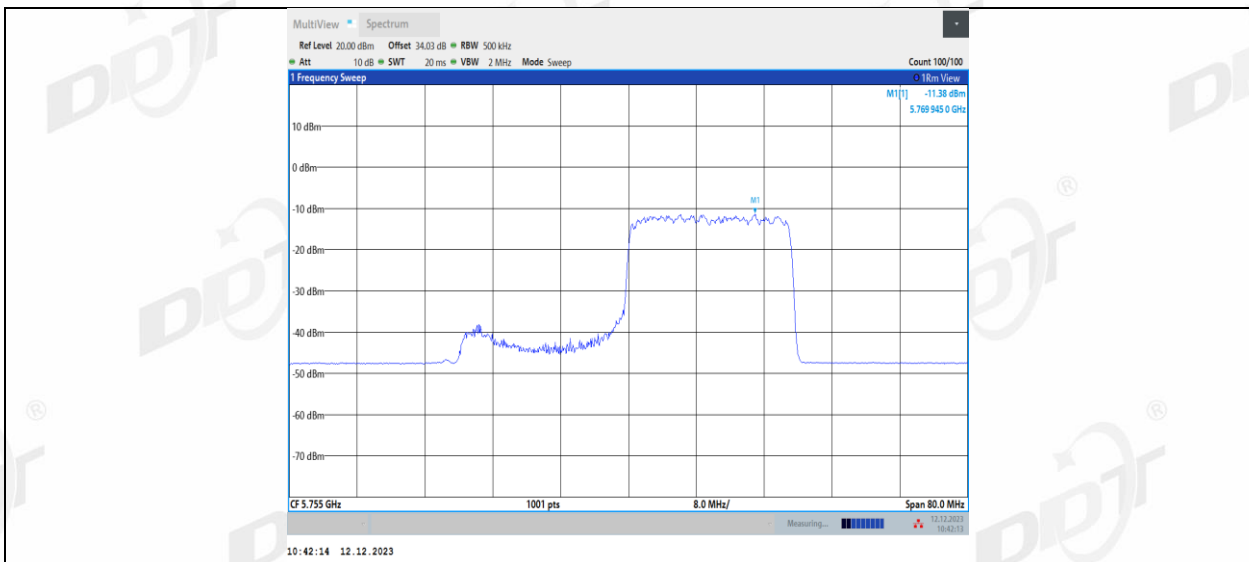
11AX40MIMO_Ant2_5755_106Tone_RU55
