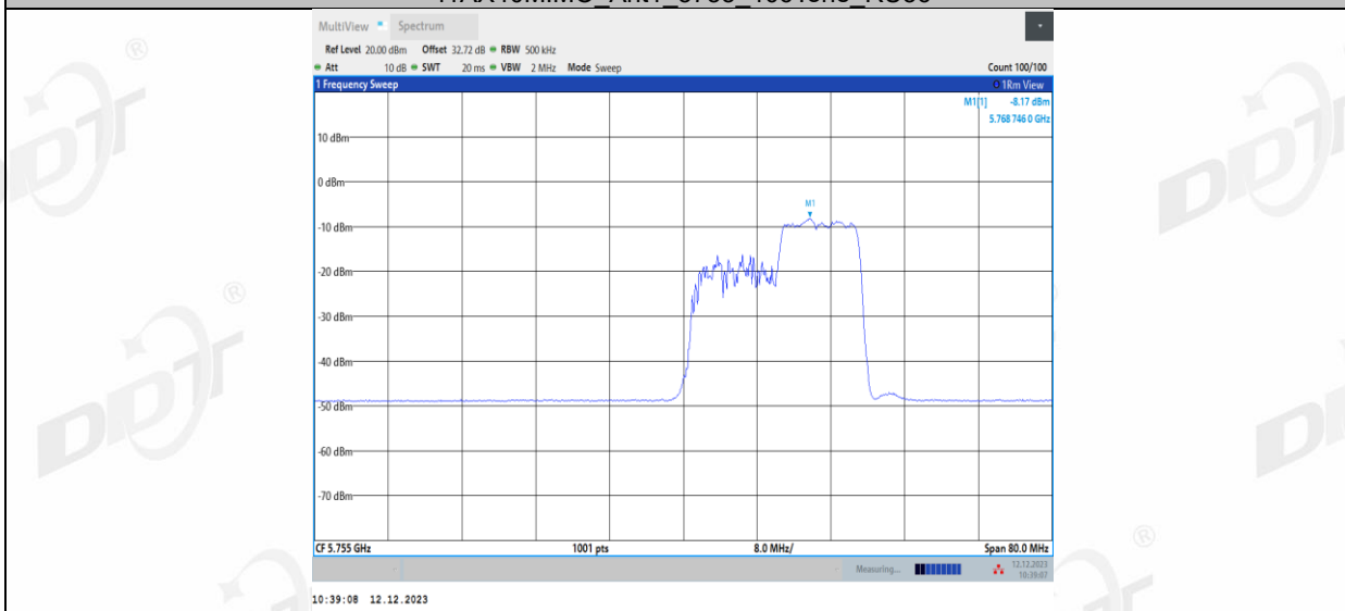
11AX40MIMO_Ant1_5755_242Tone_RU61
