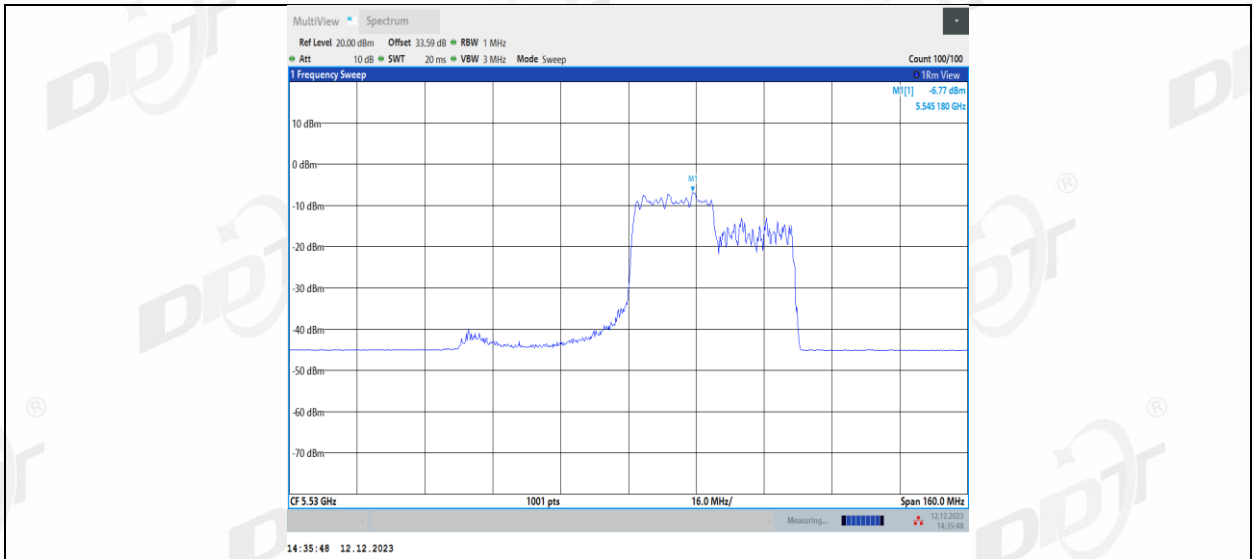
11AX80MIMO_Ant2_5530_242Tone_RU64
