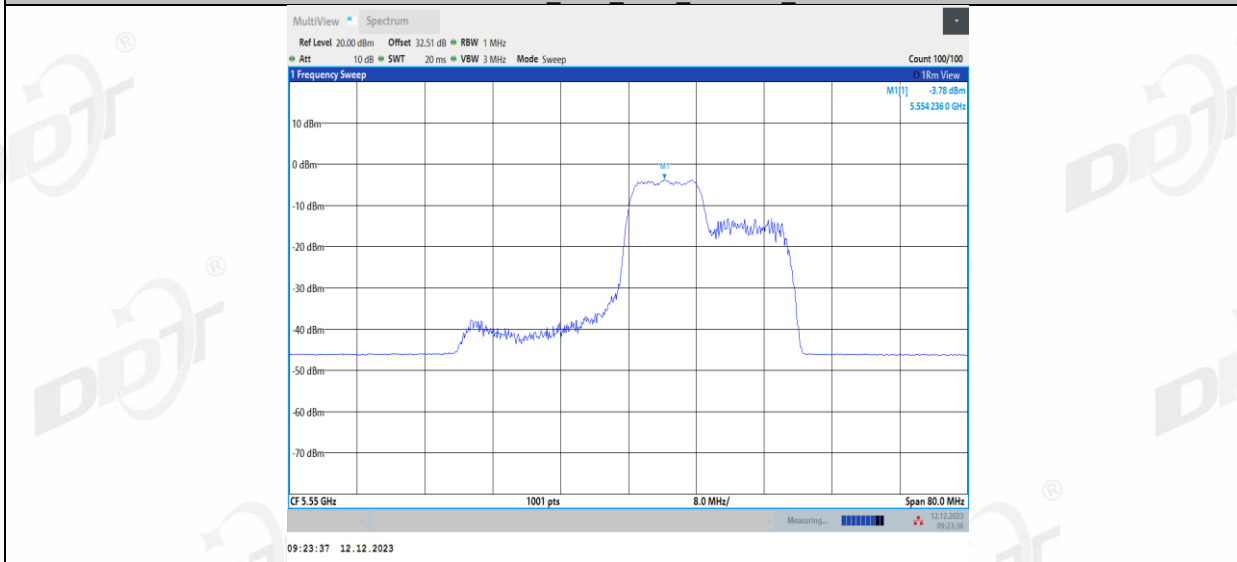
11AX40MIMO_Ant1_5550_106Tone_RU56
