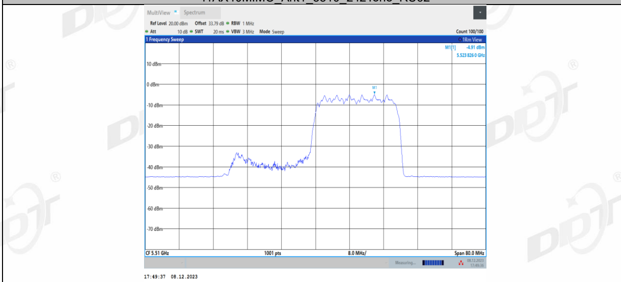
11AX40MIMO_Ant2_5510_106Tone_RU55
