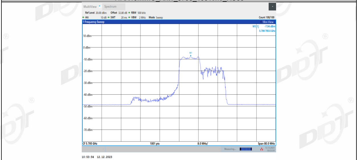
11AX40MIMO_Ant1_5795_106Tone_RU56
