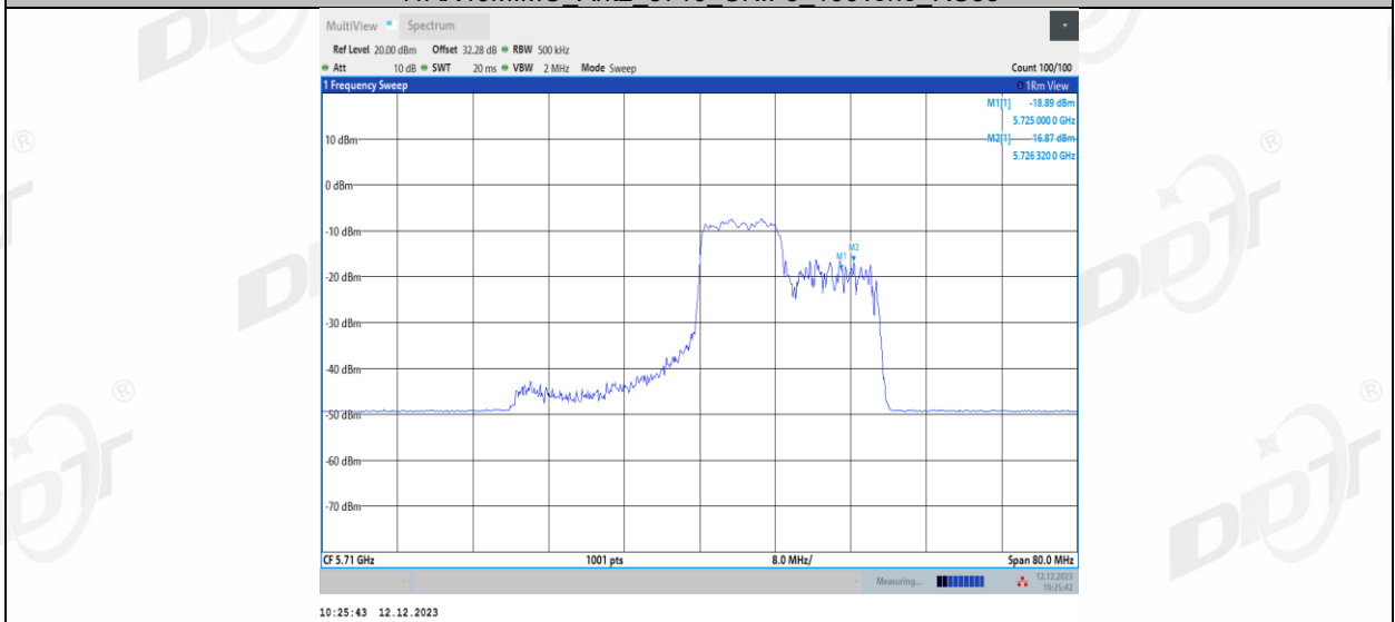
11AX40MIMO_Ant2_5710_UNII-3_106Tone_RU56
