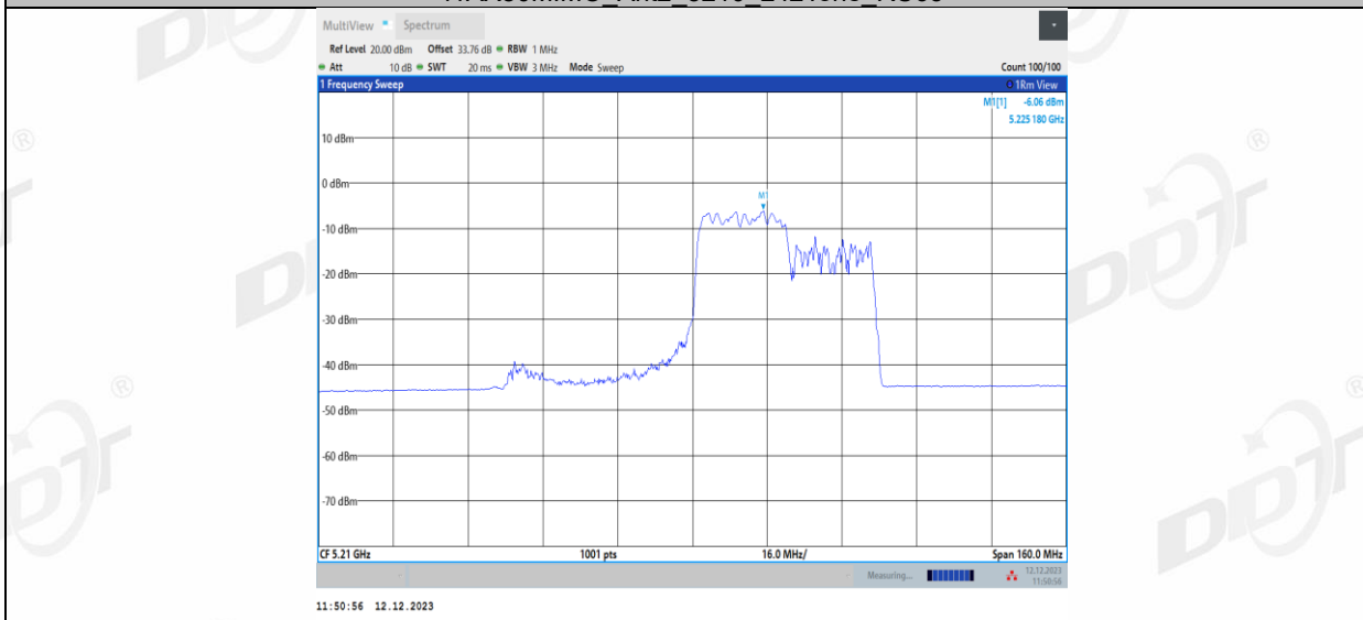
11AX80MIMO_Ant2_5210_242Tone_RU64
