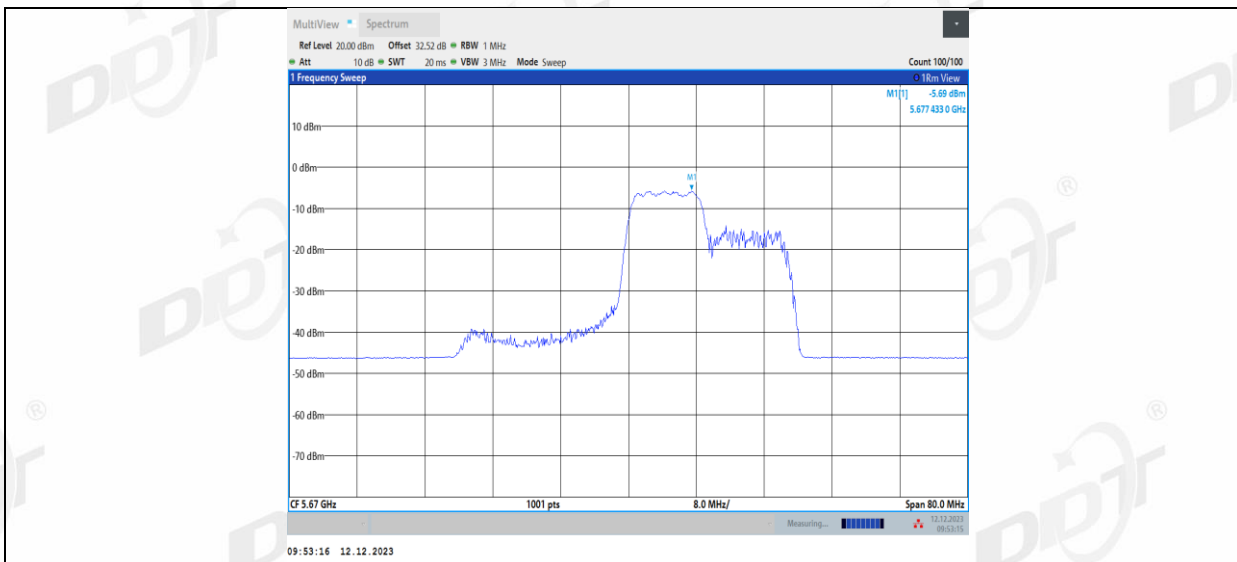
11AX40MIMO_Ant1_5670_106Tone_RU56
