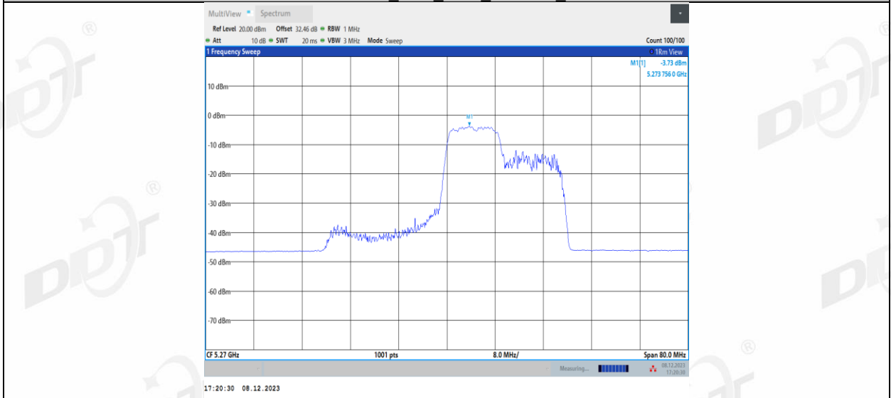
11AX40MIMO_Ant1_5270_106Tone_RU56
