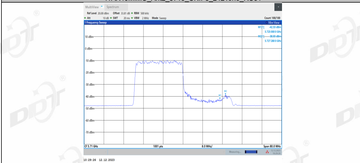
11AX40MIMO_Ant2_5710_UNII-3_242Tone_RU62
