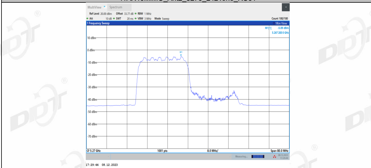
11AX40MIMO_Ant2_5270_242Tone_RU62
