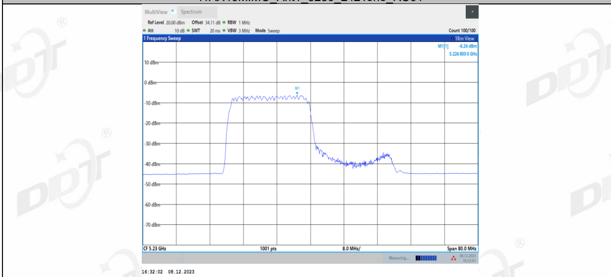
11AX40MIMO_Ant1_5230_242Tone_RU62
