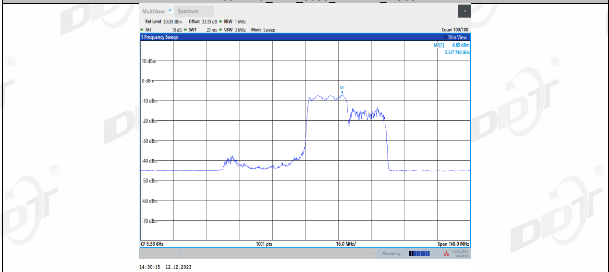
11AX80MIMO_Ant1_5530_242Tone_RU64
