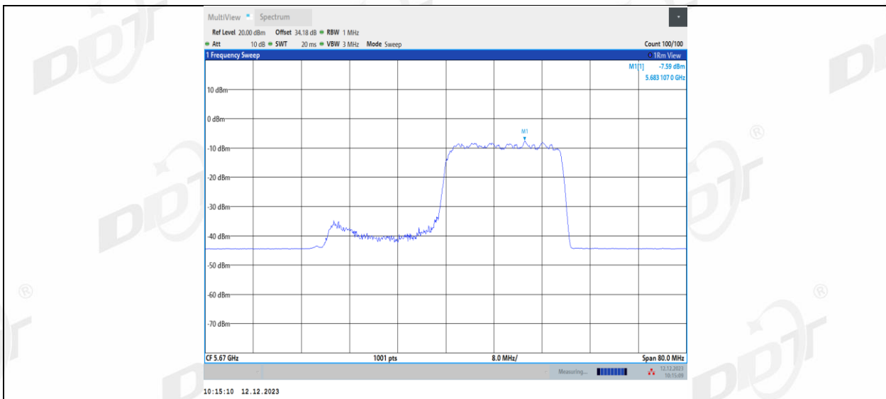
11AX40MIMO_Ant2_5670_106Tone_RU55
