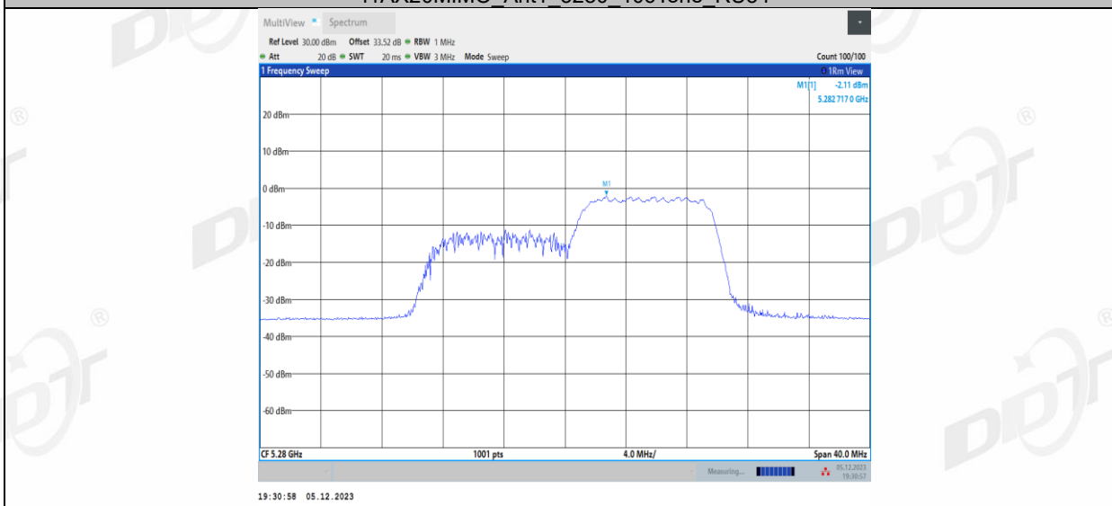
11AX20MIMO_Ant2_5280_26Tone_RU0
