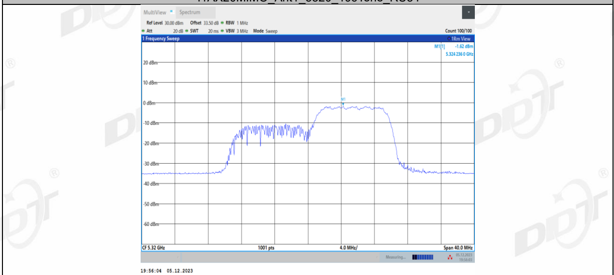
11AX20MIMO_Ant2_5320_26Tone_RU0
