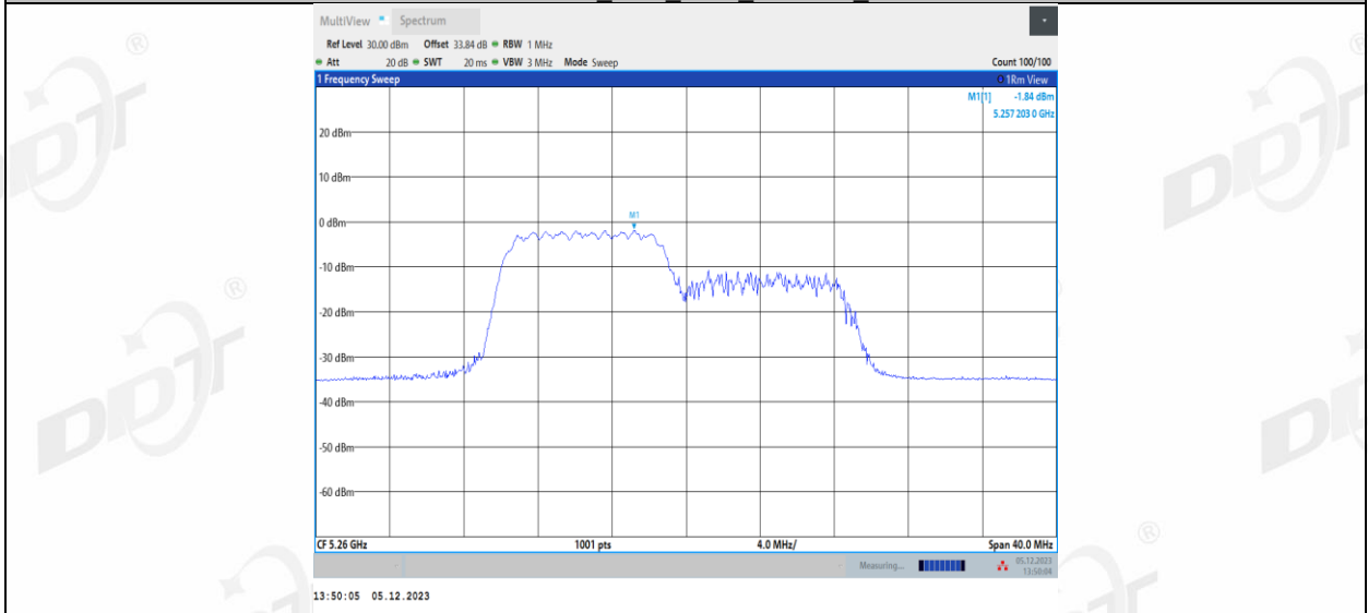
11AX20MIMO_Ant1_5260_106Tone_RU54
