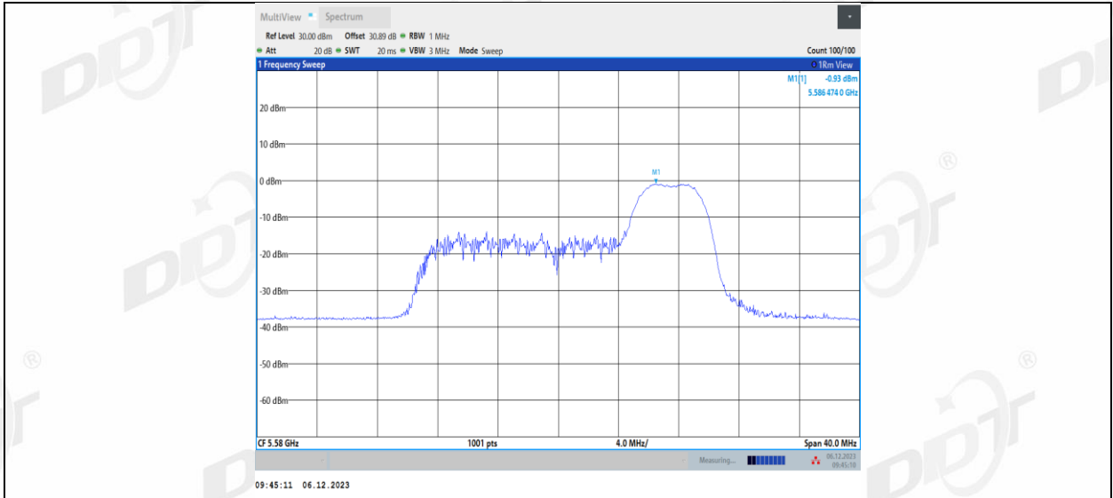
11AX20MIMO_Ant2_5580_106Tone_RU53
