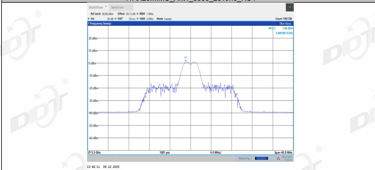
11AX20MIMO_Ant1_5500_26Tone_RU5
