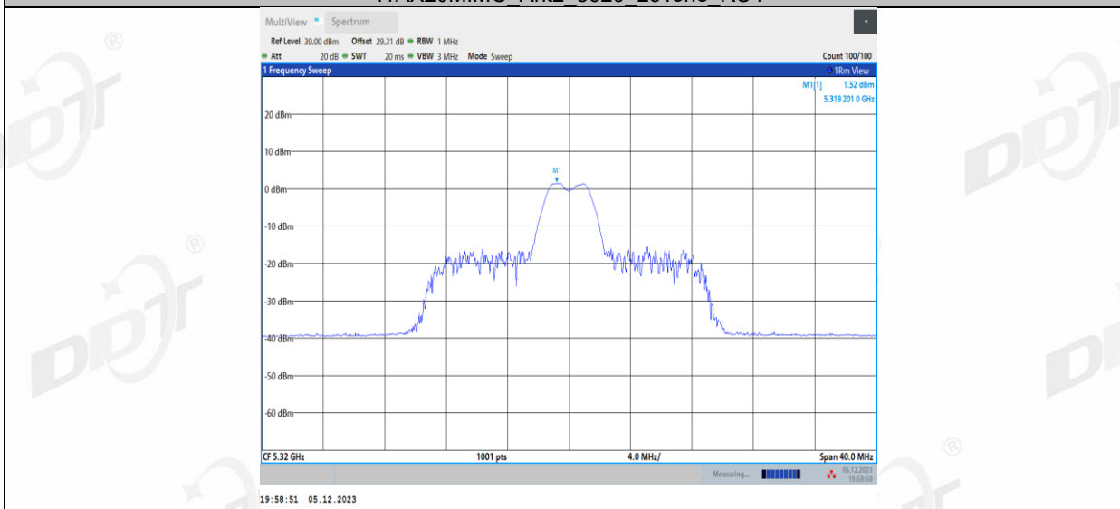
11AX20MIMO_Ant2_5320_26Tone_RU8
