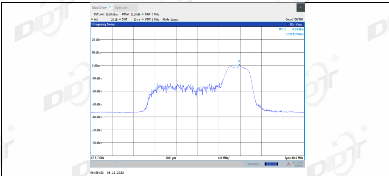
11AX20MIMO_Ant1_5700_106Tone_RU53
