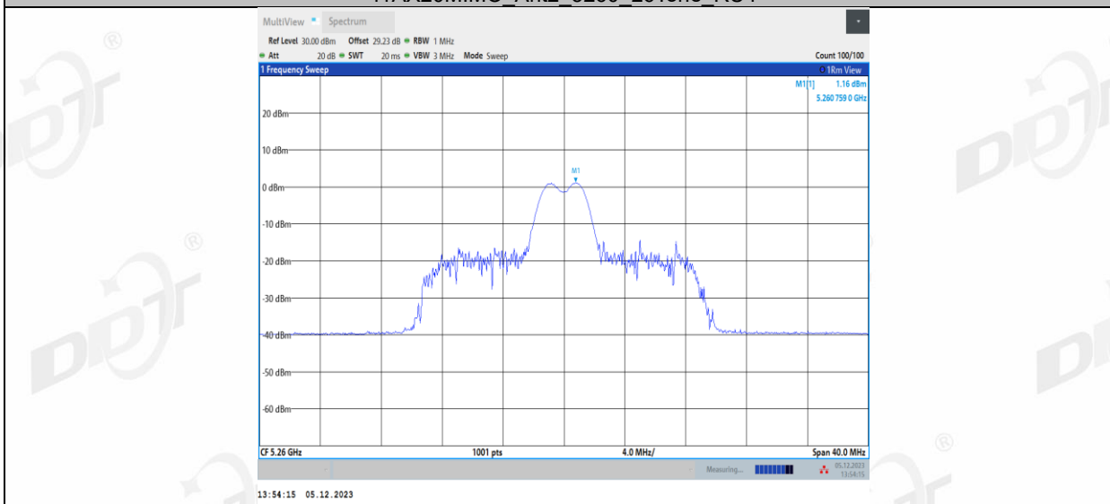
11AX20MIMO_Ant2_5260_26Tone_RU5
