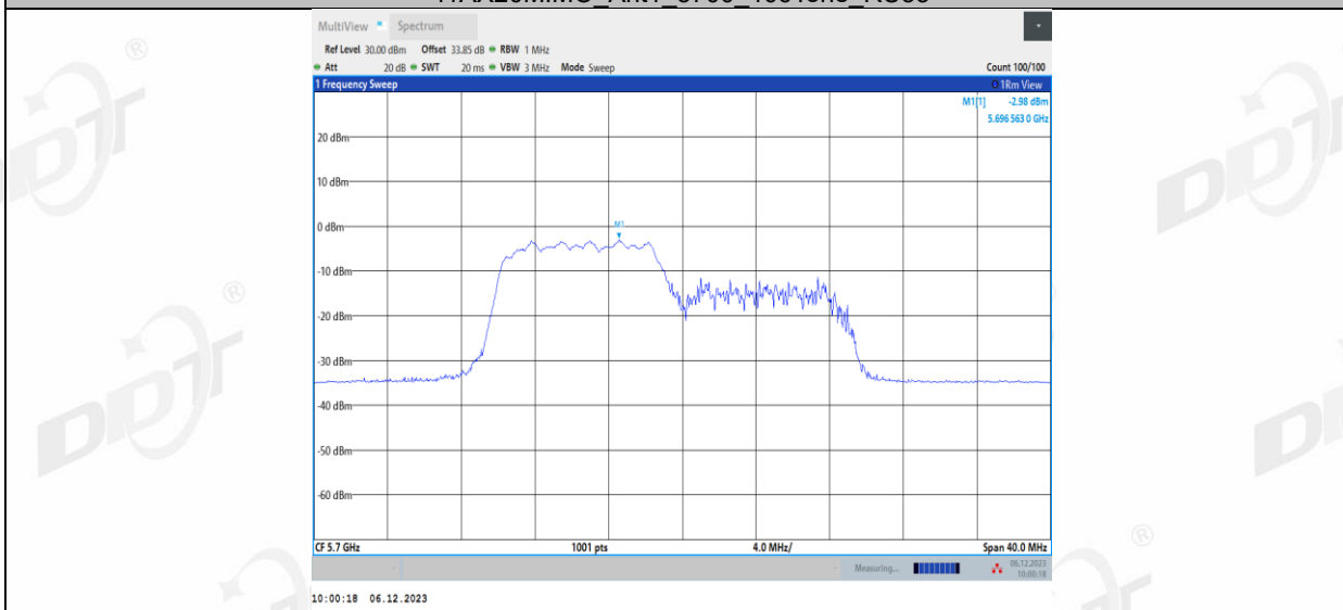
11AX20MIMO_Ant1_5700_106Tone_RU54
