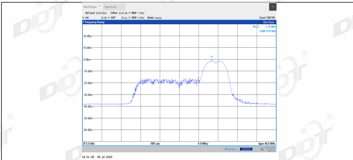
11AX20MIMO_Ant2_5500_106Tone_RU53
