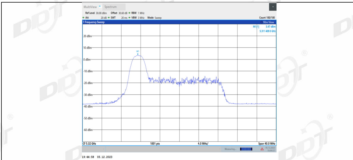
11AX20MIMO_Ant1_5320_26Tone_RU4
