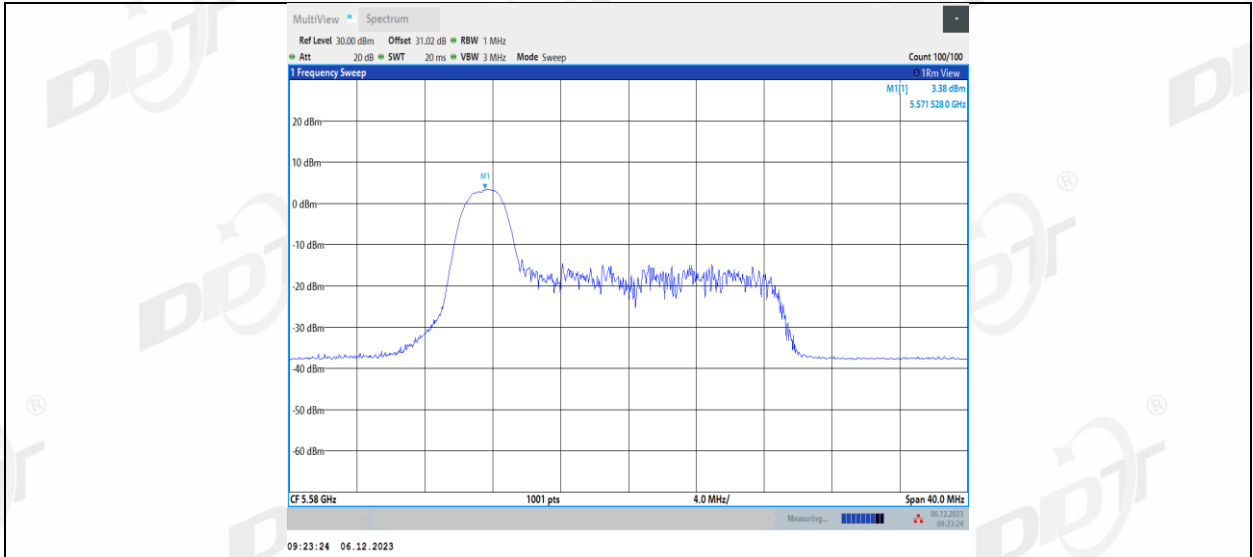
11AX20MIMO_Ant1_5580_26Tone_RU4
