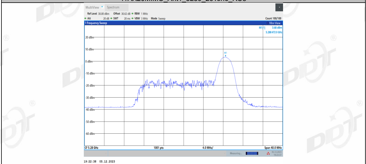
11AX20MIMO_Ant1_5280_52Tone_RU37
