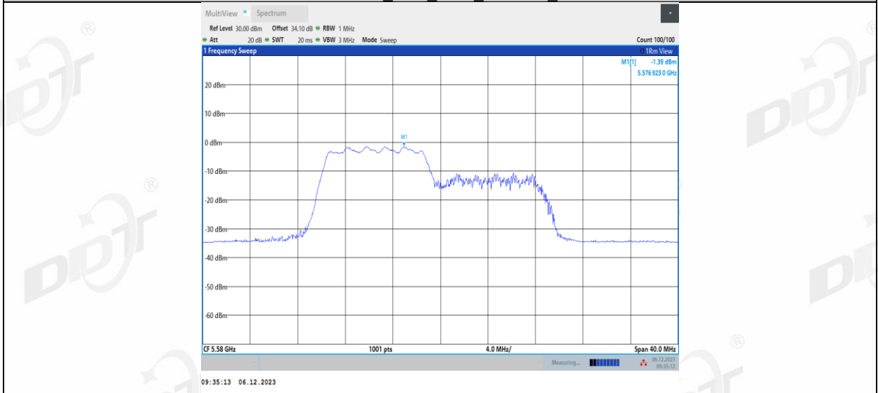
11AX20MIMO_Ant1_5580_106Tone_RU54
