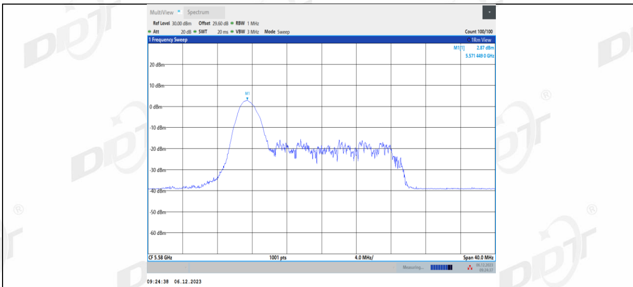
11AX20MIMO_Ant2_5580_26Tone_RU4
