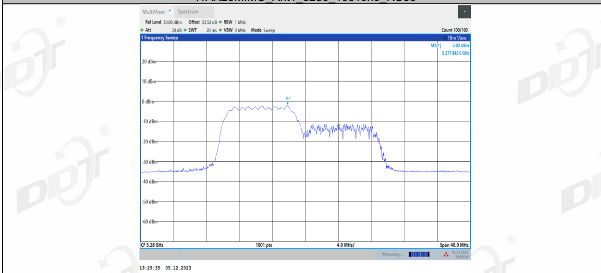
11AX20MIMO_Ant1_5280_106Tone_RU54
