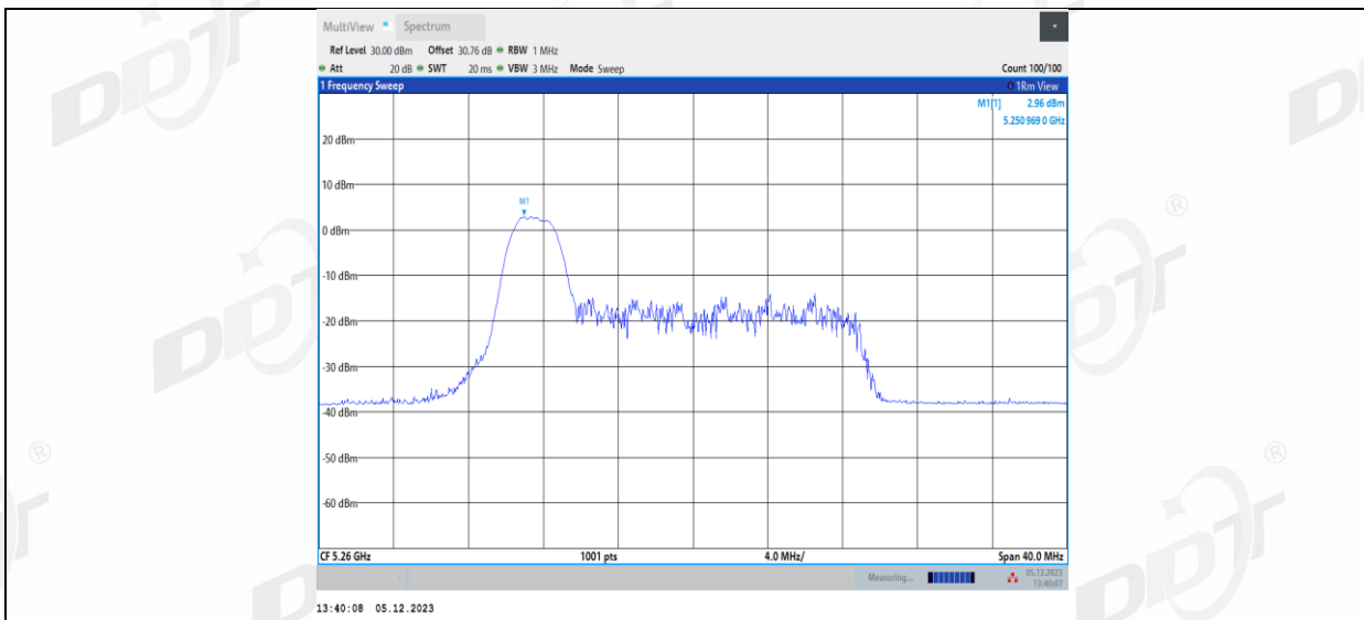
11AX20MIMO_Ant1_5260_26Tone_RU4
