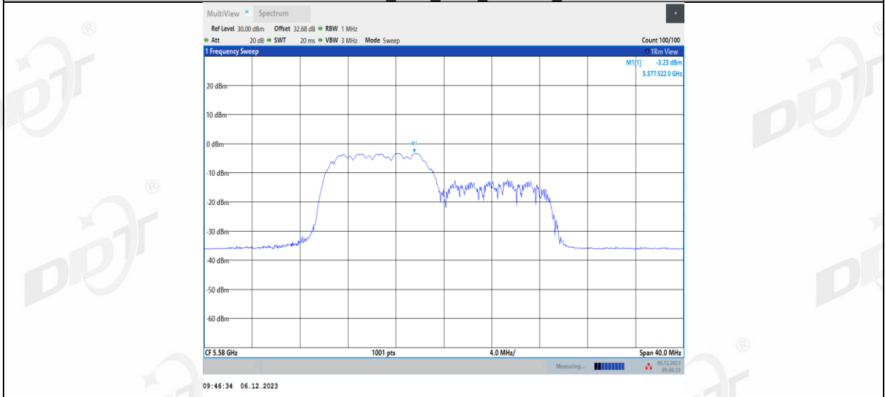
11AX20MIMO_Ant2_5580_106Tone_RU54
