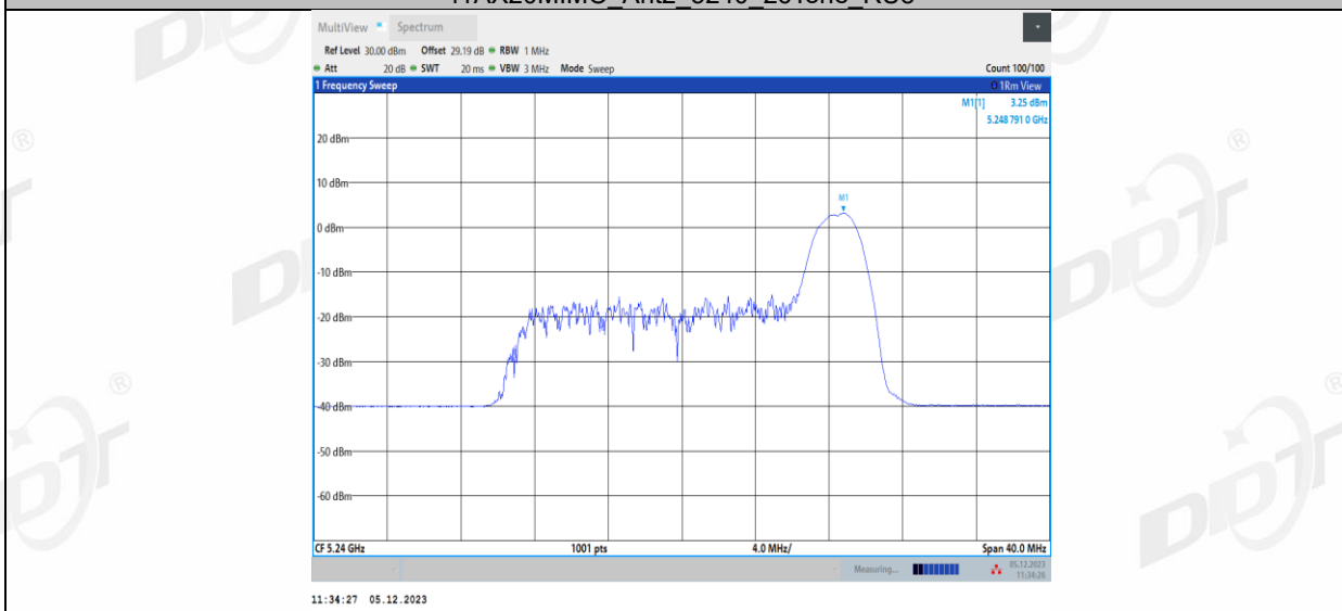
11AX20MIMO_Ant2_5240_52Tone_RU37
