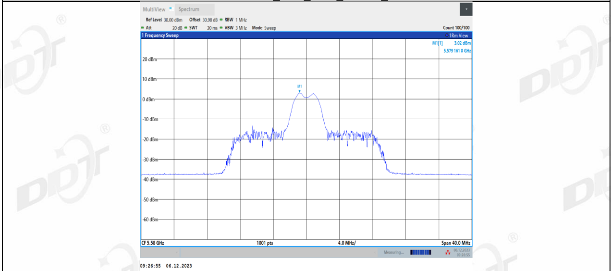
11AX20MIMO_Ant1_5580_26Tone_RU5
