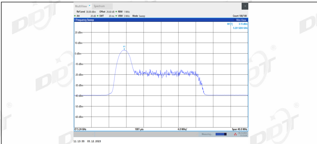
11AX20MIMO_Ant2_5240_26Tone_RU4
