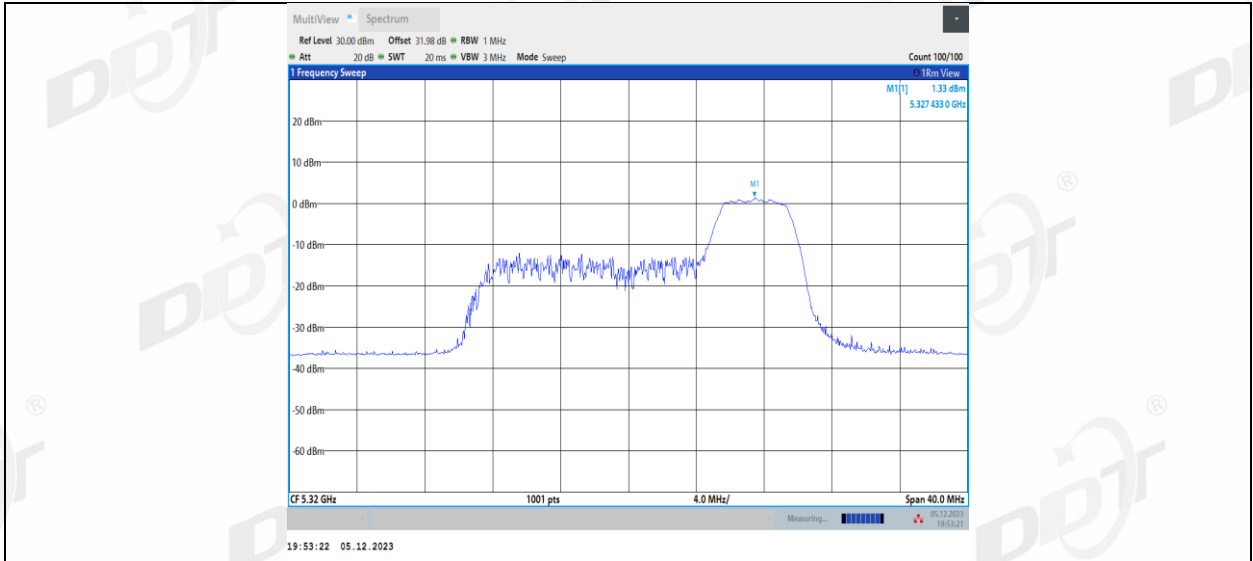
11AX20MIMO_Ant1_5320_106Tone_RU53
