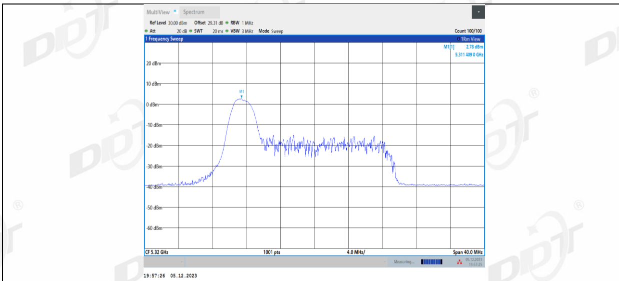
11AX20MIMO_Ant2_5320_26Tone_RU4
