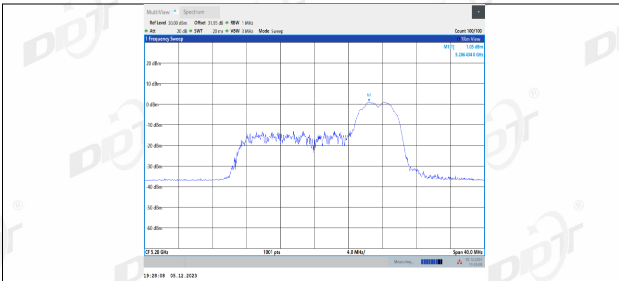
11AX20MIMO_Ant1_5280_106Tone_RU53
