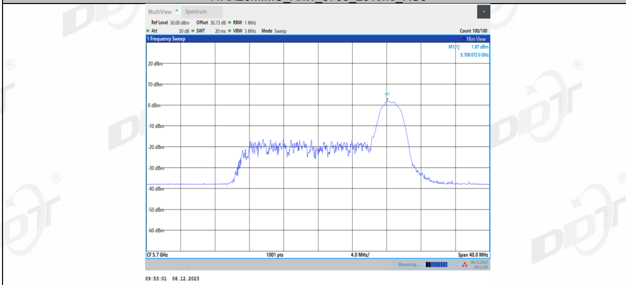
11AX20MIMO_Ant1_5700_52Tone_RU37
