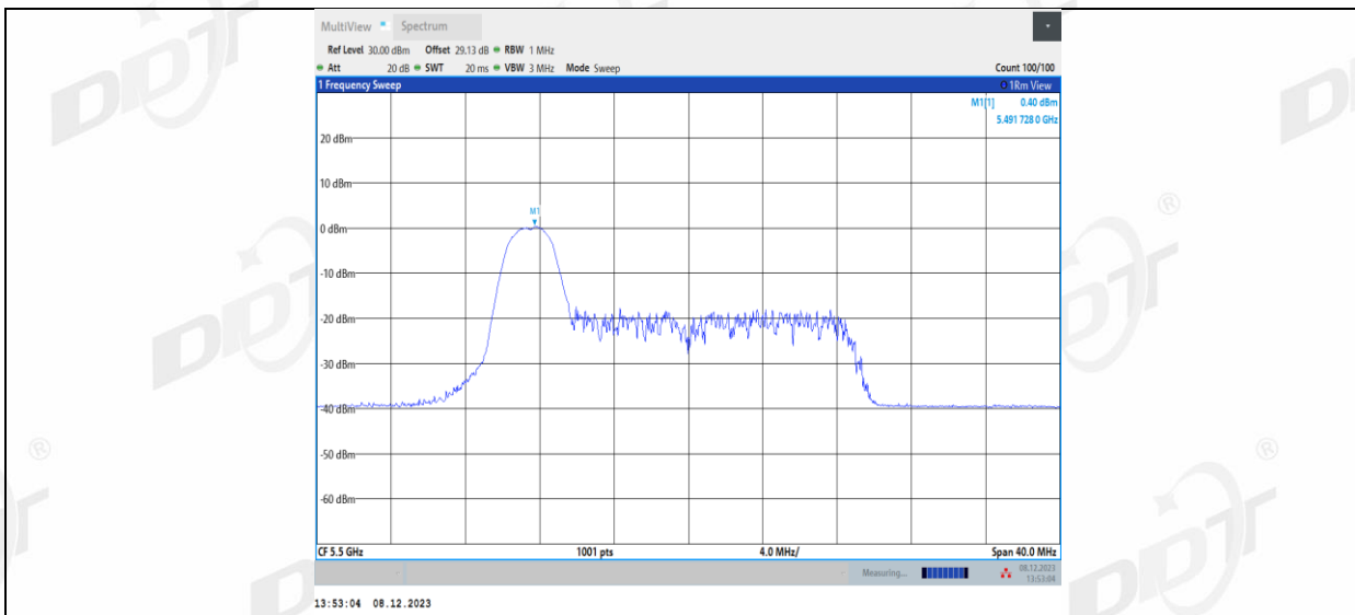
11AX20MIMO_Ant2_5500_26Tone_RU4
