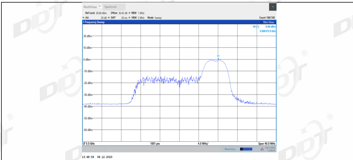
11AX20MIMO_Ant1_5500_106Tone_RU53
