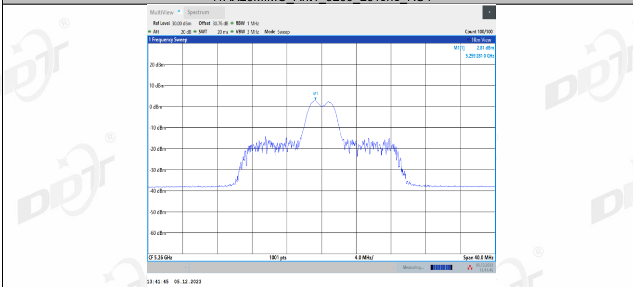
11AX20MIMO_Ant1_5260_26Tone_RU5
