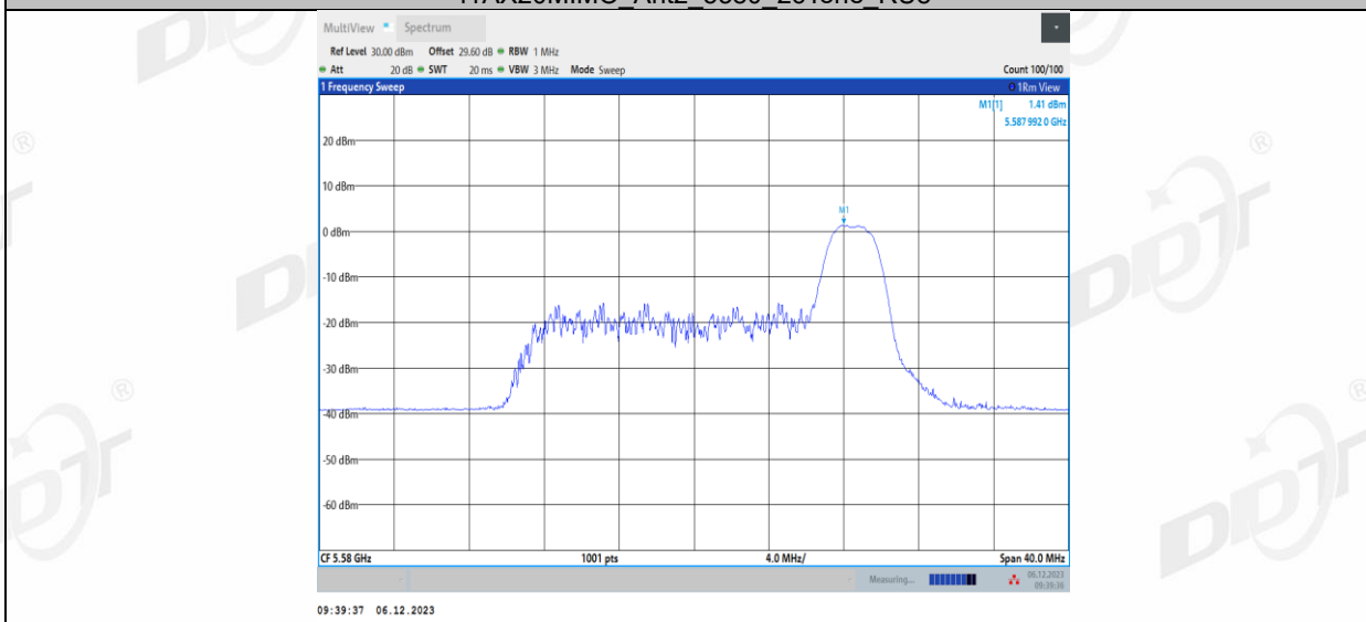
11AX20MIMO_Ant2_5580_52Tone_RU37
