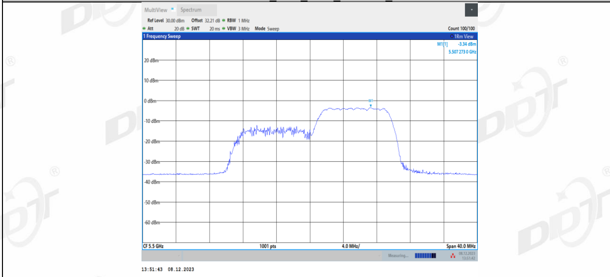
11AX20MIMO_Ant2_5500_26Tone_RU0
