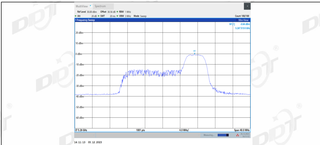
11AX20MIMO_Ant2_5260_106Tone_RU53
