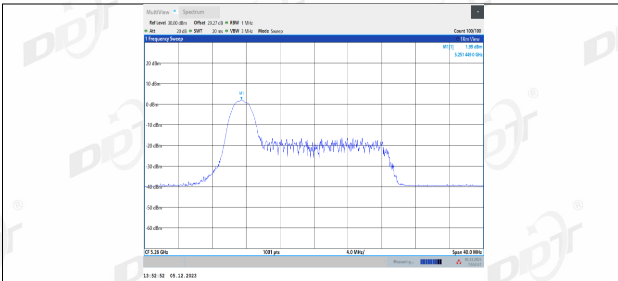
11AX20MIMO_Ant2_5260_26Tone_RU4
