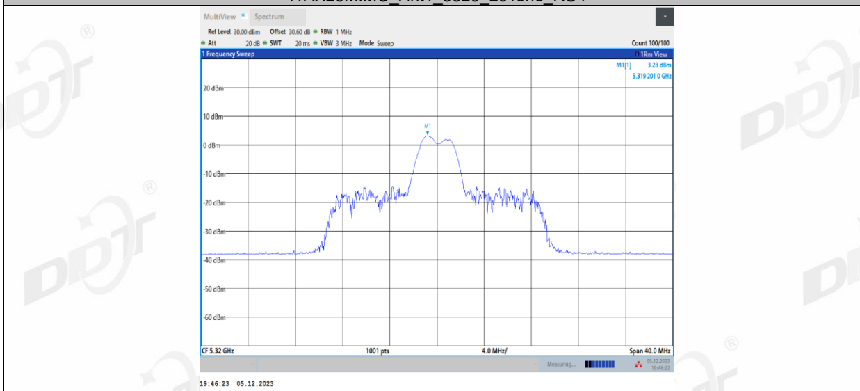
11AX20MIMO_Ant1_5320_26Tone_RU8
