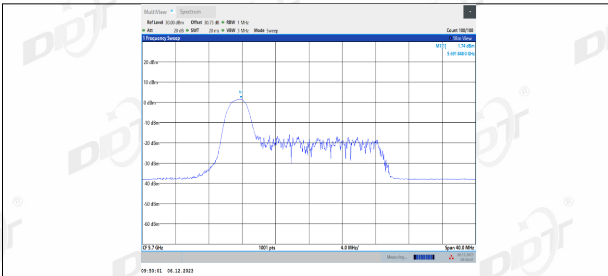
11AX20MIMO_Ant1_5700_26Tone_RU4
