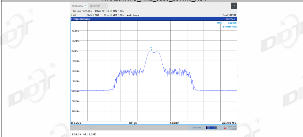
11AX20MIMO_Ant2_5500_26Tone_RU5
