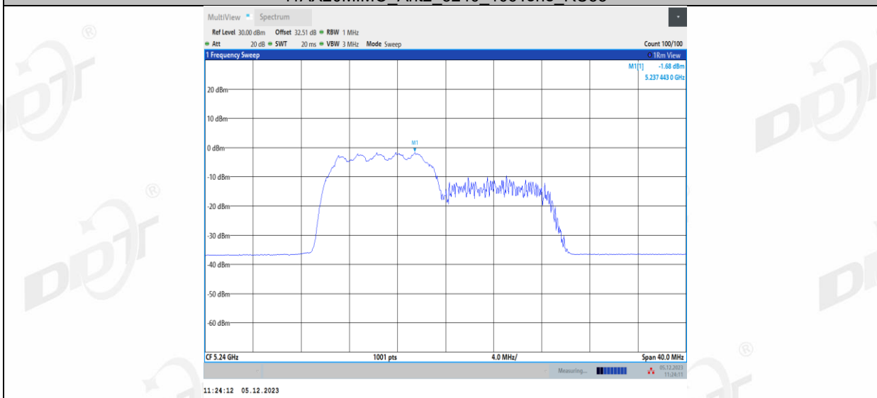
11AX20MIMO_Ant2_5240_106Tone_RU54
