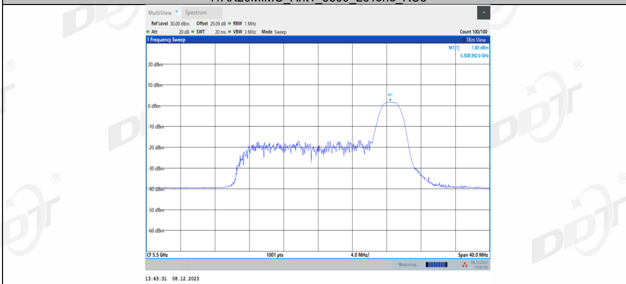
11AX20MIMO_Ant1_5500_52Tone_RU37
