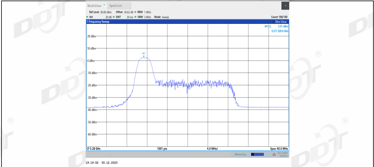
11AX20MIMO_Ant1_5280_26Tone_RU4
