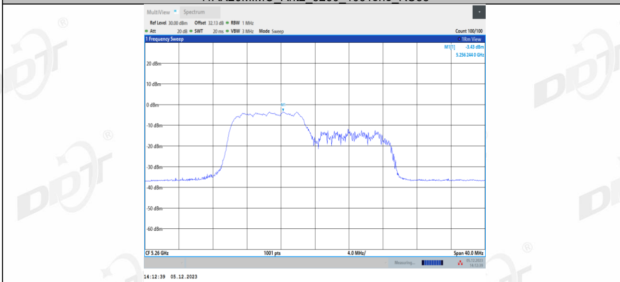
11AX20MIMO_Ant2_5260_106Tone_RU54
