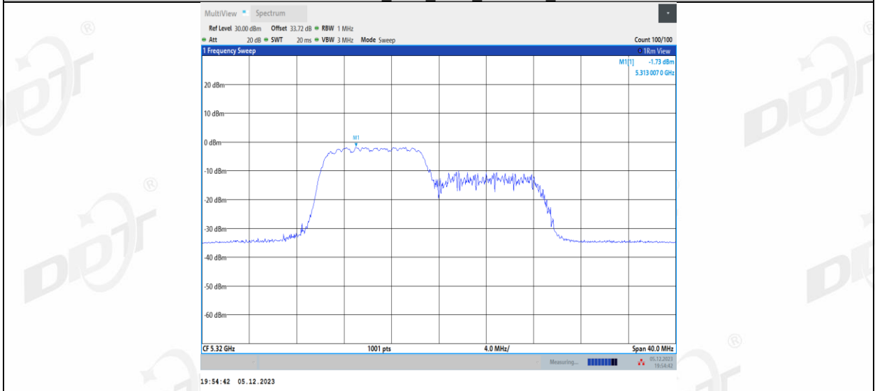
11AX20MIMO_Ant1_5320_106Tone_RU54
