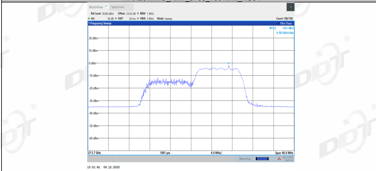
11AX20MIMO_Ant2_5700_26Tone_RU0
