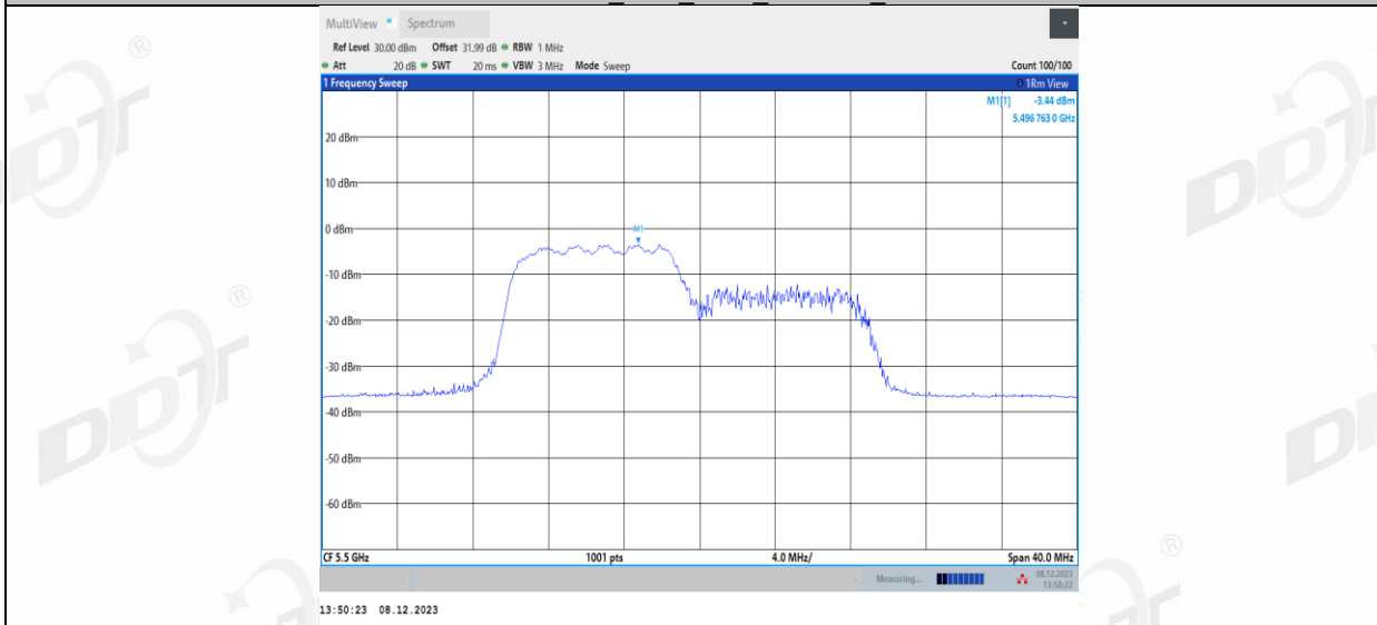
11AX20MIMO_Ant1_5500_106Tone_RU54
