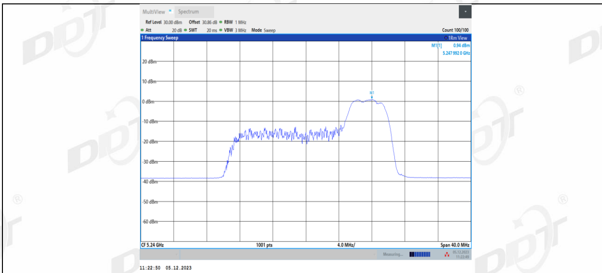
11AX20MIMO_Ant2_5240_106Tone_RU53
