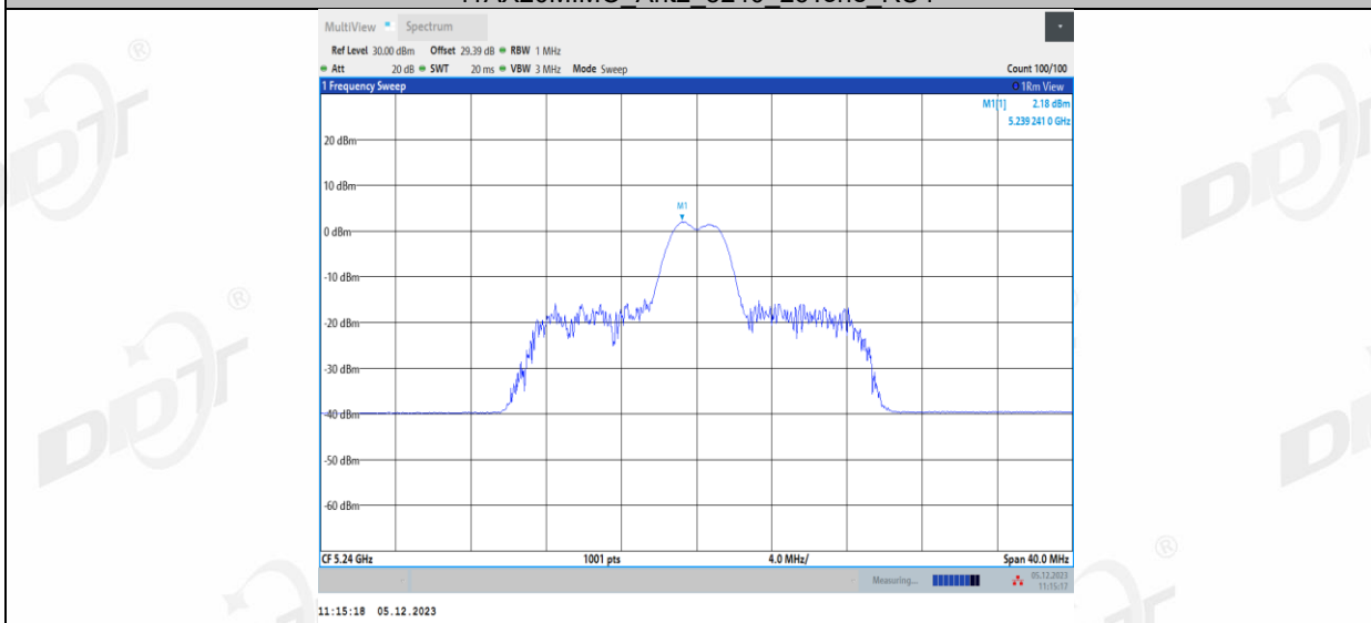
11AX20MIMO_Ant2_5240_26Tone_RU5
