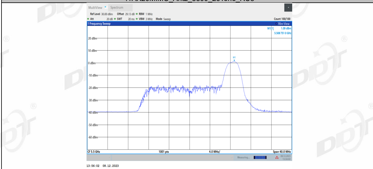
11AX20MIMO_Ant2_5500_52Tone_RU37
