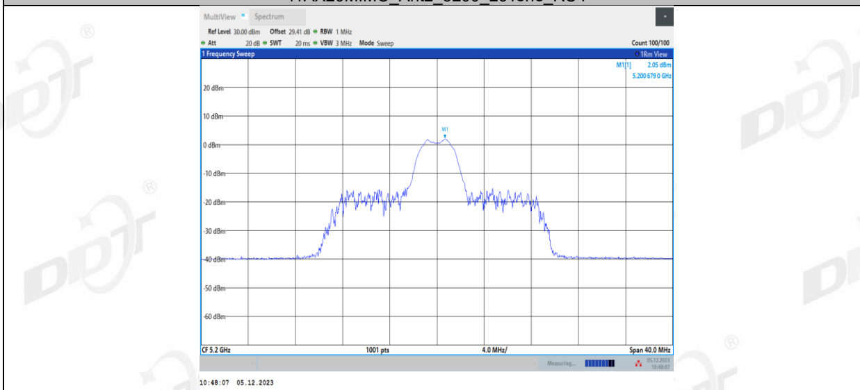
11AX20MIMO_Ant2_5200_26Tone_RU5
