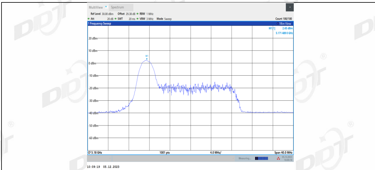
11AX20MIMO_Ant2_5180_26Tone_RU4
