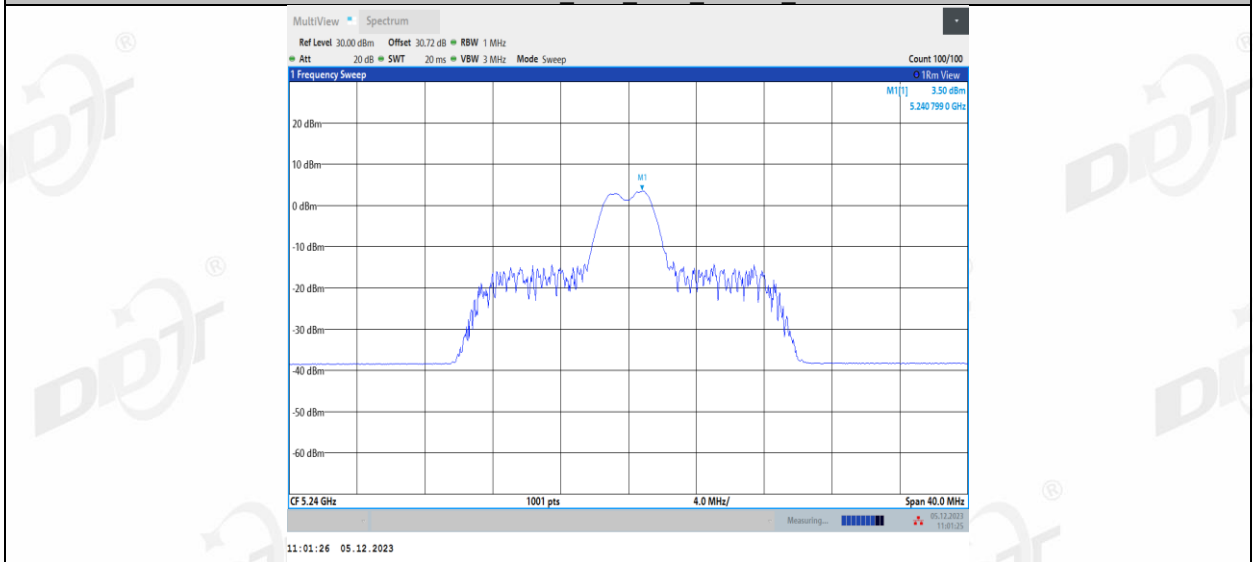
11AX20MIMO_Ant1_5240_26Tone_RU8
