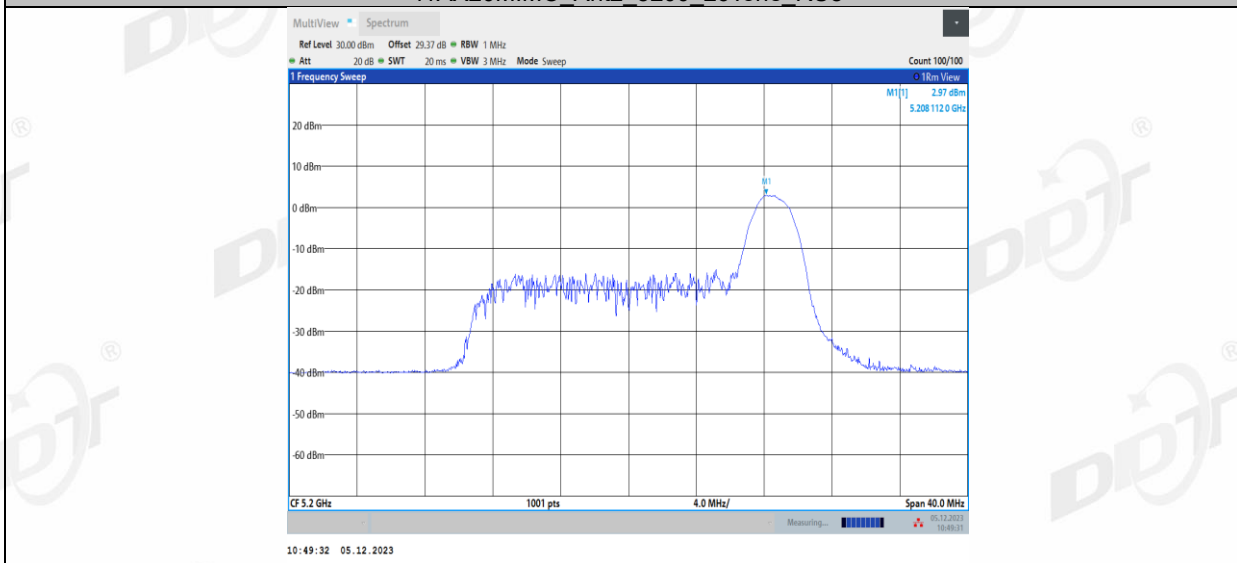
11AX20MIMO_Ant2_5200_52Tone_RU37
