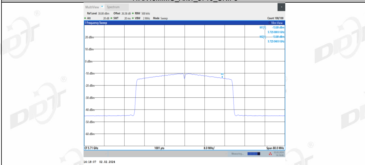
11AX40MIMO_Ant2_5710_UNII-3
