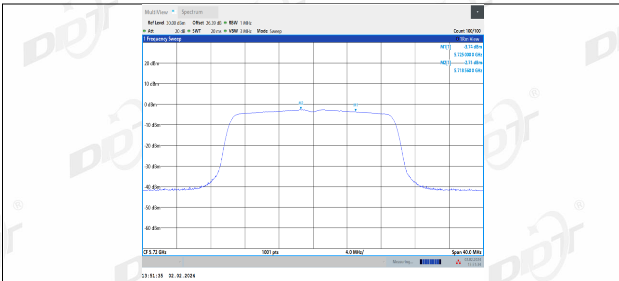
11AX20MIMO_Ant1_5720_UNII-3
