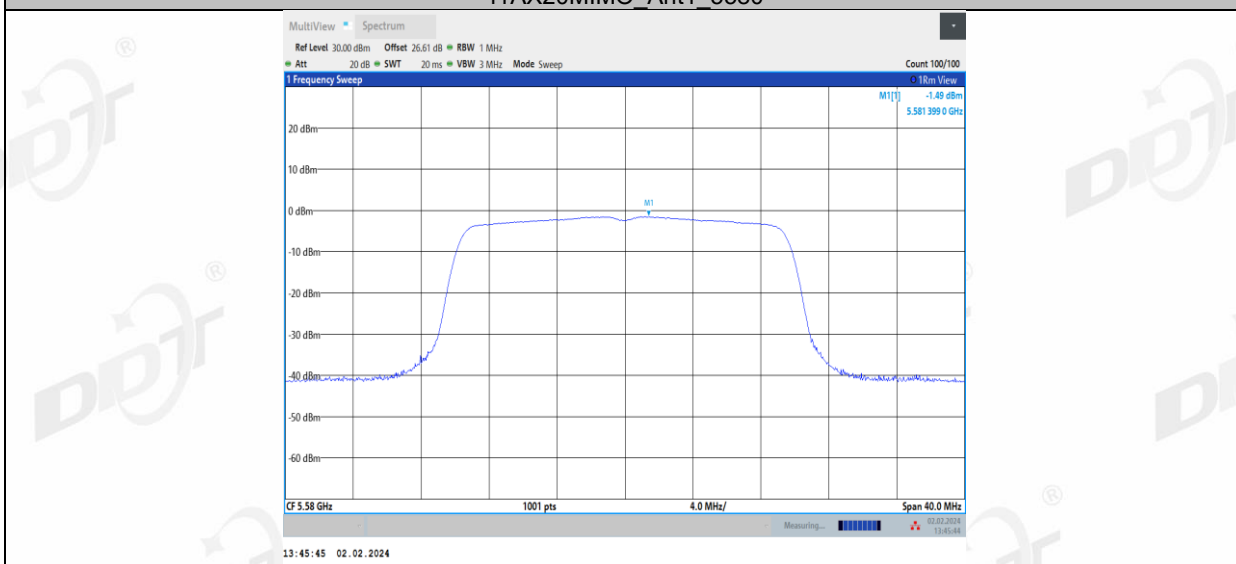
11AX20MIMO_Ant2_5580
