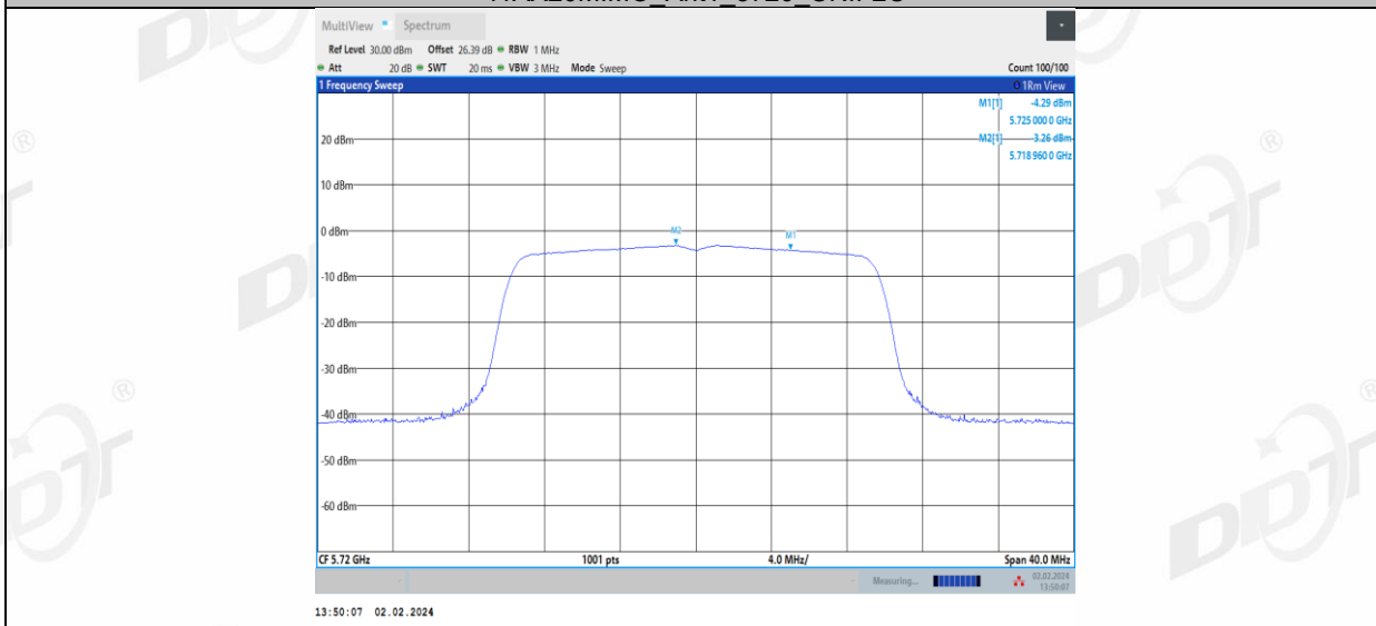
11AX20MIMO_Ant2_5720_UNII-2C
