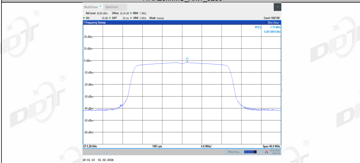
11AX20MIMO_Ant2_5280
