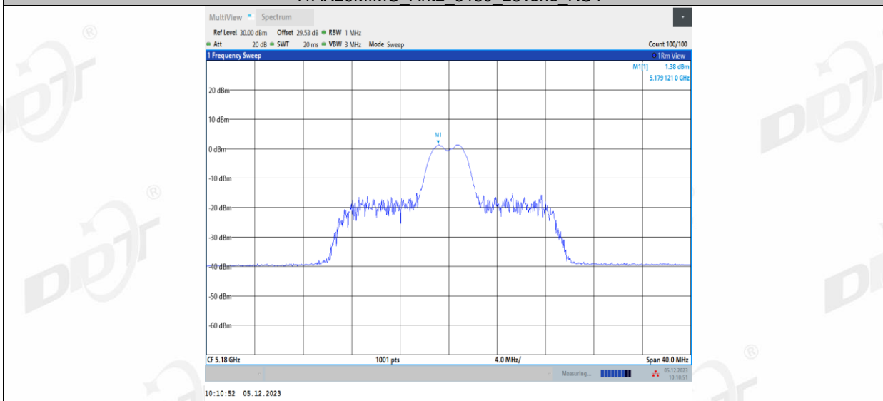
11AX20MIMO_Ant2_5180_26Tone_RU5
