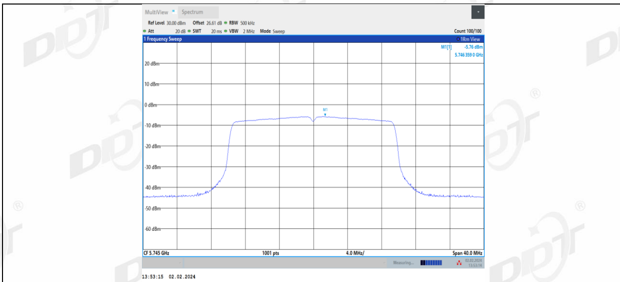
11AX20MIMO_Ant2_5745
