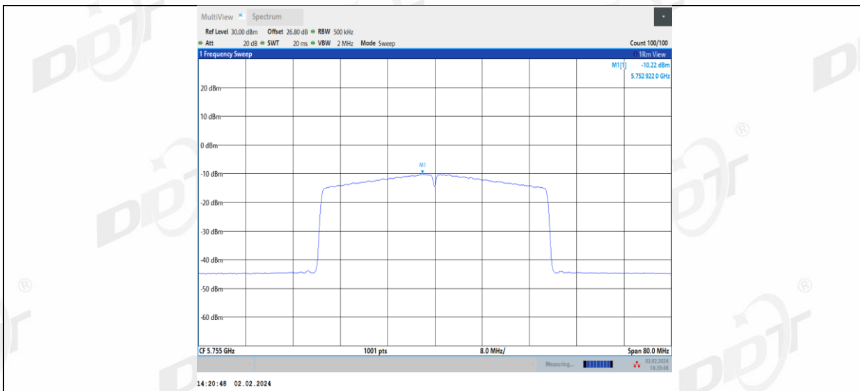
11AX40MIMO_Ant2_5755
