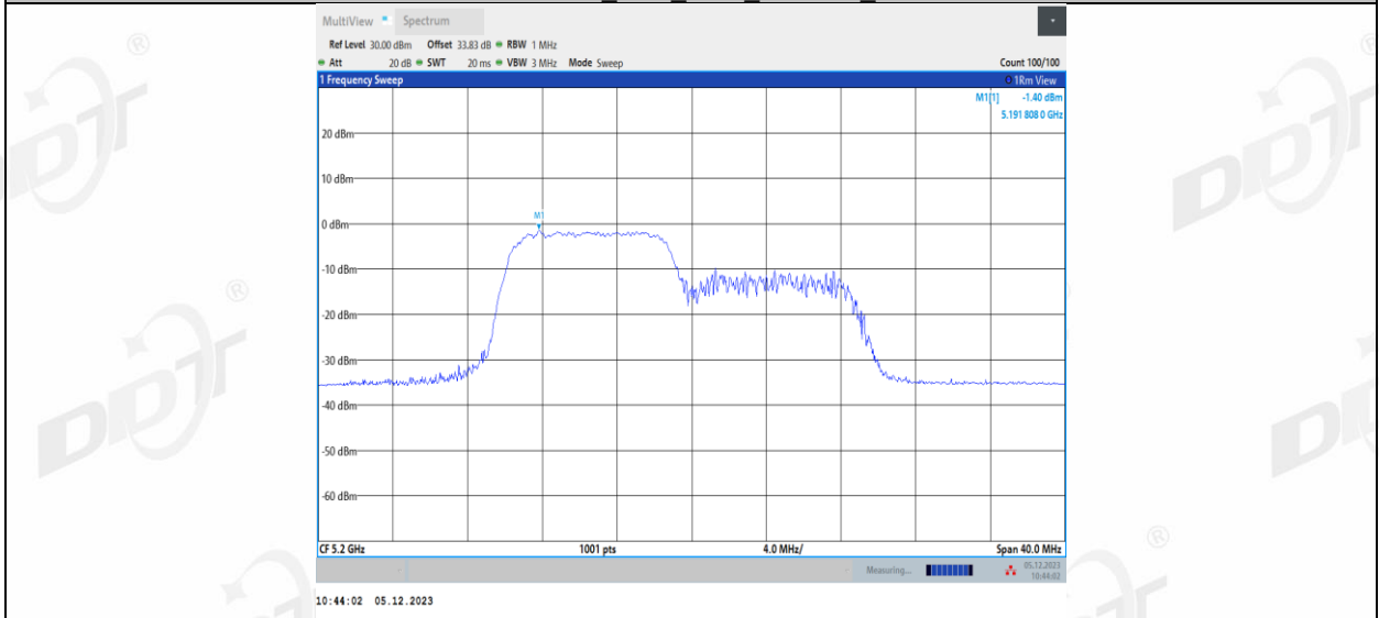
11AX20MIMO_Ant1_5200_106Tone_RU54
