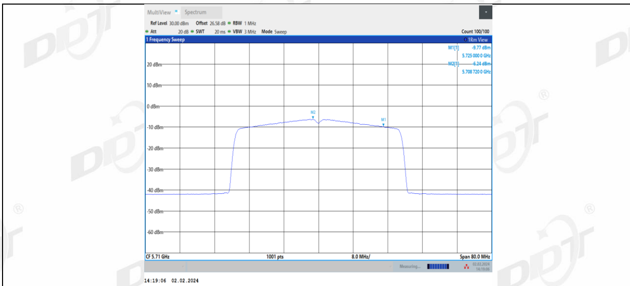
11AX40MIMO_Ant1_5710_UNII-3
