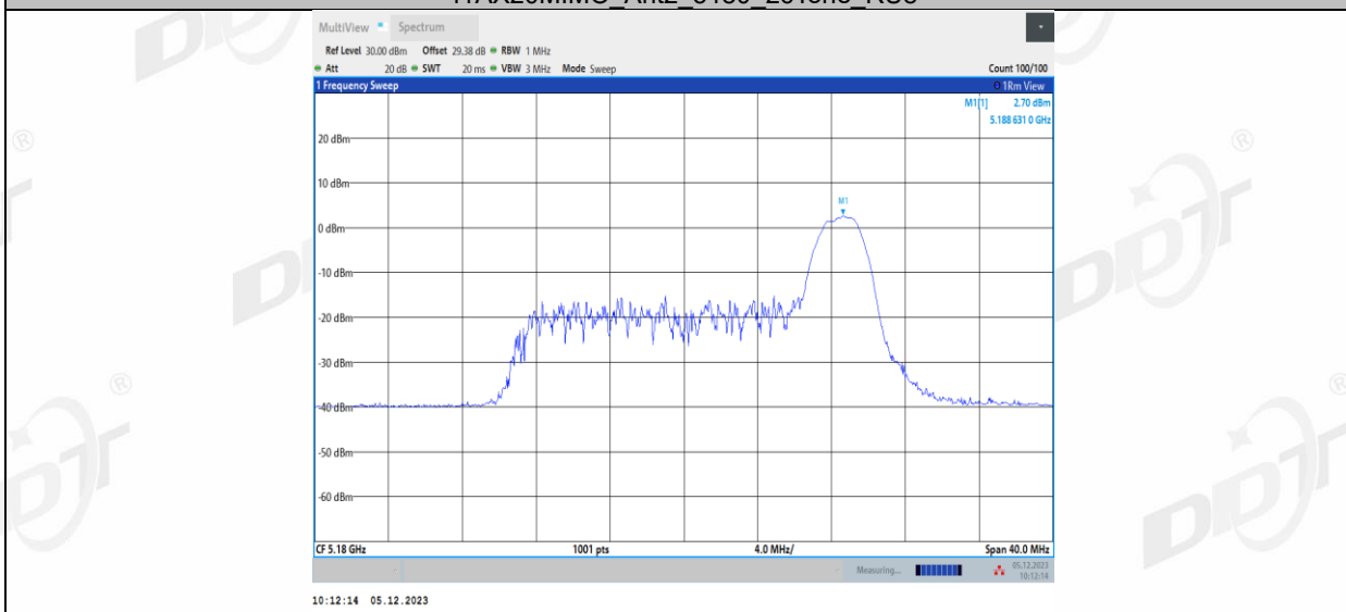
11AX20MIMO_Ant2_5180_52Tone_RU37
