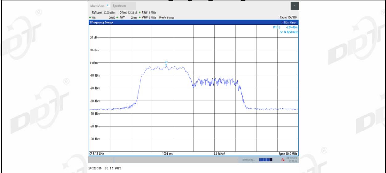
11AX20MIMO_Ant2_5180_106Tone_RU54
