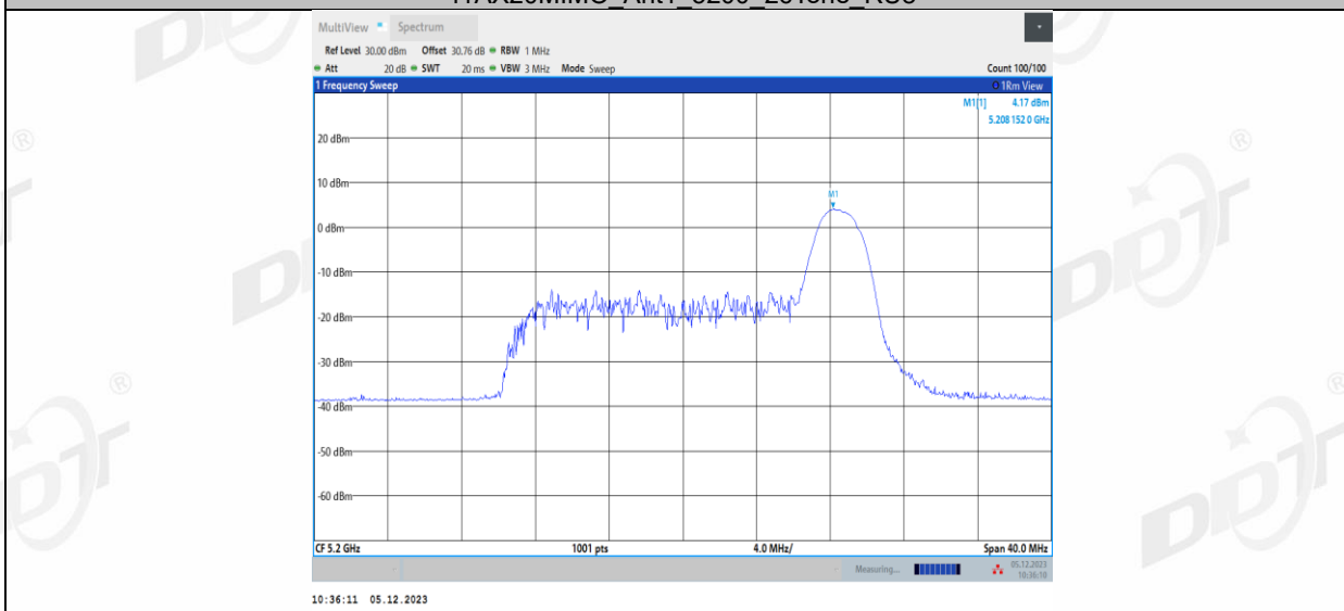
11AX20MIMO_Ant1_5200_52Tone_RU37
