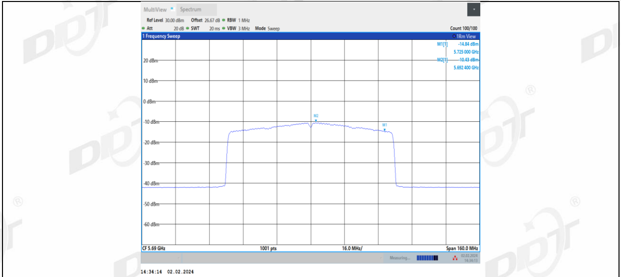
11AX80MIMO_Ant2_5690_UNII-2C
