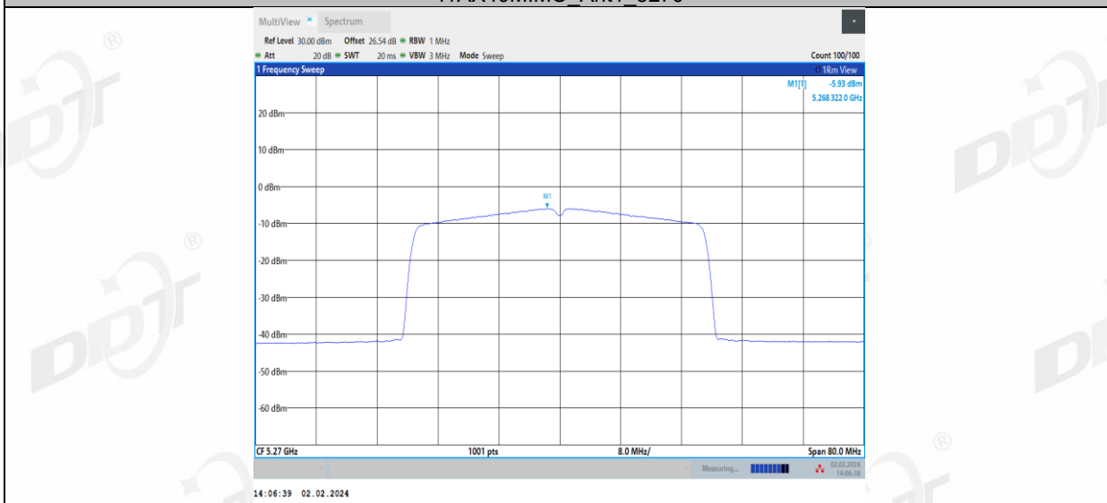
11AX40MIMO_Ant2_5270
