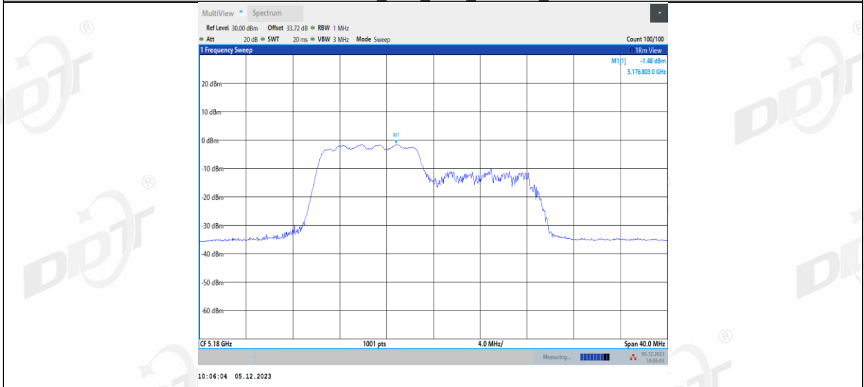
11AX20MIMO_Ant1_5180_106Tone_RU54
