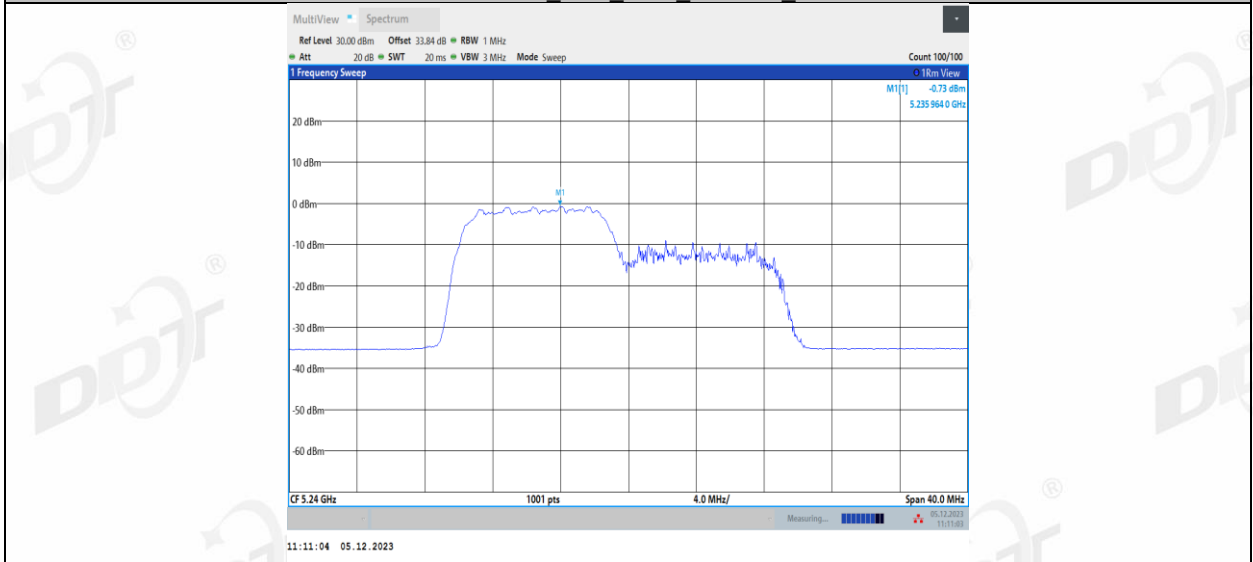
11AX20MIMO_Ant1_5240_106Tone_RU54
