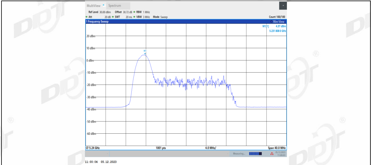
11AX20MIMO_Ant1_5240_26Tone_RU4
