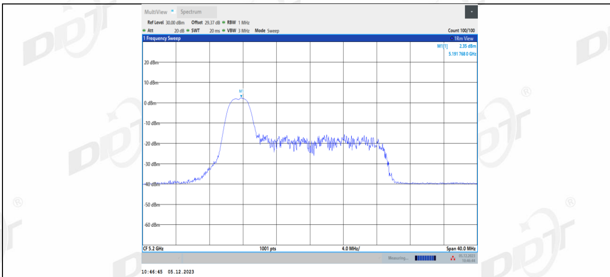
11AX20MIMO_Ant2_5200_26Tone_RU4
