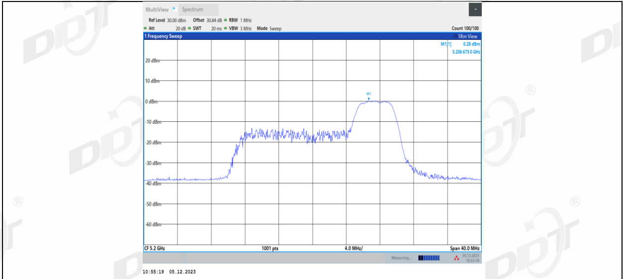
11AX20MIMO_Ant2_5200_106Tone_RU53
