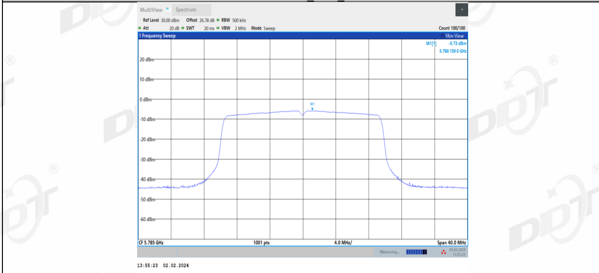
11AX20MIMO_Ant2_5785
