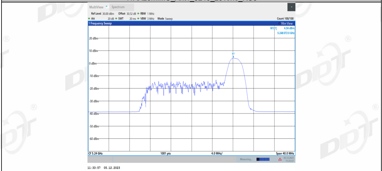
11AX20MIMO_Ant1_5240_52Tone_RU37
