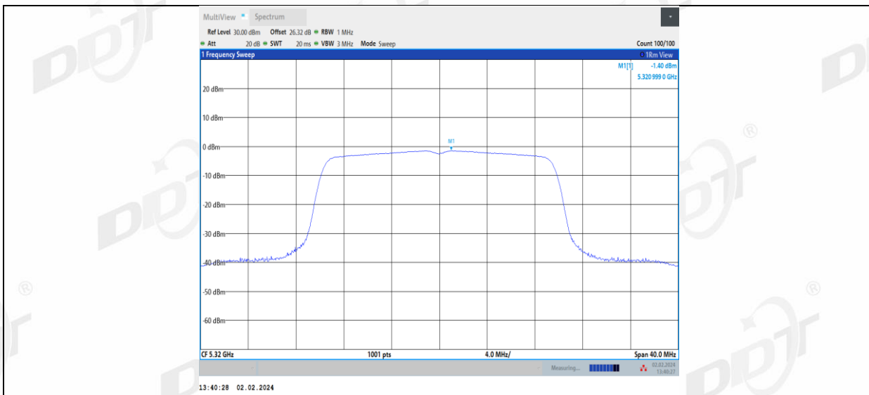
11AX20MIMO_Ant2_5320
