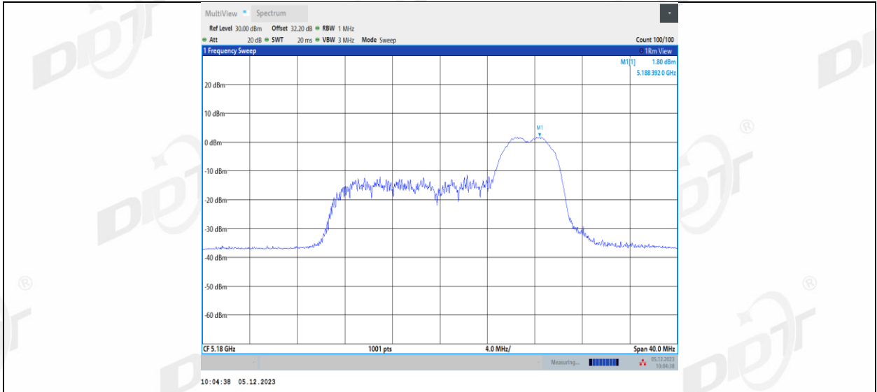
11AX20MIMO_Ant1_5180_106Tone_RU53
