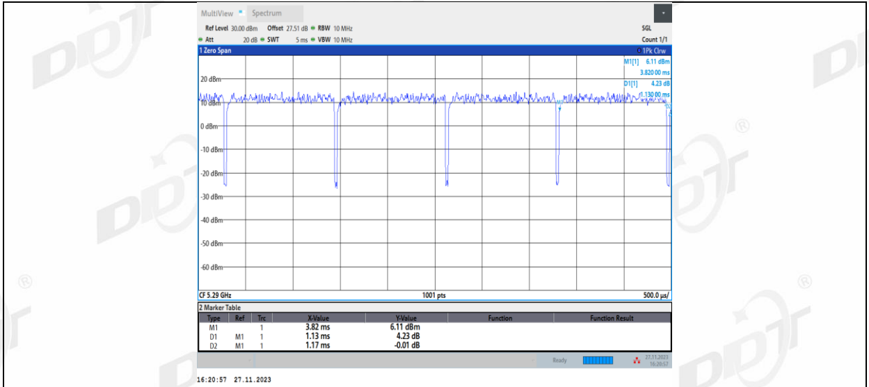
11AC80MIMO_Ant2_5290
