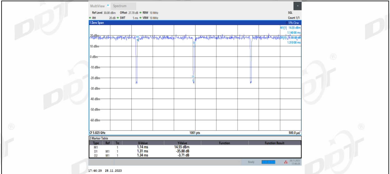
11AC20MIMO_Ant2_5825
