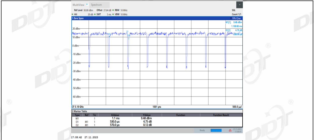
11AX40MIMO_Ant2_5190
