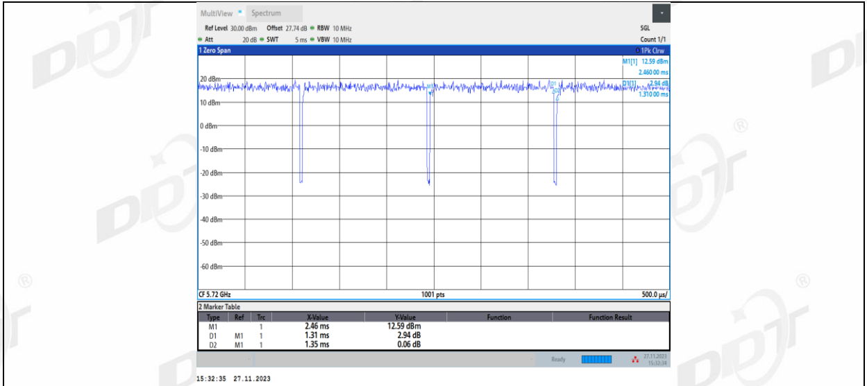
11AC20MIMO_Ant2_5720
