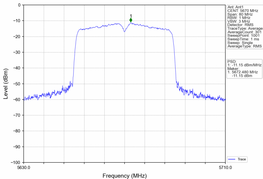
802.11ax(HEW40)_HCH_5670MHz_RU484_Left_Ant1_NTNV
