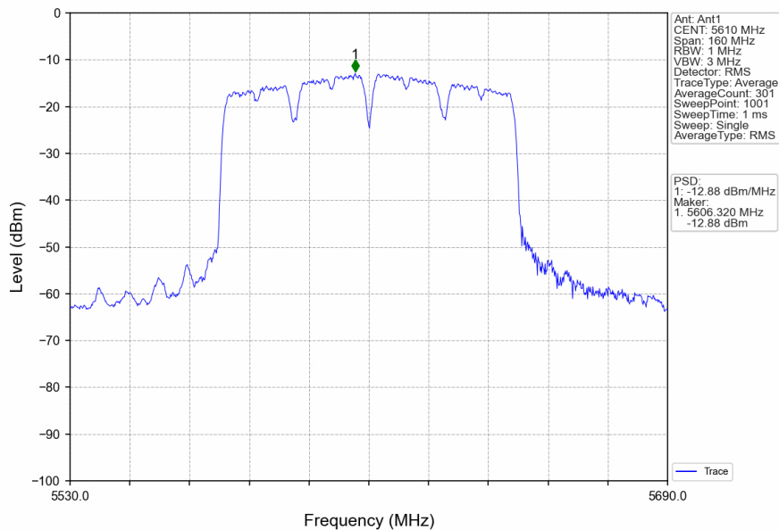
802.11ax(HEW80)_HCH_5610MHz_RU996_Left_Ant1_NTNV
