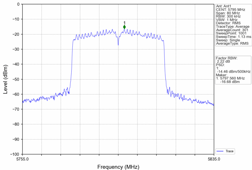
802.11ax(HEW40)_HCH_5795MHz_RU484_Left_Ant1_NTNV
