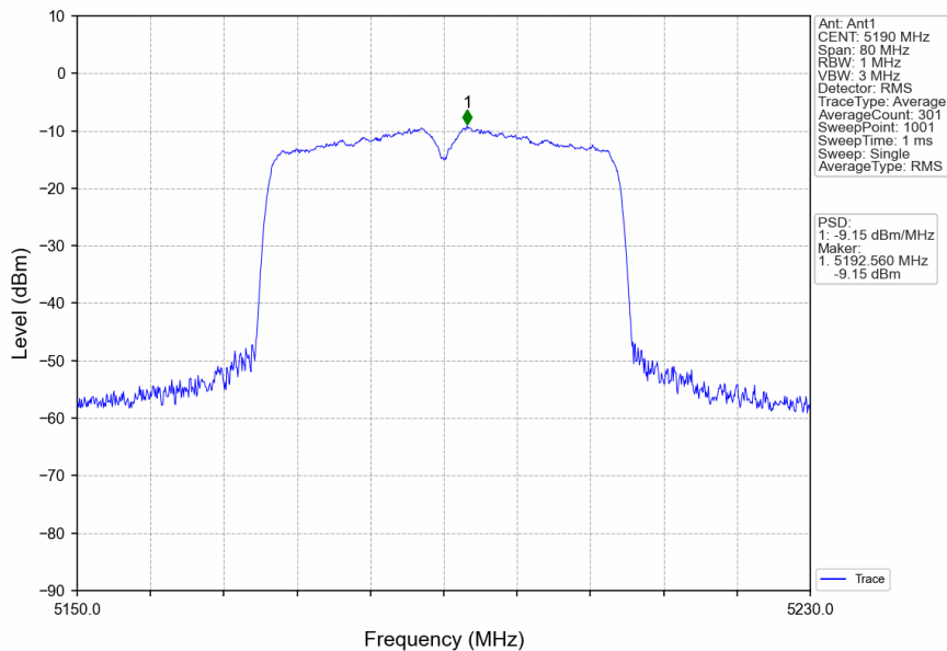
802.11ax(HEW40)_LCH_5190MHz_RU484_Left_Ant1_NTNV
