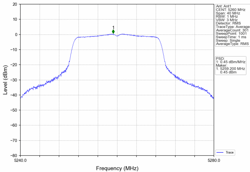
802.11n(HT20)_LCH_5260MHz_Ant1_NTNV
