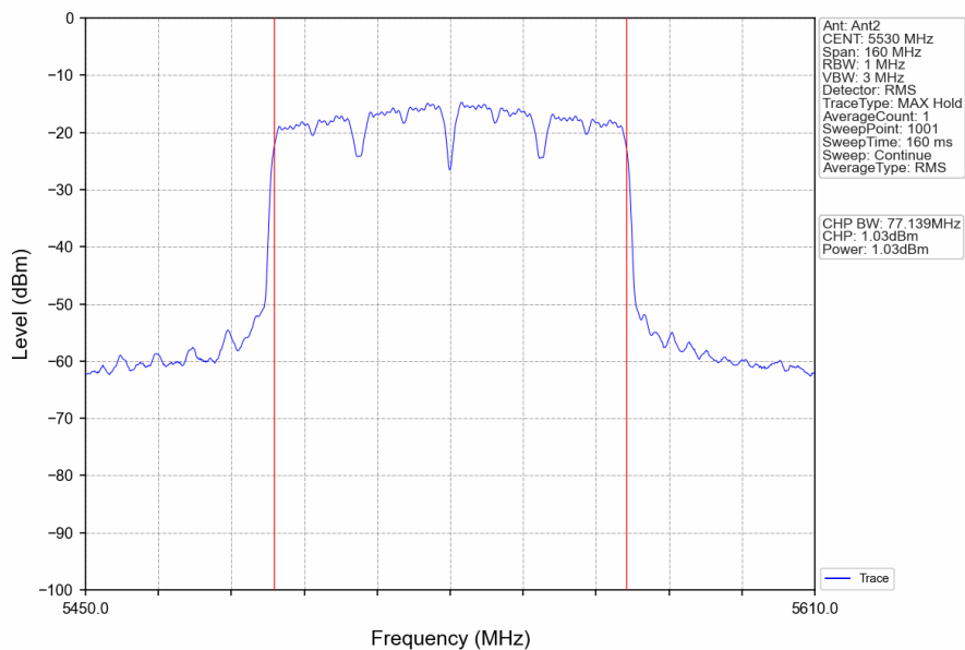
802.11ax(HEW80)_LCH_5530MHz_RU996_Left_Ant2_NTNV
