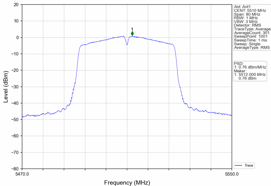
802.11n(HT40)_LCH_5510MHz_Ant1_NTNV
