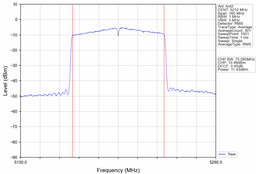
802.11ac(VHT80)_MCH_5210MHz_Ant2_NTNV
