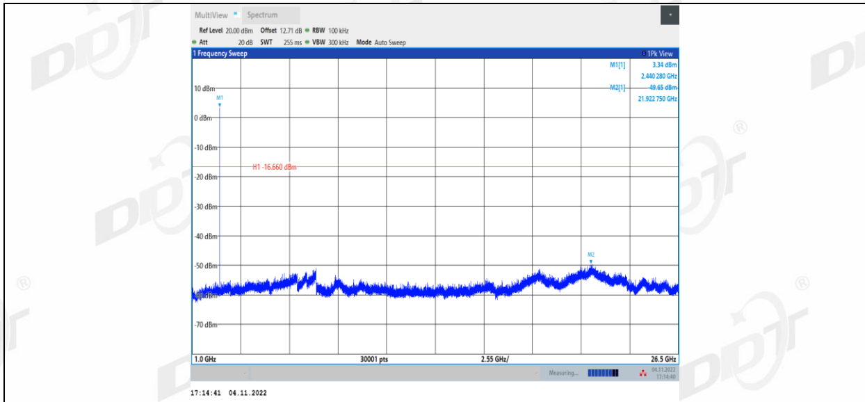
BLE 2M_Ant1_2480_0~Reference
