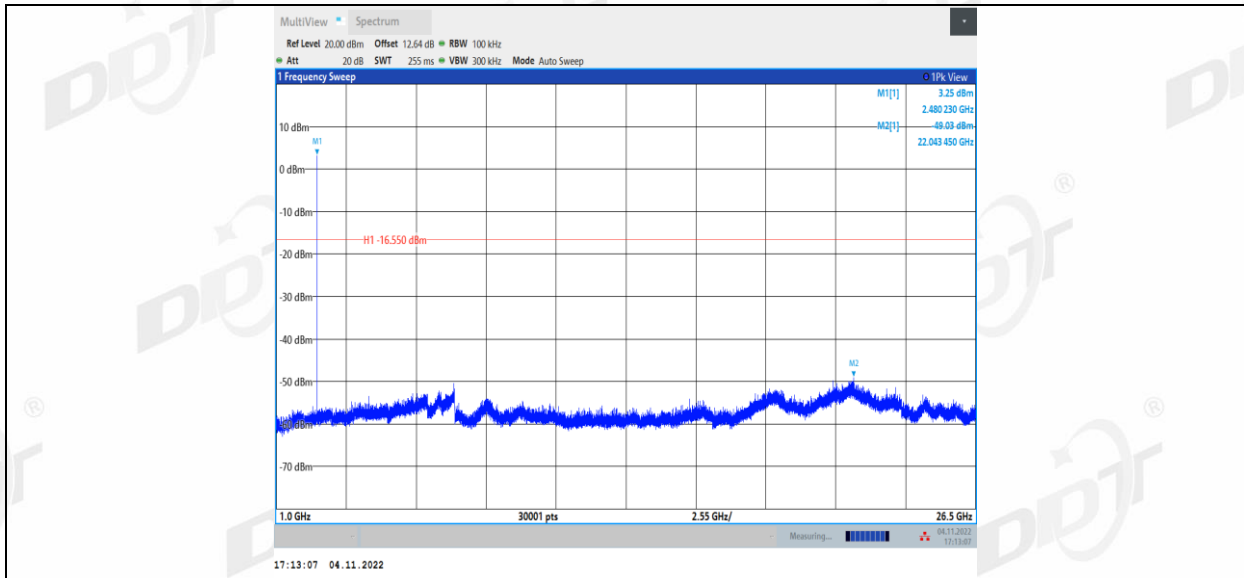
BLE 2M_Ant1_2402_0~Reference
